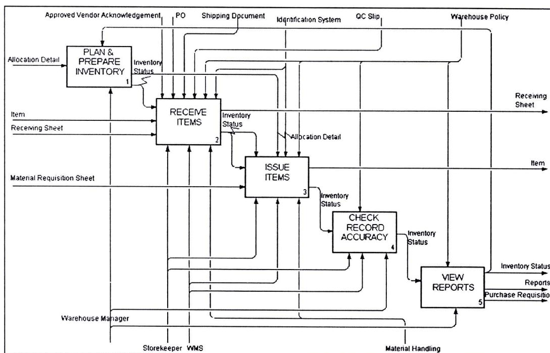
รูปที่ 3.3) แสดง IDEF0 ของกระบวนการงานจัดการคลังระดับ A0
