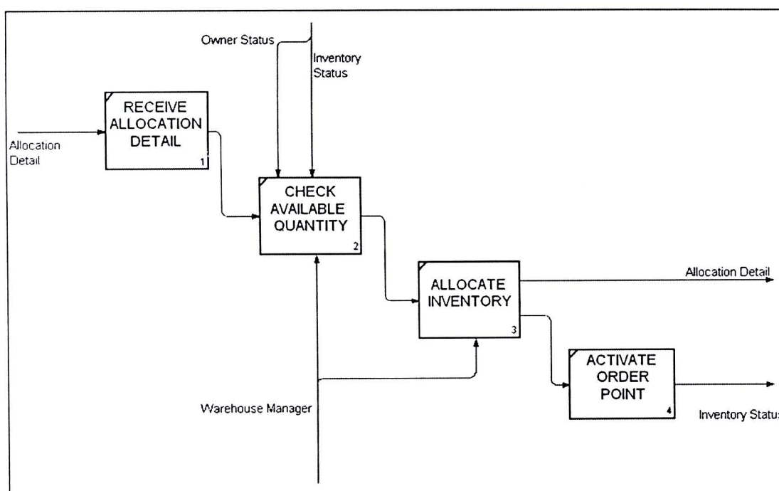
รูปที่ 3.5) แสดง IDEF0 ของกระบวนการจัดการคลังระดับ A1
