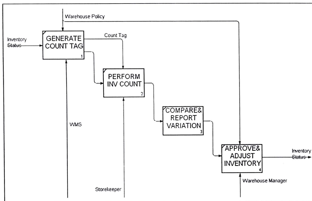
รูปที่ 3.11) แสดง IDEFO ของกระบวนการจัดการคลังระดับ A4
