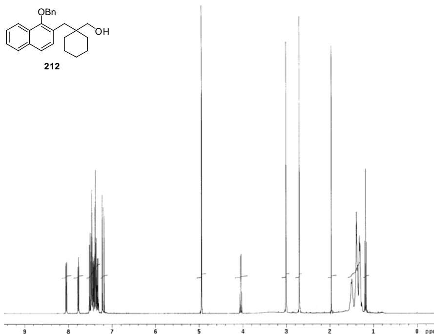
Appendix Figure 87 400 MHz 1 H NMR spectrum of (1-((1-(benzyloxy)naphthalen-2-yl)methyl)cyclohexyl)methanol ( 212 )
