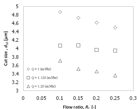
รูปที่ 5 ขนาดตัดที่อัตราส่วนการไหลและอัตราการไหลต่างๆ
