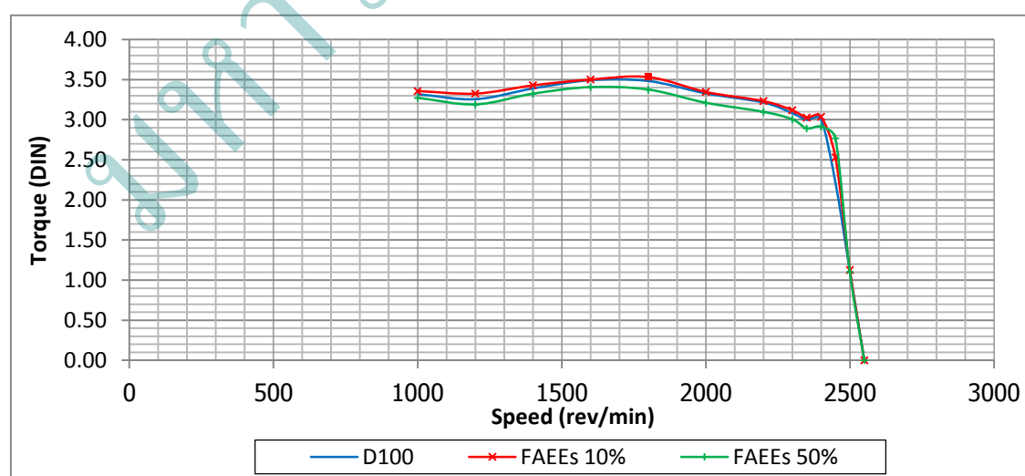
รูปที่ 4 ค่าแรงบิดของเครื่องยนต์
