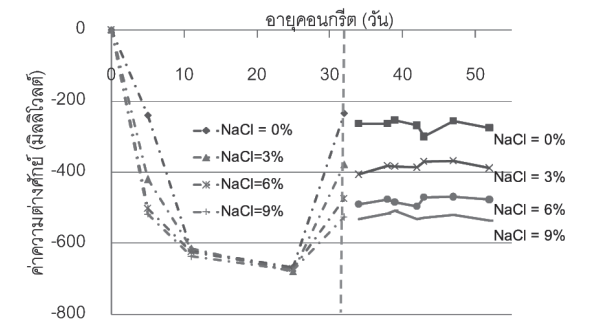
รูปที่ 4 ผลของปริมาณคลอไรด์ต่อค่าศักย์ไฟฟ้าครึ่งเซลล์
