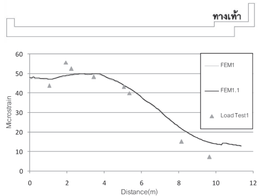
(ก) ค่าความเครียดของสะพานกรณีวางน้ำหนักบรรทุกชิดขอบคันตก
