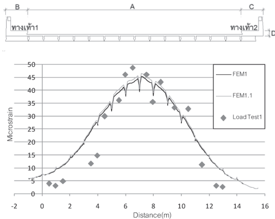
(ก) ค่าความเครียดของสะพานกรณีวางน้ำหนักบรรทุก กึ่งกลางสะพาน
