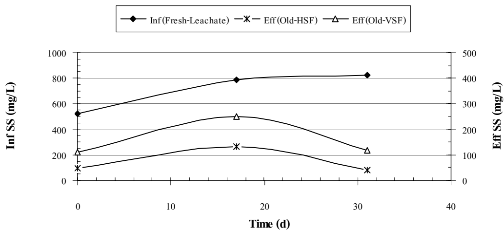
ภาพผนวกที่ ข61 SS ของ Fresh Leachate ระบบ HSF และ VSF Run 3
