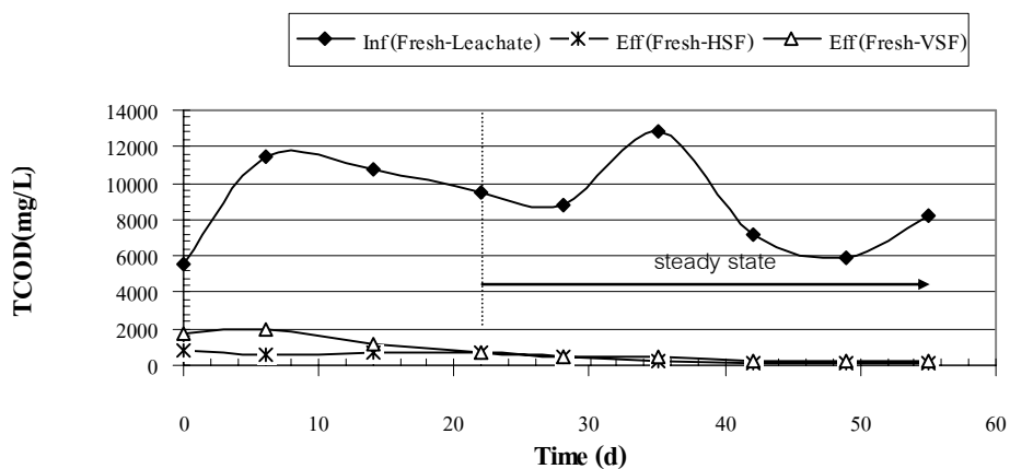
ภาพผนวกที่ ข27 TCOD ของ Fresh Leachate ระบบ HSF และ VSF Run 2
