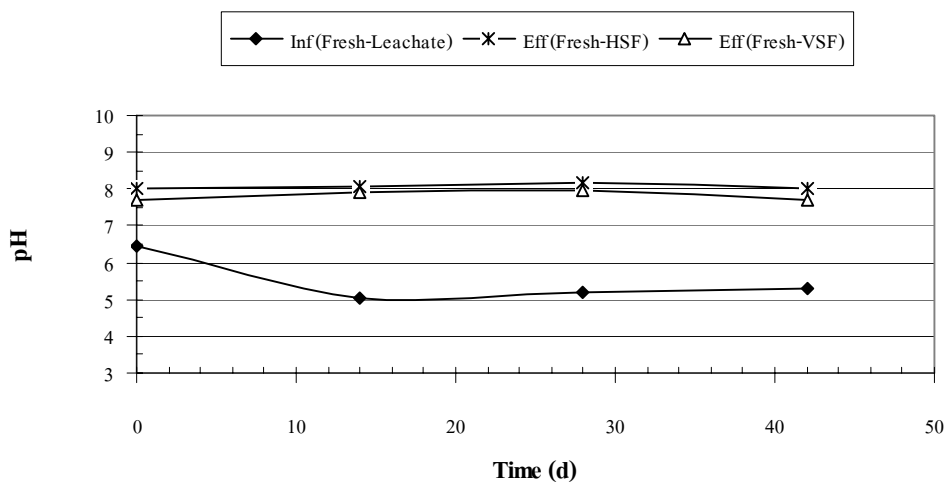
ภาพผนวกที่ ข38 pH ของ Fresh Leachate ระบบ HSF และ VSF Run 2
