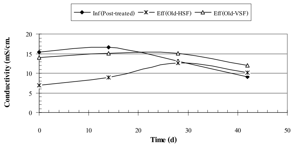
ภาพผนวกที่ ข52 EC ของ Old Leachate ระบบ HSF และ VSF Run 2
