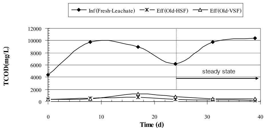
ภาพผนวกที่ ข53 TCOD ของ Fresh Leachate ระบบ HSF และ VSF Run 3
