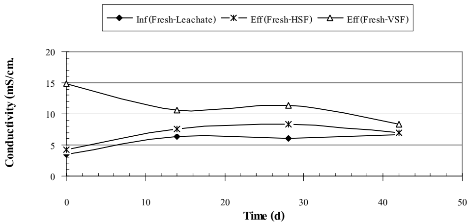
ภาพผนวกที่ ข39 EC ของ Fresh Leachate ระบบ HSF และ VSF Run 2
