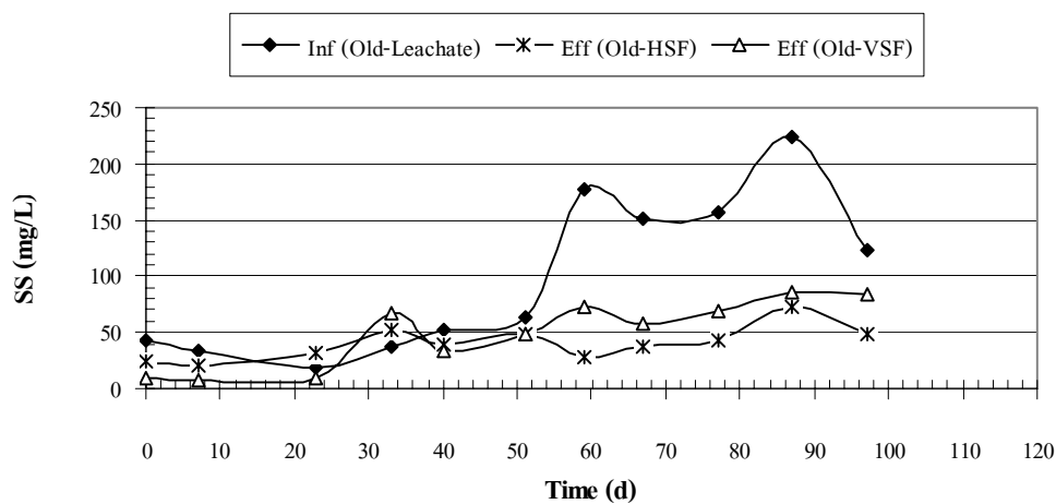
ภาพผนวกที่ ข22 SS ของ Old Leachate ระบบ HSF และ VSF Run 1
