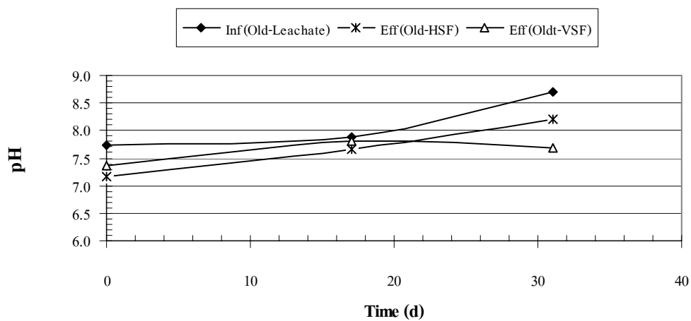
ภาพผนวกที่ ข77 pH ของ Old Leachate ระบบ HSF และ VSF Run 3
