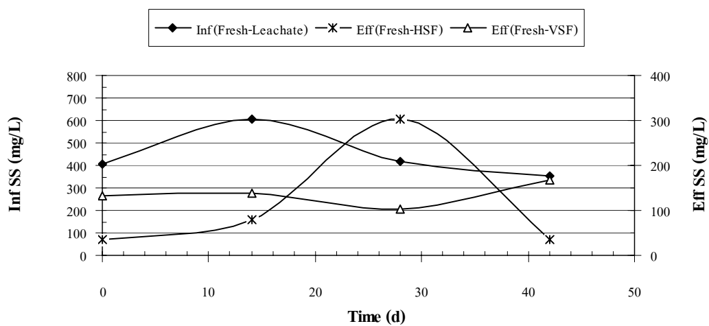
ภาพผนวกที่ ข35 SS ของ Fresh Leachate ระบบ HSF และ VSF Run 2
