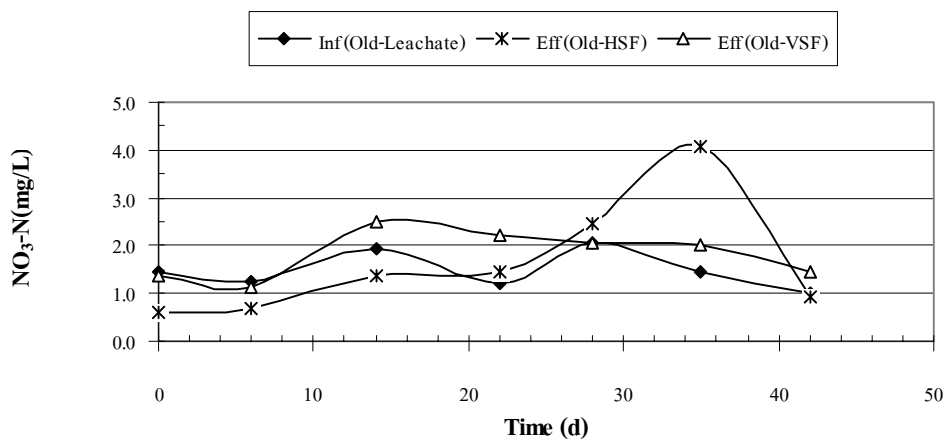
ภาพผนวกที่ ๔๖ NO 3 -N ของ Old Leachate ระบบ HSF และ VSF Run 2
