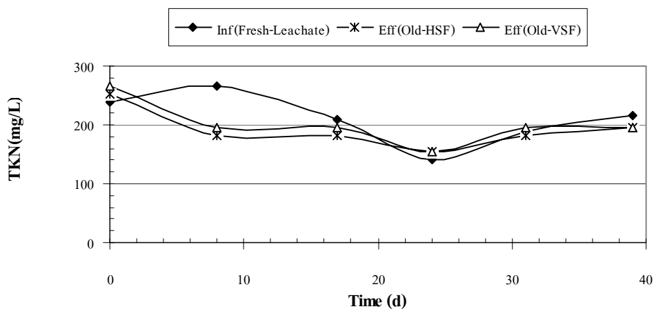
ภาพผนวกที่ ๕๖ TKN ของ Fresh Leachate ระบบ HSF และ VSF Run 3
