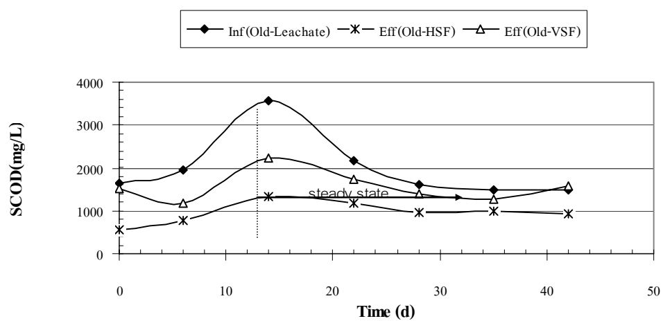
ภาพผนวกที่ ๒41 SCOD ของ Old Leachate ระบบ HSF และ VSF Run 2
