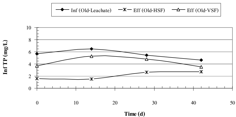
ภาพผนวกที่ ๔๗ TP ของ Old Leachate ระบบ HSF และ VSF Run 2
