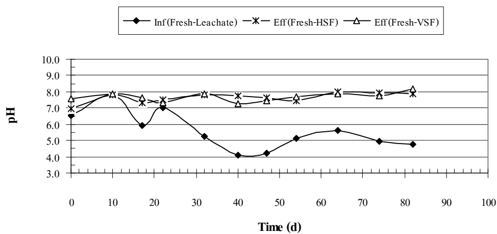
ภาพผนวกที่ ข12 pH ของ Fresh Leachate ระบบ HSF และ VSF Run 1
