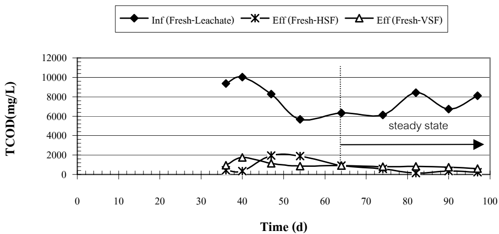
ภาพผนวกที่ ข1 TCOD ของ Fresh Leachate ระบบ HSF และ VSF Run 1
