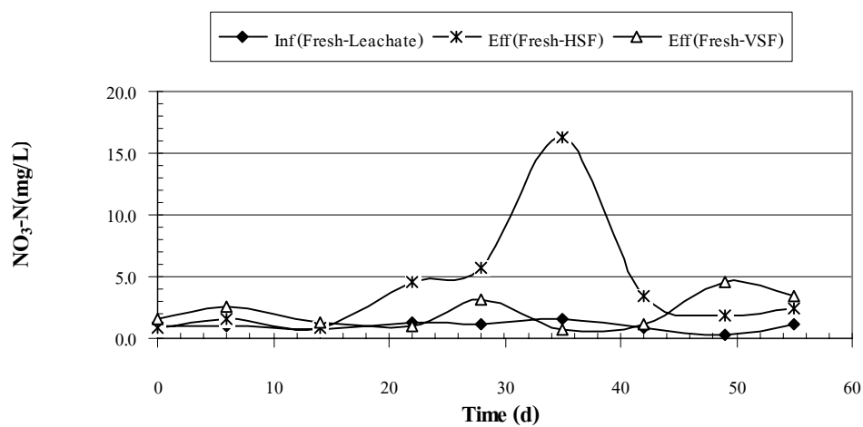
ภาพผนวกที่ ข33 \text{NO}_3\text{-N} ของ Fresh Leachate ระบบ HSF และ VSF Run 2
