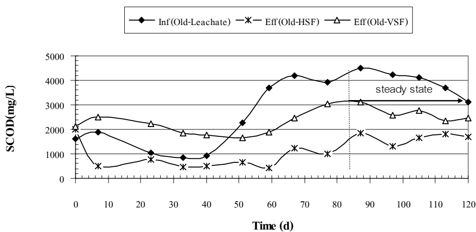
ภาพผนวกที่ ข15 SCOD ของ Old Leachate ระบบ HSF และ VSF Run 1
