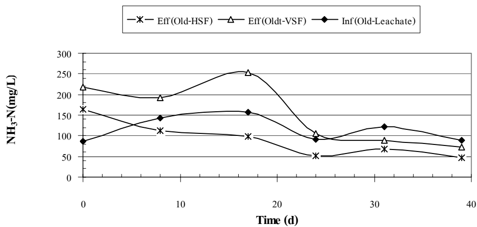
ภาพผนวกที่ ข70 NH 3 -N ของ Old Leachate ระบบ HSF และ VSF Run 3
