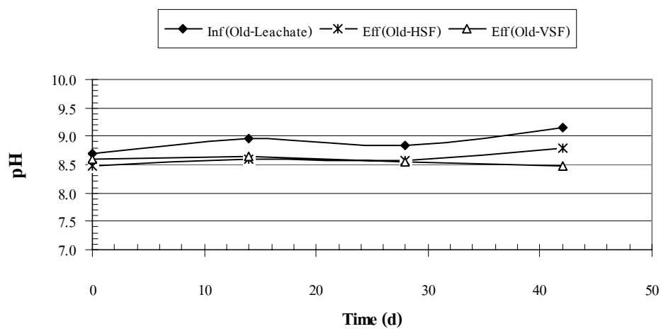
ภาพผนวกที่ ๕๑ pH ของ Old Leachate ระบบ HSF และ VSF Run 2
