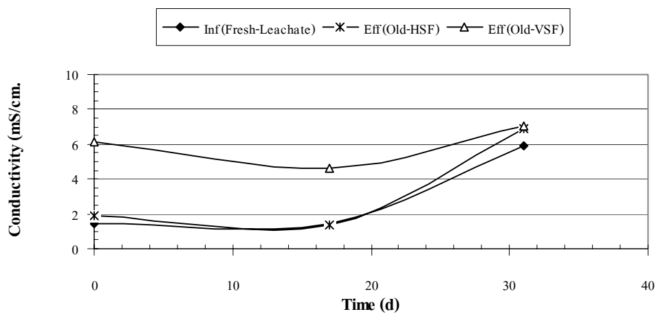
ภาพผนวกที่ ข65 EC ของ Fresh Leachate ระบบ HSF และ VSF Run 3
