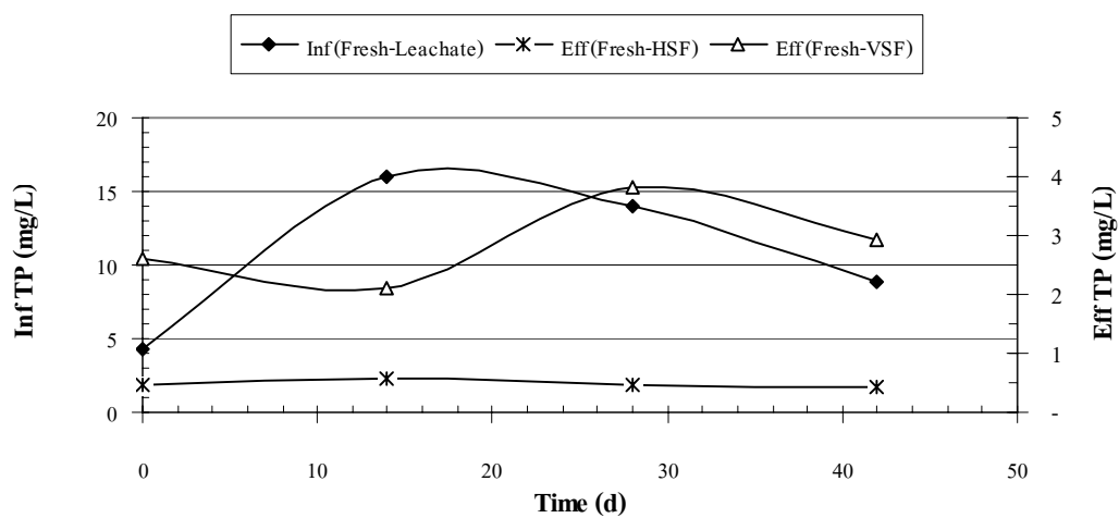
ภาพผนวกที่ ข34 TP ของ Fresh Leachate ระบบ HSF และ VSF Run 2
