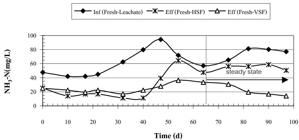
ภาพผนวกที่ ๕ \text{NH}_3\text{-N} ของ Fresh Leachate ระบบ HSF และ VSF Run 1
