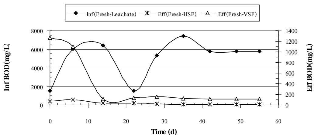
ภาพผนวกที่ ๒๒๙ SBOD ของ Fresh Leachate ระบบ HSF และ VSF Run 2
