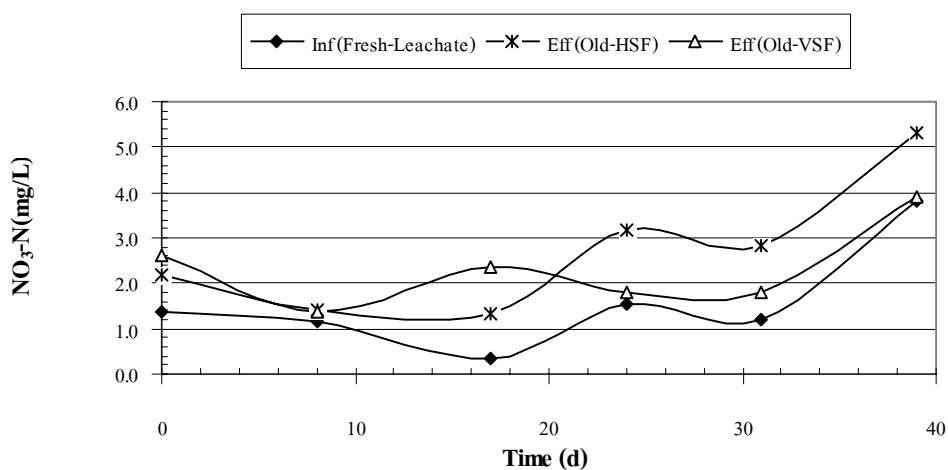
ภาพผนวกที่ ข59 NO 3 -N ของ Fresh Leachate ระบบ HSF และ VSF Run 3
