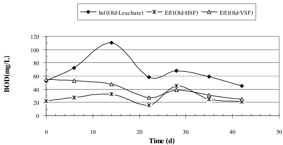
ภาพผนวกที่ ๒42 SBOD ของ Old Leachate ระบบ HSF และ VSF Run 2
