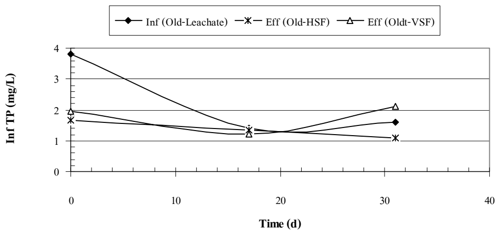
ภาพผนวกที่ ข73 TP ของ Old Leachate ระบบ HSF และ VSF Run 3
