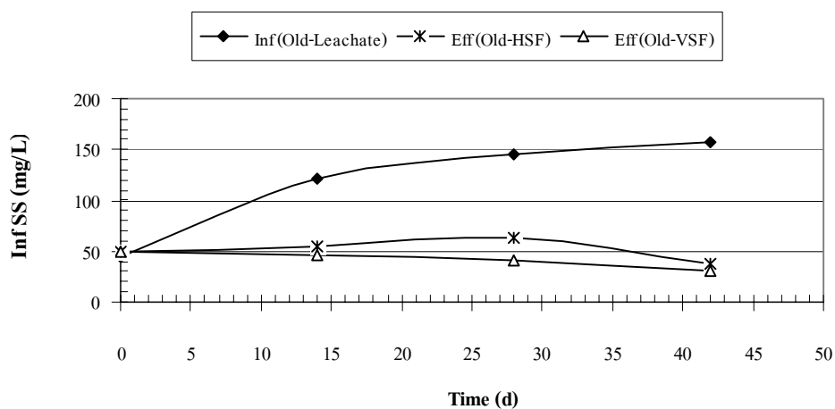
ภาพผนวกที่ ๔๘ SS ของ Old Leachate ระบบ HSF และ VSF Run 2
