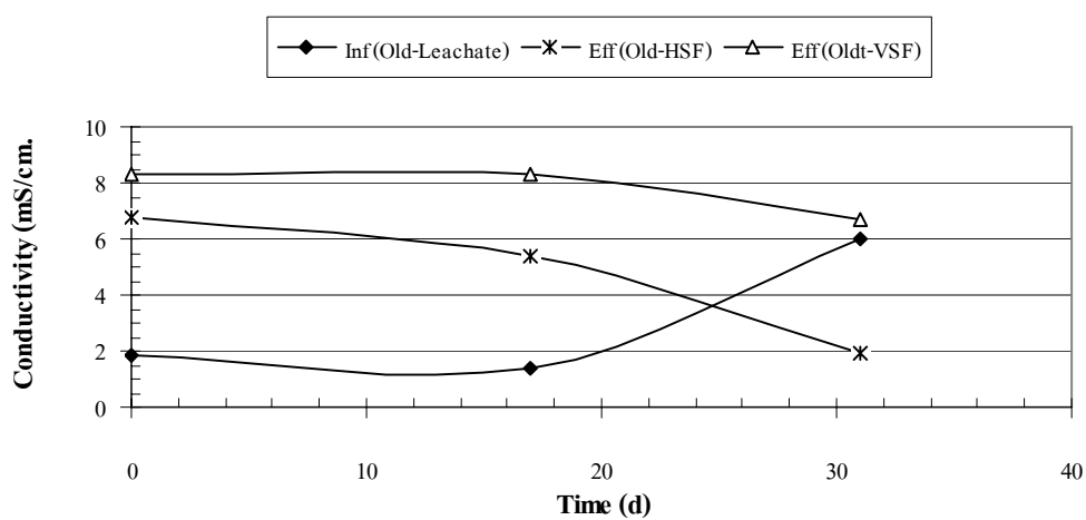
ภาพผนวกที่ ข78 EC ของ Old Leachate ระบบ HSF และ VSF Run 3
