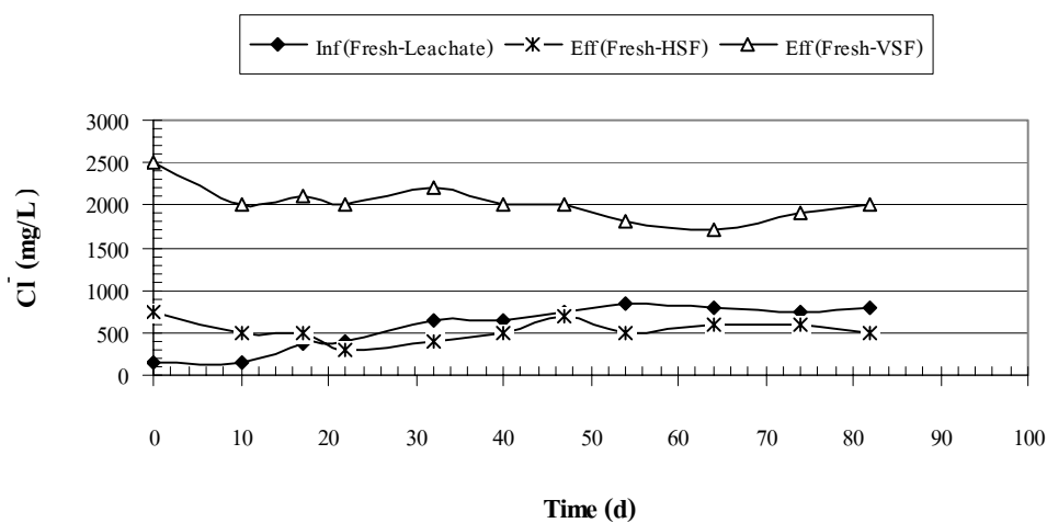
ภาพผนวกที่ ข11 Cl- ของ Fresh Leachate ระบบ HSF และ VSF Run 1
