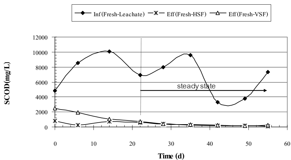
ภาพผนวกที่ ๒๒๘ SCOD ของ Fresh Leachate ระบบ HSF และ VSF Run 2
