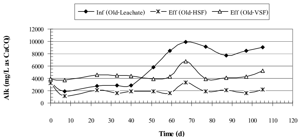
ภาพผนวกที่ ข23 Alk ของ Old Leachate ระบบ HSF และ VSF Run 1
