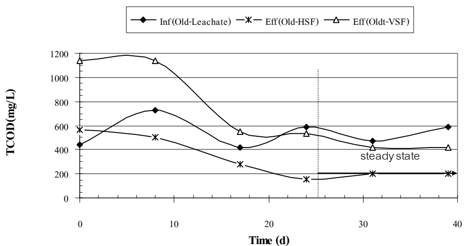
ภาพผนวกที่ ข66 TCOD ของ Old Leachate ระบบ HSF และ VSF Run 3
