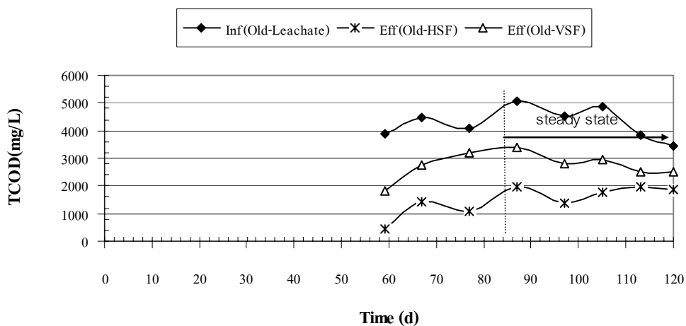
ภาพผนวกที่ ข14 TCOD ของ Old Leachate ระบบ HSF และ VSF Run 1
