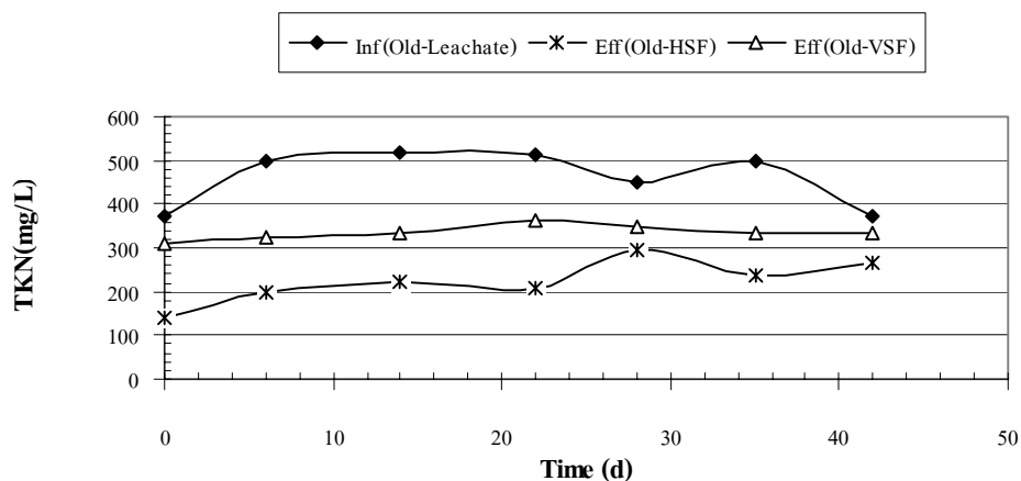
ภาพผนวกที่ ข43 TKN ของ Old Leachate ระบบ HSF และ VSF Run 2
