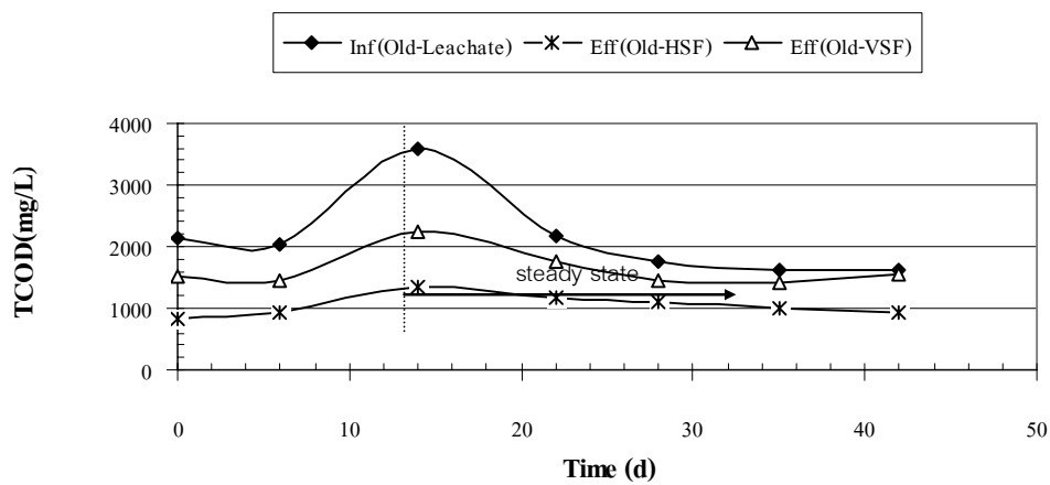
ภาพผนวกที่ ๒40 TCOD ของ Old Leachate ระบบ HSF และ VSF Run 2
