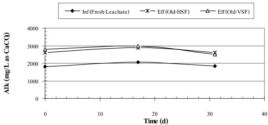
ภาพผนวกที่ ข62 Alk ของ Fresh Leachate ระบบ HSF และ VSF Run 3
