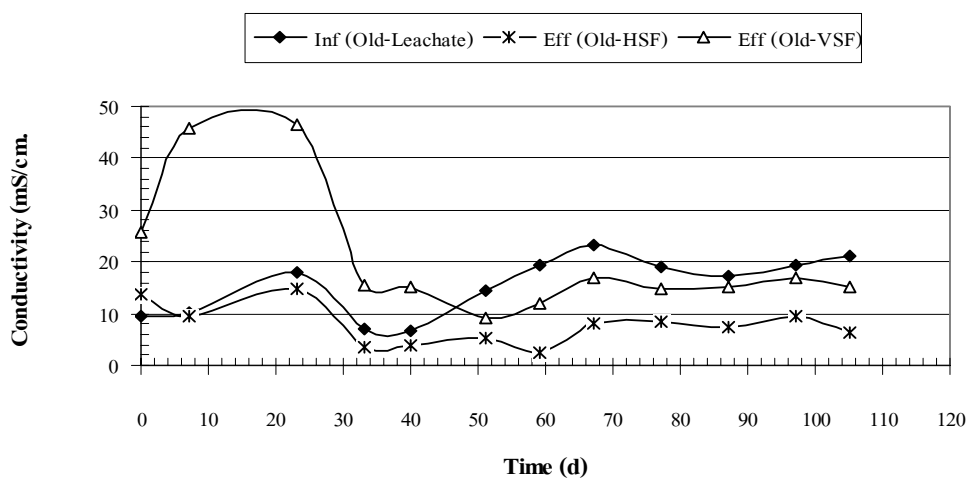
ภาพผนวกที่ ข26 EC ของ Old Leachate ระบบ HSF และ VSF Run 1
