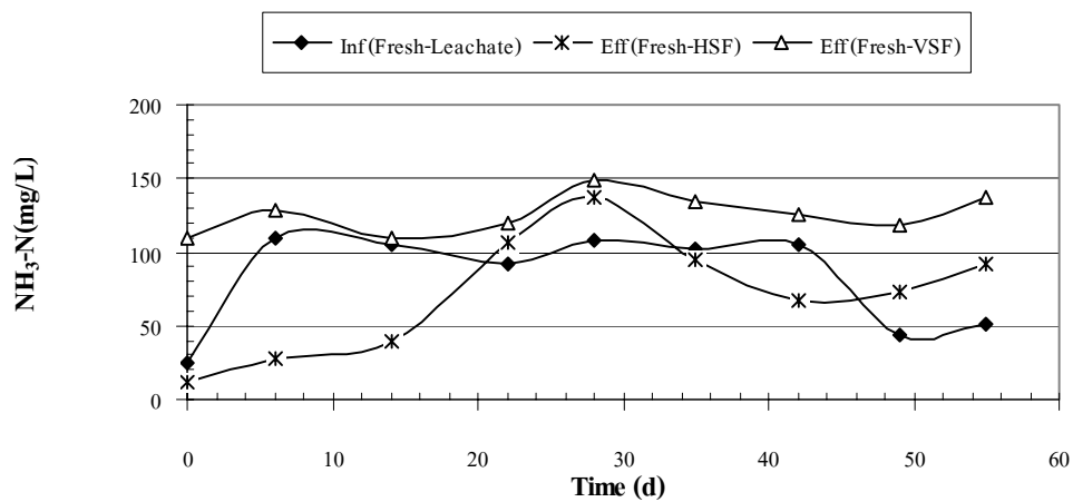
ภาพผนวกที่ ข31 \text{NH}_3\text{-N} ของ Fresh Leachate ระบบ HSF และ VSF Run 2
