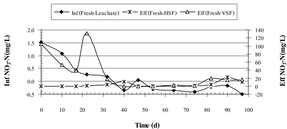
ภาพผนวกที่ ๖ \text{NO}_2\text{-N} ของ Fresh Leachate ระบบ HSF และ VSF Run 1
