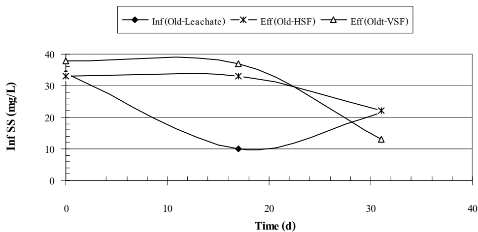
ภาพผนวกที่ ข74 SS ของ Old Leachate ระบบ HSF และ VSF Run 3
