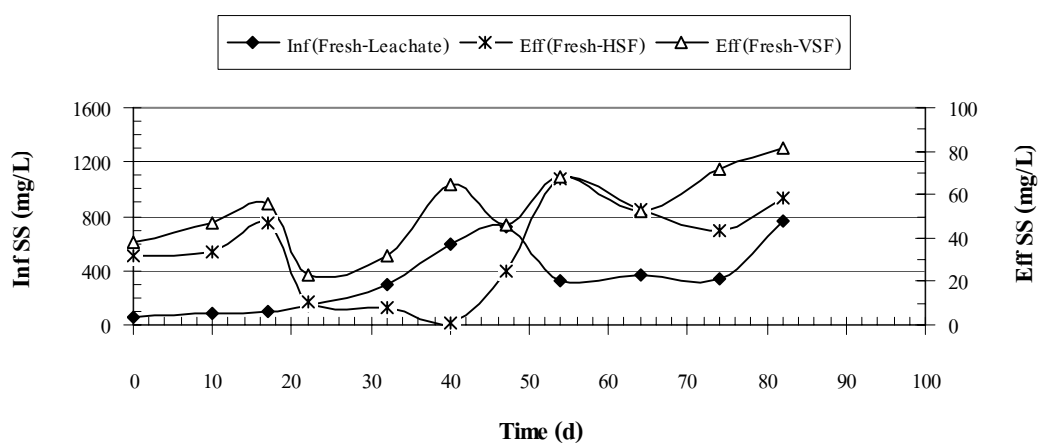
ภาพผนวกที่ ข9 SS ของ Fresh Leachate ระบบ HSF และ VSF Run 1
