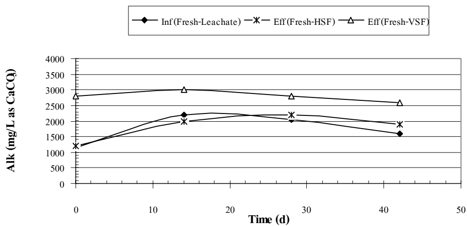
ภาพผนวกที่ ข36 Alk ของ Fresh Leachate ระบบ HSF และ VSF Run 2
