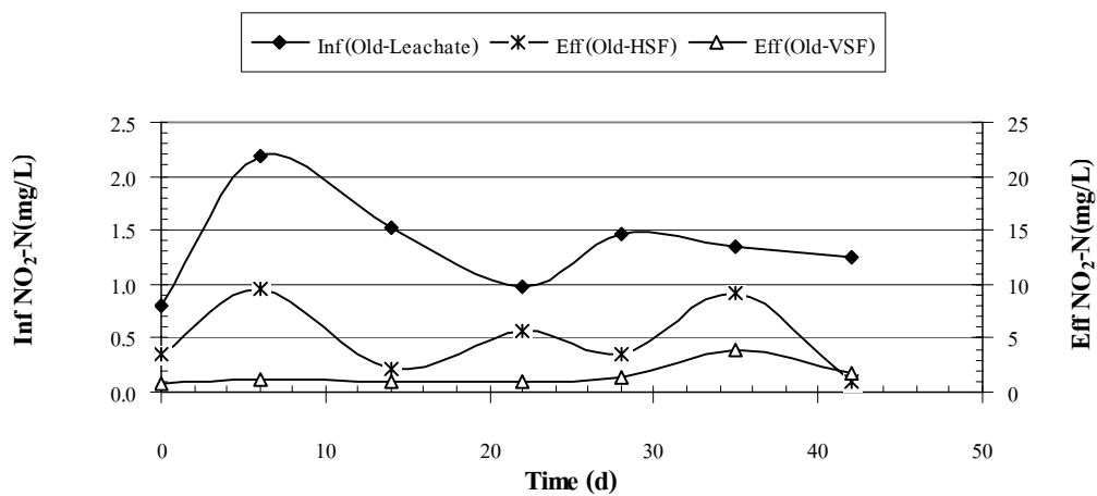
ภาพผนวกที่ ข45 NO 2 -N ของ Old Leachate ระบบ HSF และ VSF Run 2
