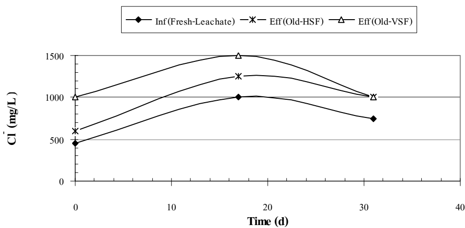
ภาพผนวกที่ ข63 Cl- ของ Fresh Leachate ระบบ HSF และ VSF Run 3
