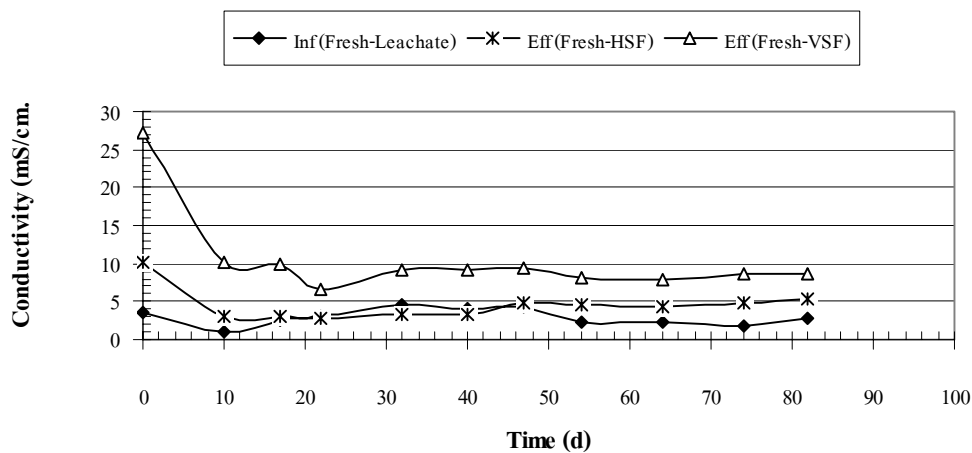
ภาพผนวกที่ ข13 EC ของ Fresh Leachate ระบบ HSF และ VSF Run 1
