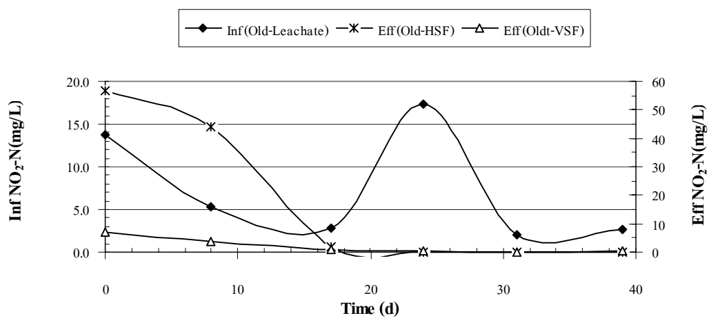
ภาพผนวกที่ ข71 NO 2 -N ของ Old Leachate ระบบ HSF และ VSF Run 3
