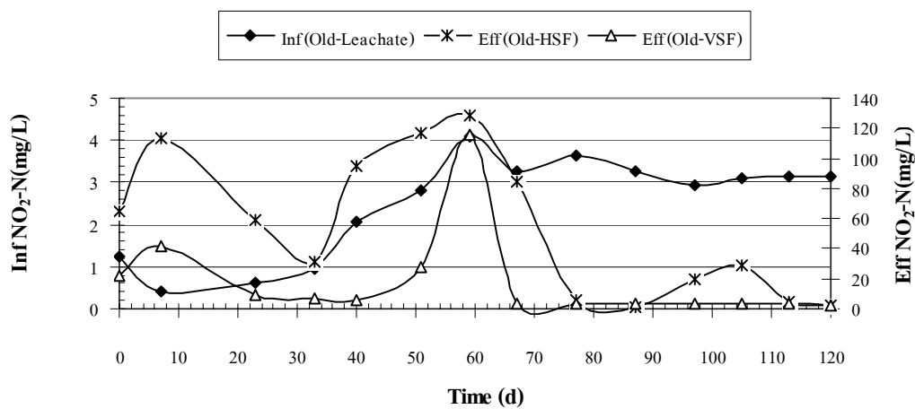
ภาพผนวกที่ ข19 \text{NO}_2\text{-N} ของ Old Leachate ระบบ HSF และ VSF Run 1
