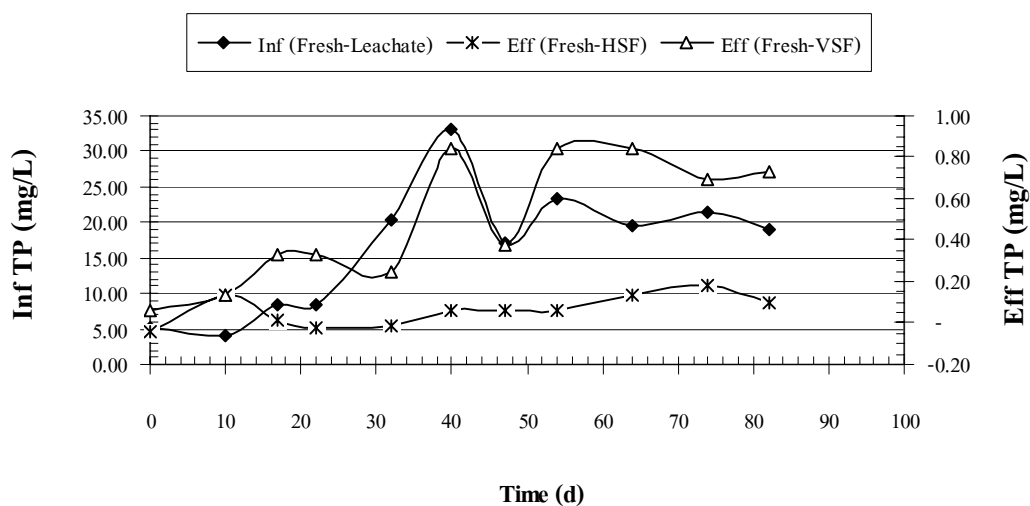
ภาพผนวกที่ ข8 TP ของ Fresh Leachate ระบบ HSF และ VSF Run 1
