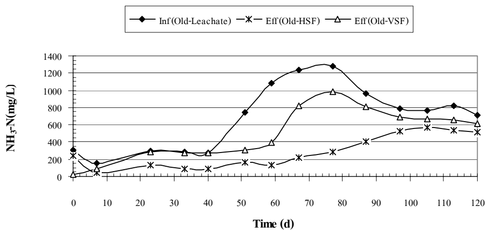
ภาพผนวกที่ ข18 NH 3 -N ของ Old Leachate ระบบ HSF และ VSF Run 1
