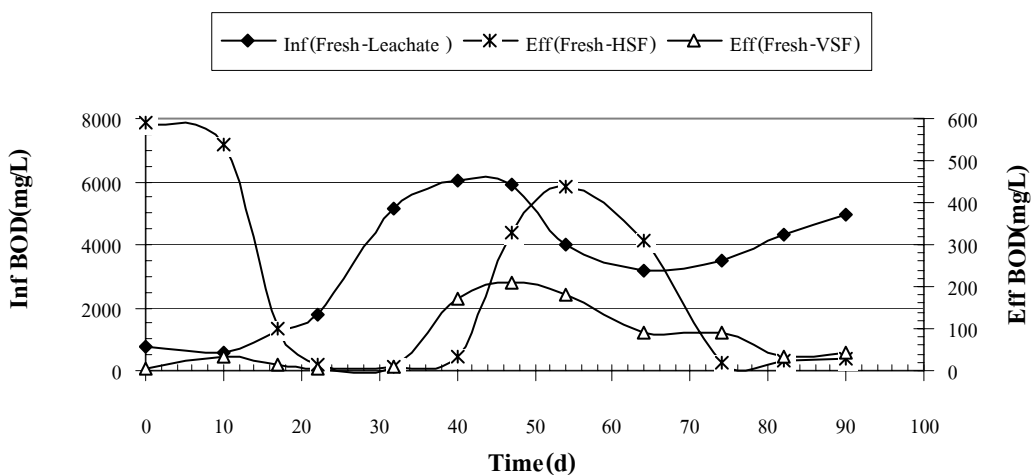
ภาพผนวกที่ ข3 SBOD ของ Fresh Leachate ระบบ HSF และ VSF Run 1
