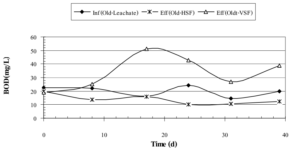
ภาพผนวกที่ ข68 SBOD ของ Old Leachate ระบบ HSF และ VSF Run 3
