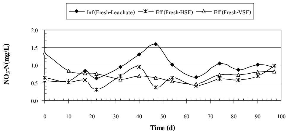
ภาพผนวกที่ ข7 \text{NO}_3\text{-N} ของ Fresh Leachate ระบบ HSF และ VSF Run 1
