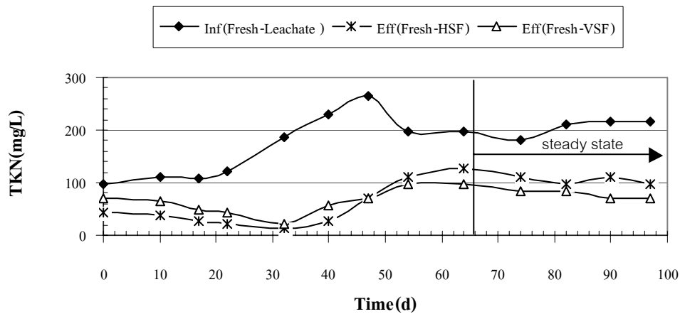
ภาพผนวกที่ ๔ TKN ของ Fresh Leachate ระบบ HSF และ VSF Run 1
