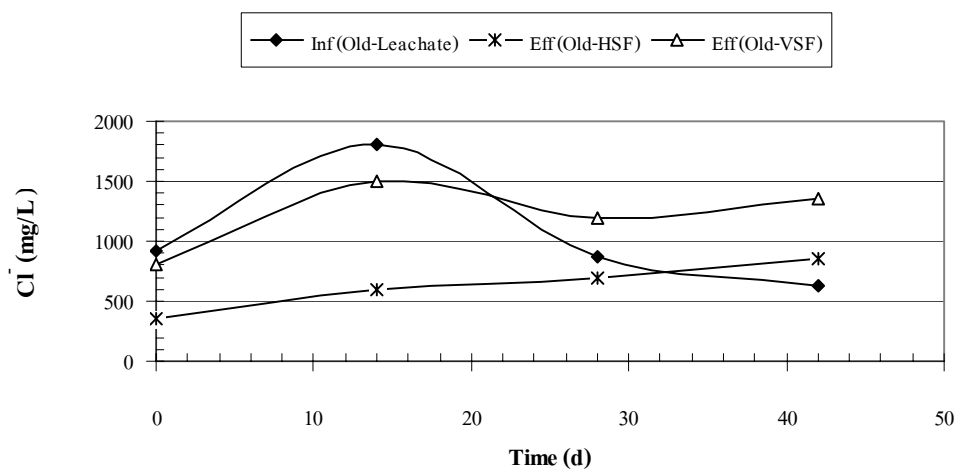
ภาพผนวกที่ ๕๐ Cl- ของ Old Leachate ระบบ HSF และ VSF Run 2
