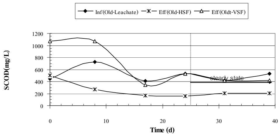
ภาพผนวกที่ ข67 SCOD ของ Old Leachate ระบบ HSF และ VSF Run 3
