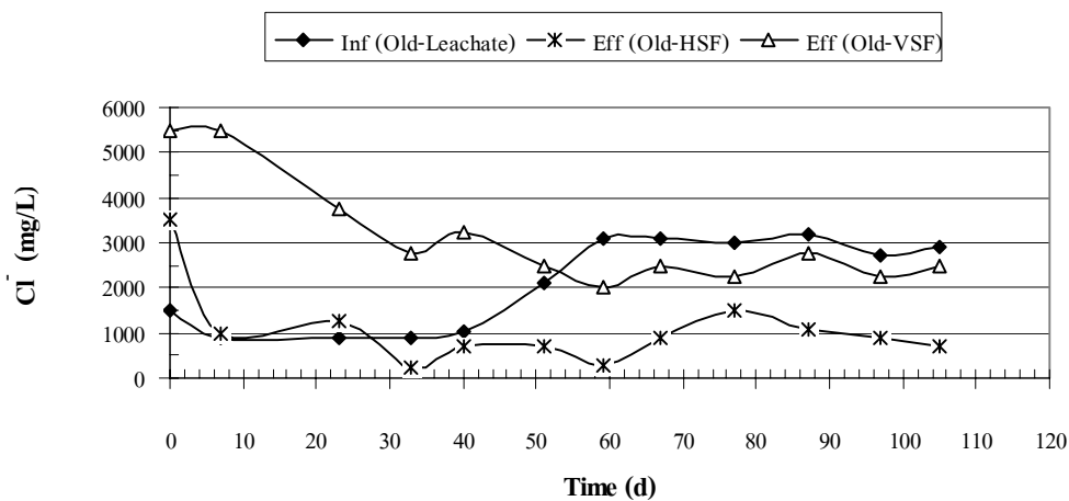
ภาพผนวกที่ ข24 Cl- ของ Old Leachate ระบบ HSF และ VSF Run 1
