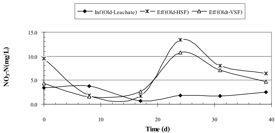
ภาพผนวกที่ ข72 NO 3 -N ของ Old Leachate ระบบ HSF และ VSF Run 3
