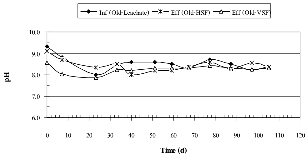
ภาพผนวกที่ ข25 pH ของ Old Leachate ระบบ HSF และ VSF Run 1
