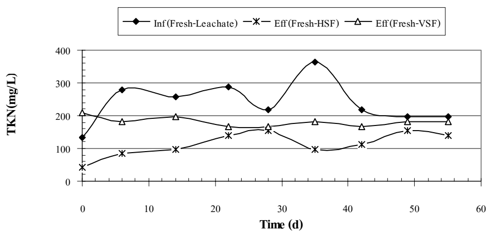
ภาพผนวกที่ ๒๓๐ TKN ของ Fresh Leachate ระบบ HSF และ VSF Run 2
