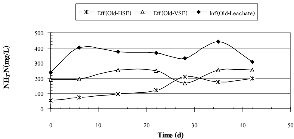
ภาพผนวกที่ ข44 NH 3 -N ของ Old Leachate ระบบ HSF และ VSF Run 2
