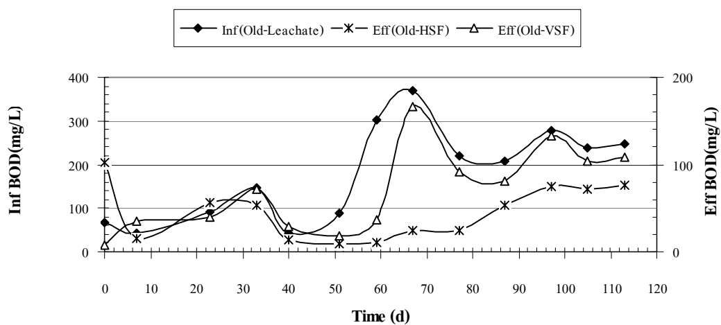
ภาพผนวกที่ ข16 SBOD ของ Old Leachate ระบบ HSF และ VSF Run 1
