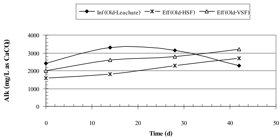
ภาพผนวกที่ ๔๙ Alk ของ Old Leachate ระบบ HSF และ VSF Run 2
