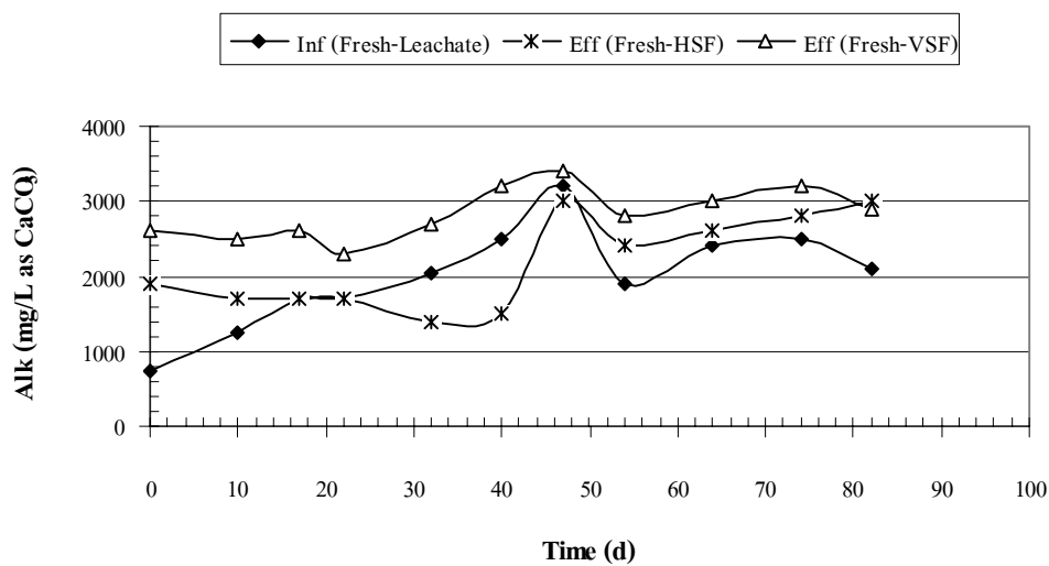
ภาพผนวกที่ ข10 Alk ของ Fresh Leachate ระบบ HSF และ VSF Run 1
