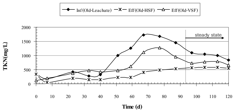
ภาพผนวกที่ ข17 TKN ของ Old Leachate ระบบ HSF และ VSF Run 1
