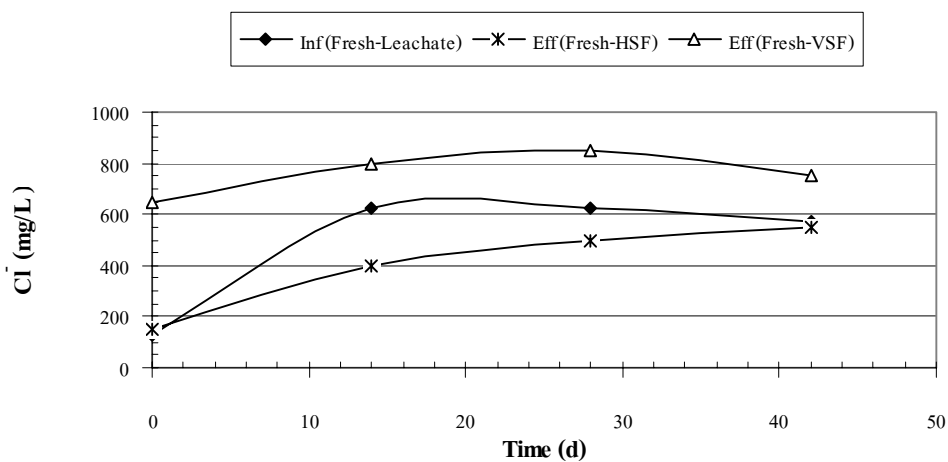
ภาพผนวกที่ ข37 Cl- ของ Fresh Leachate ระบบ HSF และ VSF Run 2
