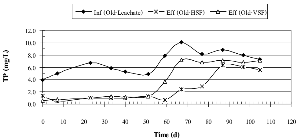
ภาพผนวกที่ ข21 TP ของ Old Leachate ระบบ HSF และ VSF Run 1
