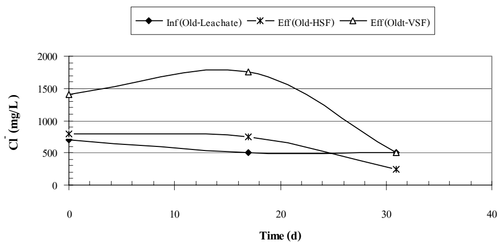
ภาพผนวกที่ ข76 Cl⁻ ของ Old Leachate ระบบ HSF และ VSF Run 3
