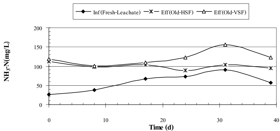
ภาพผนวกที่ ๕๗ \text{NH}_3\text{-N} ของ Fresh Leachate ระบบ HSF และ VSF Run 3
