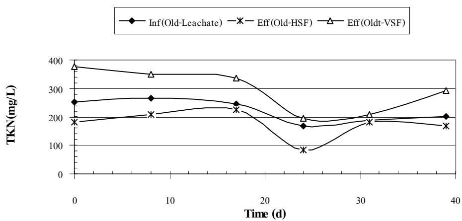
ภาพผนวกที่ ข69 TKN ของ Old Leachate ระบบ HSF และ VSF Run 3
