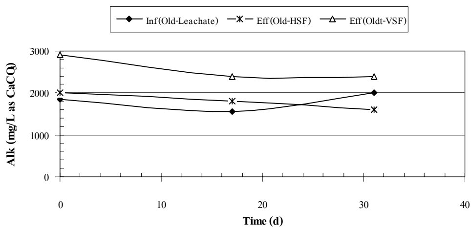
ภาพผนวกที่ ข75 Alk ของ Old Leachate ระบบ HSF และ VSF Run 3
