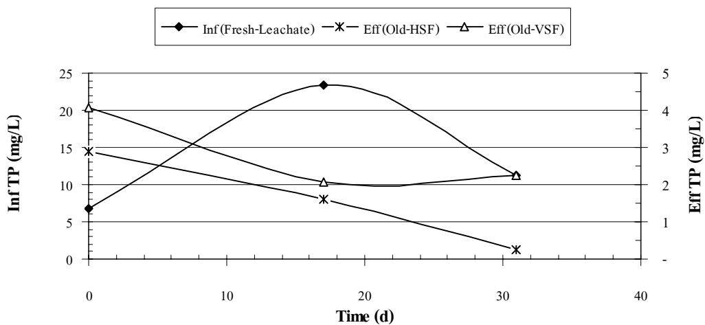
ภาพผนวกที่ ข60 TP ของ Fresh Leachate ระบบ HSF และ VSF Run 3
