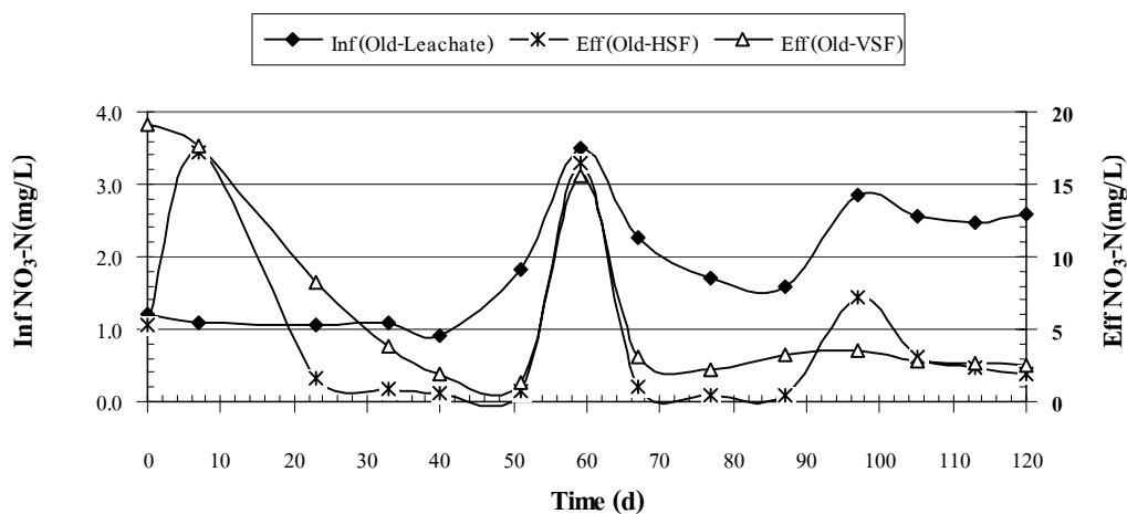
ภาพผนวกที่ ข20 \text{NO}_3\text{-N} ของ Old Leachate ระบบ HSF และ VSF Run 1
