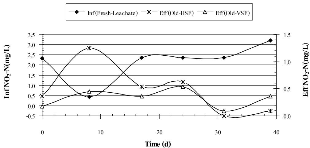
ภาพผนวกที่ ข58 NO 2 -N ของ Fresh Leachate ระบบ HSF และ VSF Run 3
