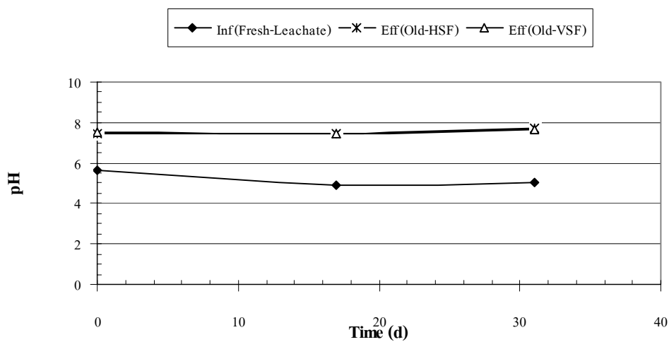
ภาพผนวกที่ ข64 pH ของ Fresh Leachate ระบบ HSF และ VSF Run 3
