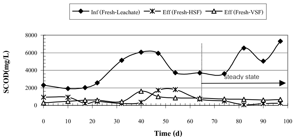
ภาพผนวกที่ ข2 SCOD ของ Fresh Leachate ระบบ HSF และ VSF Run 1
