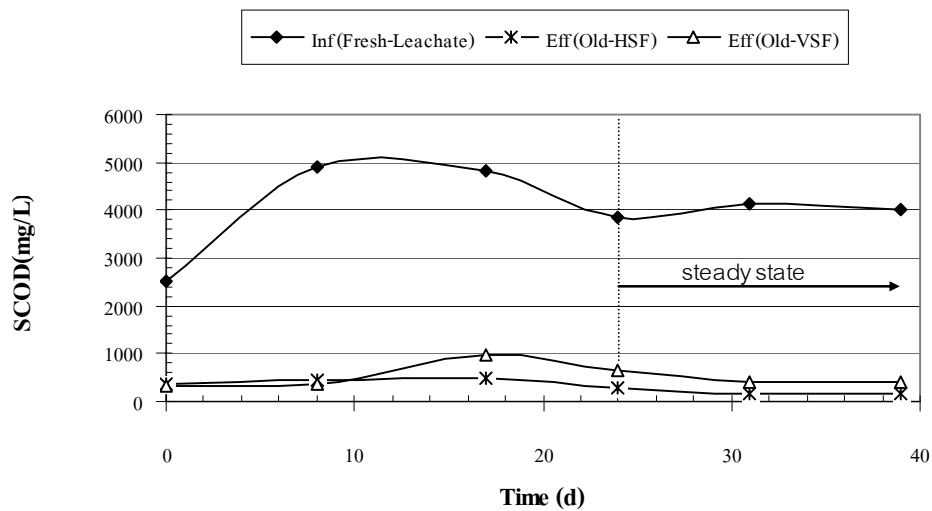
ภาพผนวกที่ ข54 SCOD ของ Fresh Leachate ระบบ HSF และ VSF Run 3
