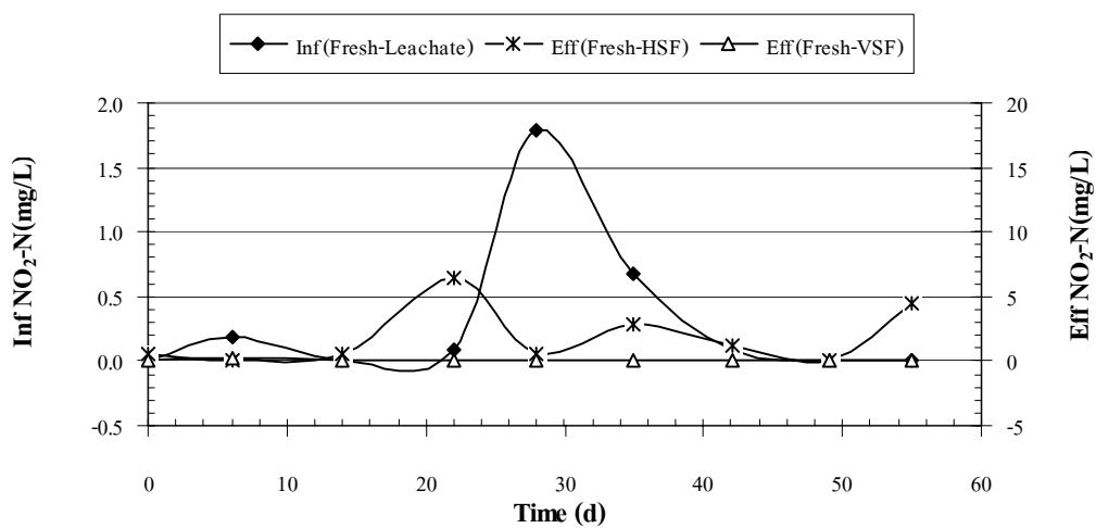
ภาพผนวกที่ ข32 \text{NO}_2\text{-N} ของ Fresh Leachate ระบบ HSF และ VSF Run 2
