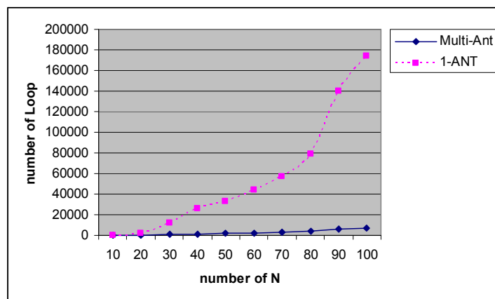
ภาพที่ 33 เปรียบเทียบจำนวนรอบของการทำงานระหว่างอัลกอริทึมอาณาจักรมดที่ใช้มดหลายตัวและการใช้มดตัวเดียวในการทำงาน เมื่อ n = 10, 20, 30, \dots, 90 เมื่ออัตราการระเหยเป็น 1/n
