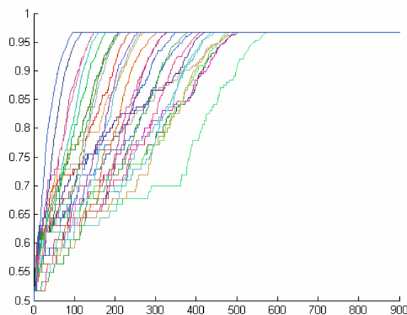
ภาพที่ 22 การปรับค่าของฟีโรโมนบนเส้นทางที่ x_i มีค่าเป็น 1 เมื่อเทียบกับเวลา multiple-ant algorithm สำหรับ One-Max โดยกำหนด n = 30 เมื่ออัตราการระเหยเป็น 1/n
