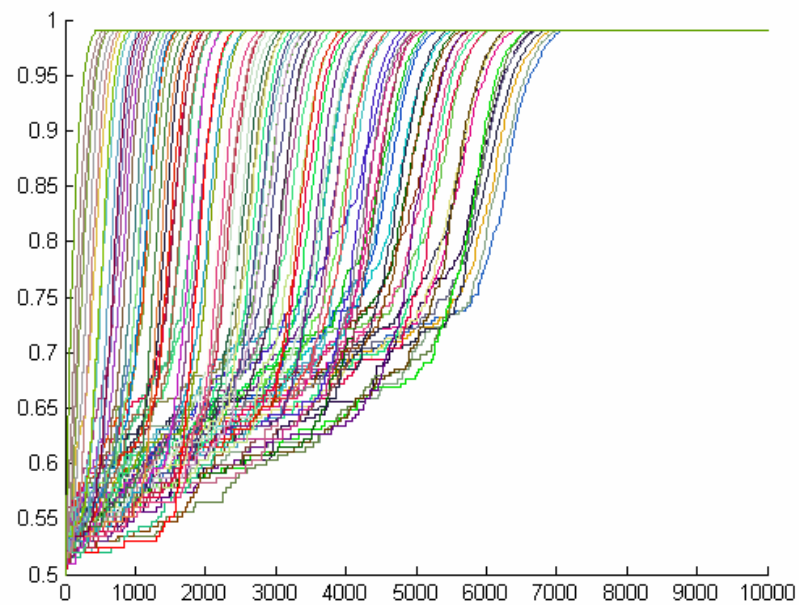
ภาพที่ 24 การปรับค่าของฟีโรโมนบนเส้นทางที่ x_i มีค่าเป็น 1 เมื่อเทียบกับเวลา multiple-ant algorithm สำหรับ One-Max โดยกำหนด n = 100 เมื่ออัตราการระเหยเป็น 1/n
