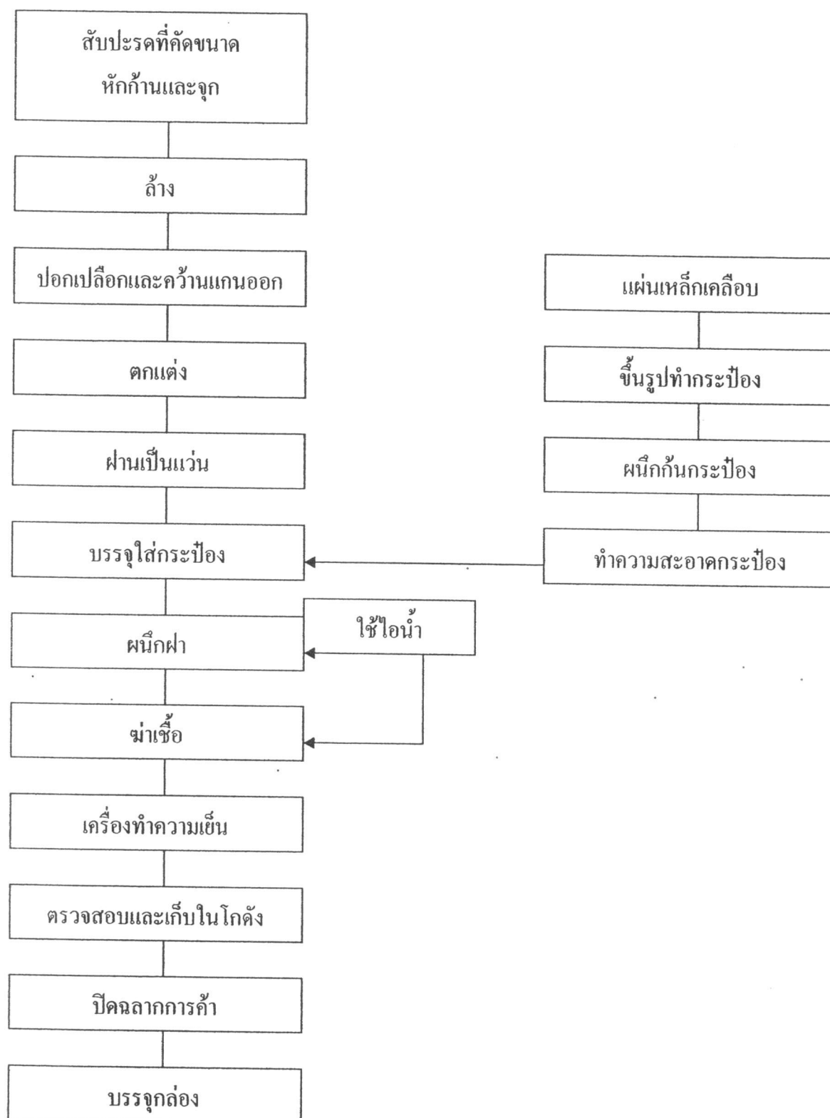
ภาพที่ 4.1 ขั้นตอนการผลิตของอุตสาหกรรมสับประดกระป๋อง
