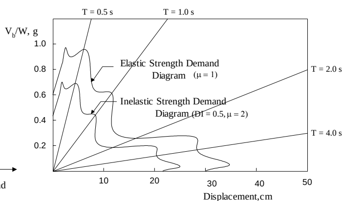
ภาพประกอบ 6ข Strength Demand Diagram
