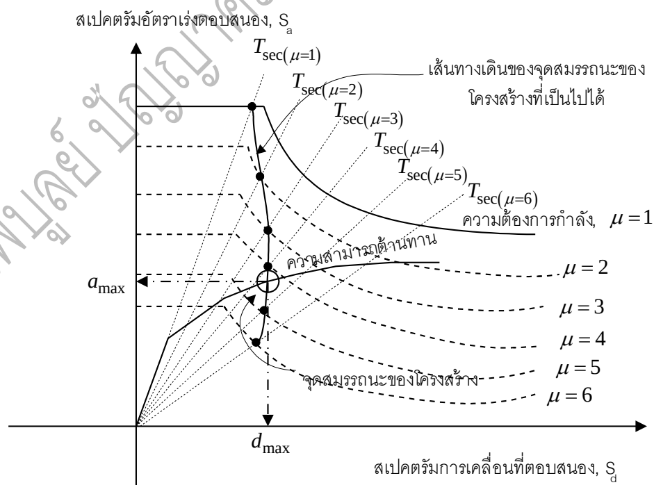
ภาพประกอบ 11 การหาจุดสมรรถนะของวิธีการสเปกตรัมของความสามารถปรับปรุงใหม่
