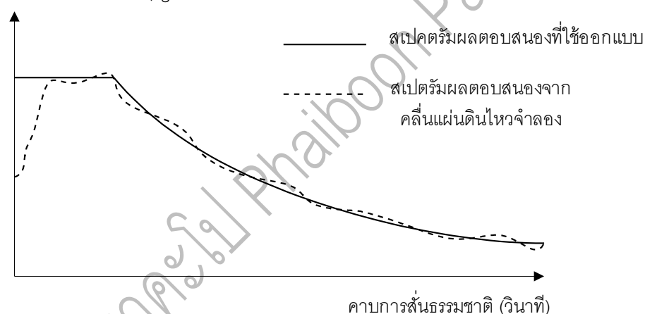
ภาพประกอบ 4 สเปกตรัมผลตอบสนองที่ใช้ออกแบบและผลจากคลื่นแผ่นดินไหวจำลอง
