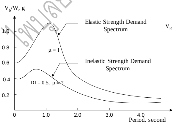
ภาพประกอบ 6ก Strength Demand Spectrum
