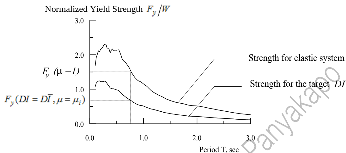
ภาพประกอบ 5 ค่าความต้องการกำลังระบบอีลาสติกและระบบความเสียหายคงที่ (ไพบูลย์ ปัญญาคะโป 2548, Panyakapo, P. 2002)
