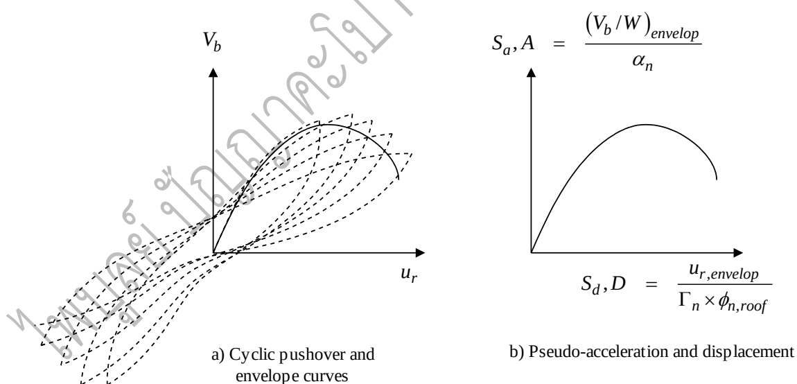
ภาพประกอบ 2 การเปลี่ยนจากกราฟการผลักอาคารแบบวิถจักรเป็นกราฟค่าอัตราเร่งเสมือนและค่าการเคลื่อนที่เสมือน (Capacity spectrum)
