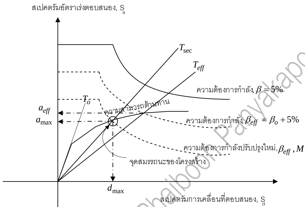
ภาพประกอบ 10 วิธีการสเปกตรัมของความสามารถปรับปรุงใหม่
