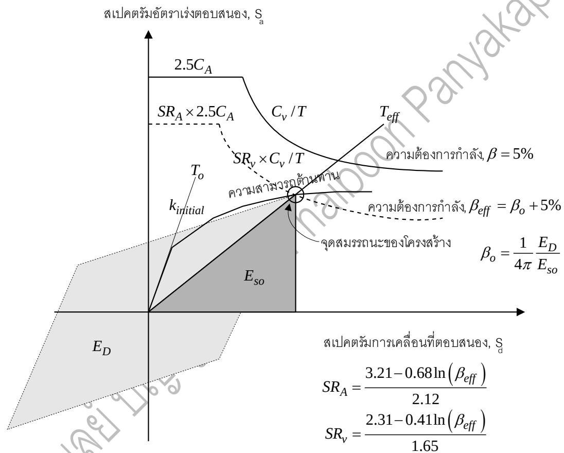
ภาพประกอบ 9 วิธีการสเปกตรัมของความสามารถ (Capacity Spectrum Method) โดย ATC-40
