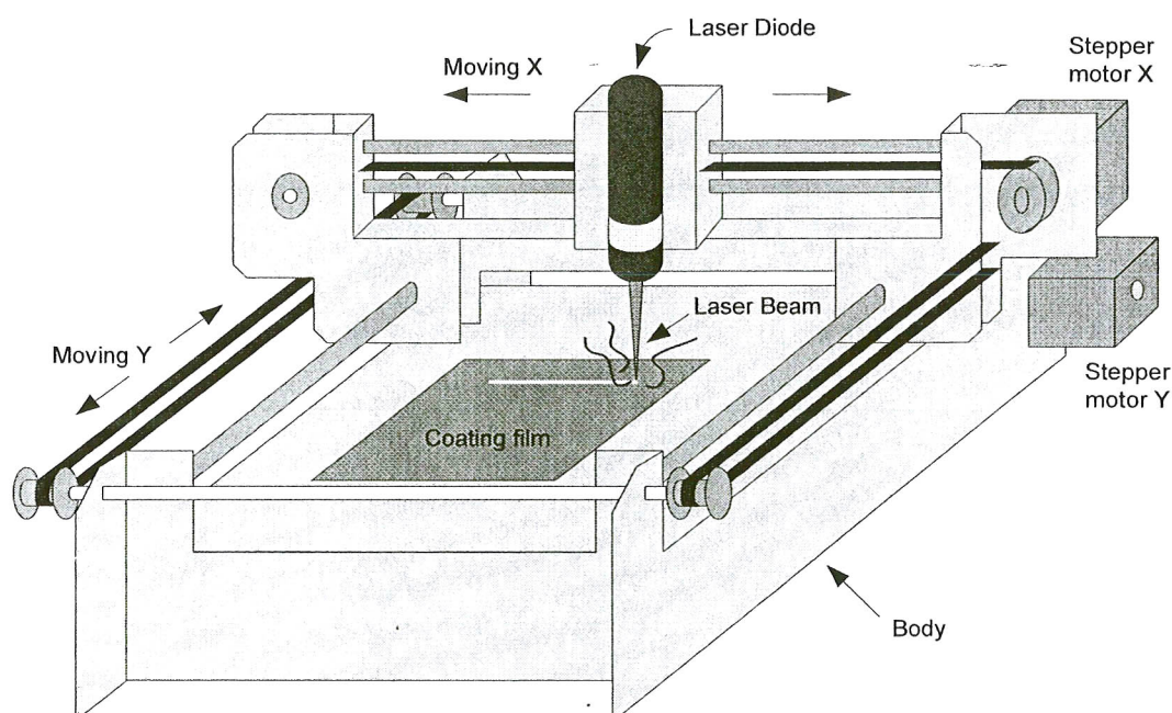
รูปที่ 3.10 แบบจำลองแสดงให้เห็นโครงสร้างต่างๆ ของเครื่อง
