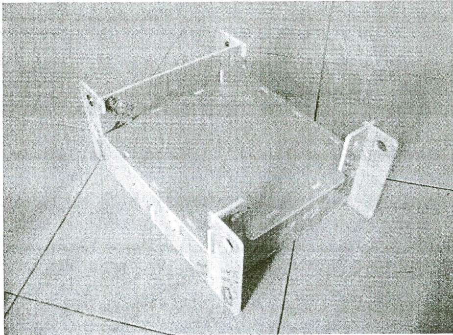
รูปที่ 3.14 แสดงส่วนของโครงสร้างของเครื่องและแกน Y ที่ประกอบกันเสร็จเรียบร้อยแล้ว
