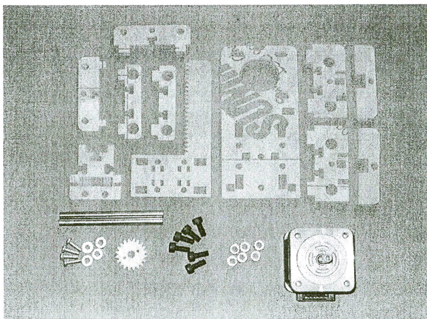
รูปที่ 3.19 แสดงชิ้นส่วนของส่วนที่ยึดหัวเลเซอร์ เป็นแผ่นอะคริลิกหนา 5 mm.
