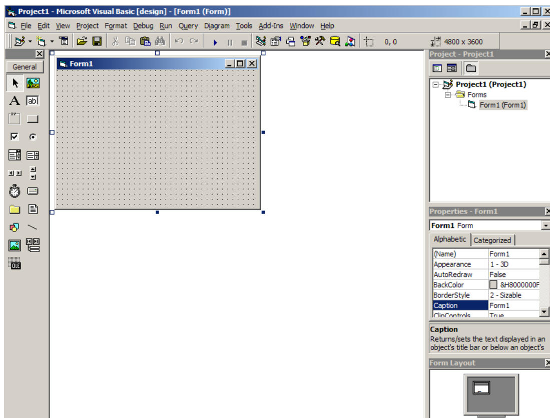
รูปที่ 4.11 แสดงส่วนประกอบต่างๆ ของโปรแกรม Visual Basic 6.0
