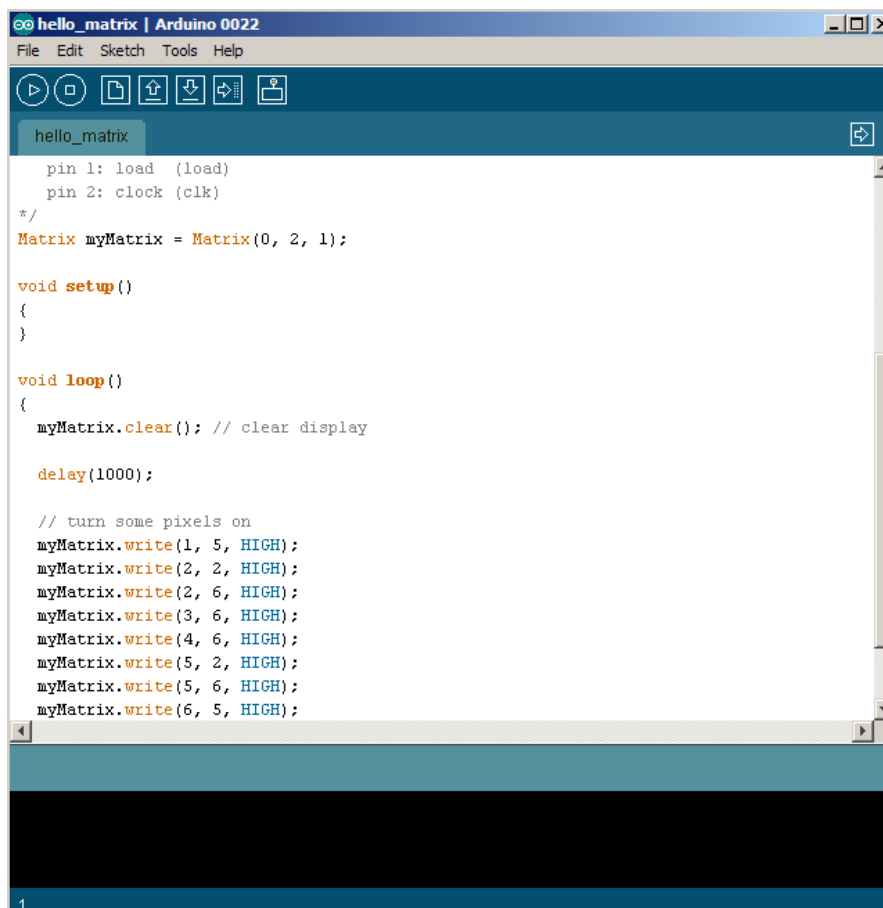
รูปที่ 4.12 แสดงส่วนประกอบต่างๆ ของโปรแกรม Arduino V22
