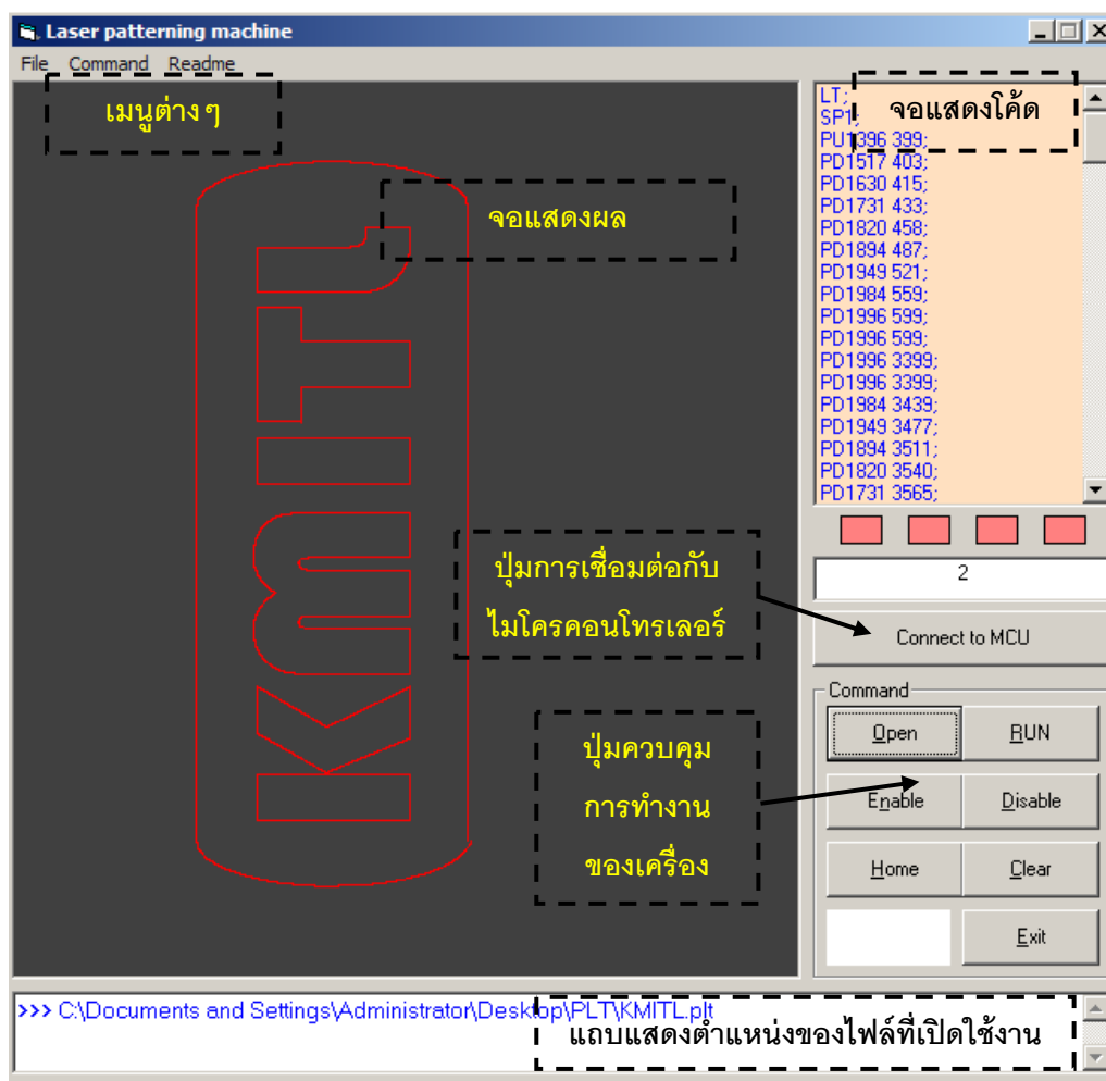
รูปที่ 4.19 หน้าต่างแสดงส่วนประกอบต่างๆ ของโปรแกรม Laser Patterning Machine
