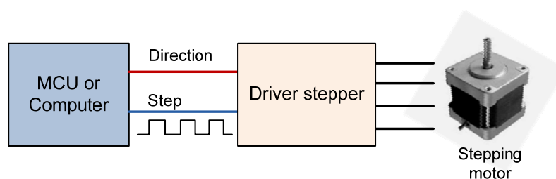
รูปที่ 4.4 หลักการใช้งานไดรเวอร์สเต็ปมอเตอร์ขั้นพื้นฐาน
