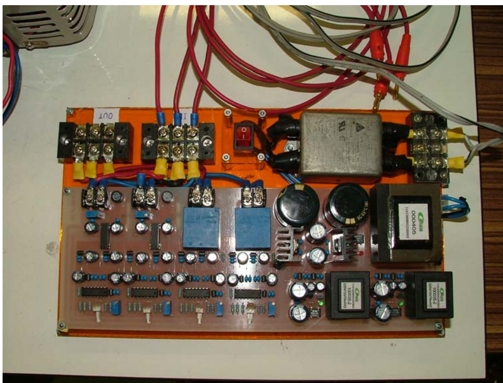
วงจรตรวจจับแรงดันและกระแสอินพุท
