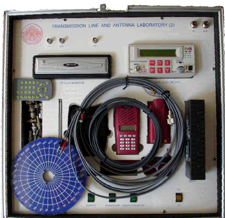
รูปที่ น8 แสดงรูปกล่อง Transmission Line and Antenna Lab 2
