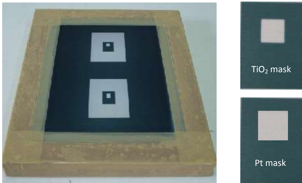
รูปที่ 2.2 บล็อกพิมพ์สกรีนแม่พิมพ์ต้นแบบของ TiO 2 และ Pt
