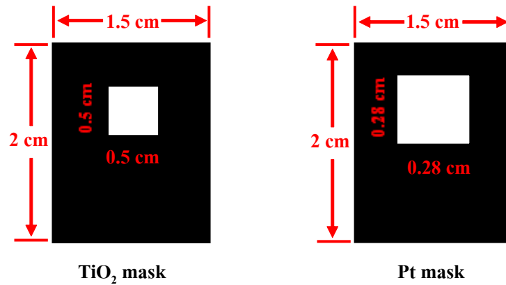
รูปที่ 2.1 ต้นแบบลวดลายมาร์กของ TiO 2 และ Pt
