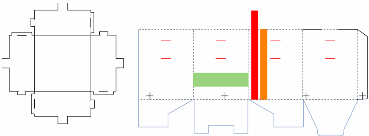
ภาพที่ ค.6 แบบร่างโครงสร้างบรรจุภัณฑ์
