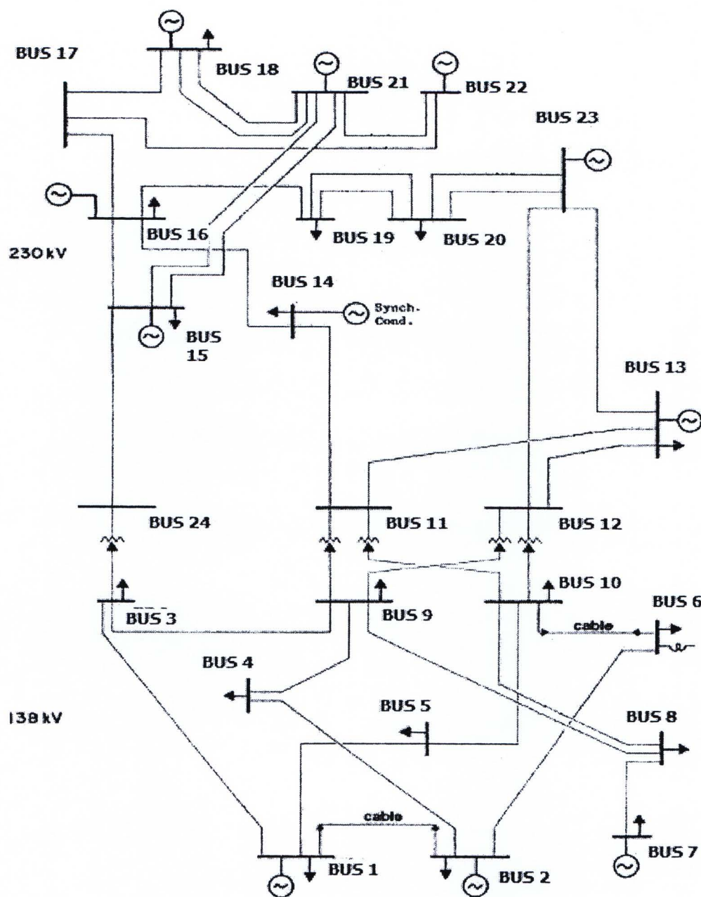
รูปที่ ก.1 ไดอะแกรมระบบทดสอบ IEEE RTS-79
