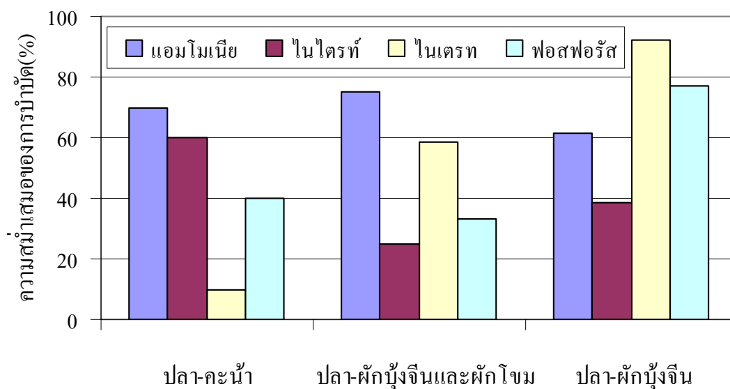
ภาพที่ ง.2 ความสม่ำเสมอในการบำบัดแอมโมเนีย ไนไตรท์ ไนเตรท และฟอสฟอรัสที่ละลายในน้ำเจือย (%) ของระบบ DRFT-Fish ทั้ง 3 การทดลอง
