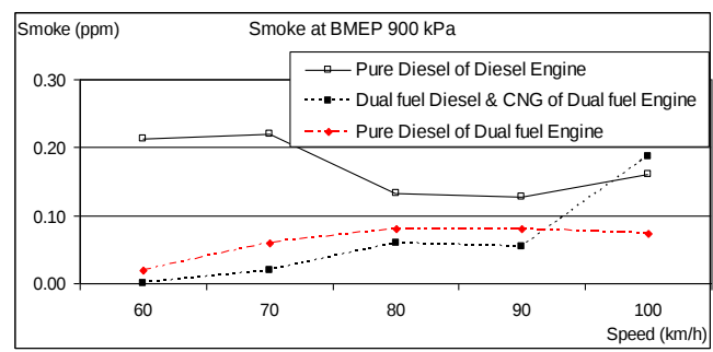
รูปที่ 17 ปริมาณควันดำที่ 900 kPa BMEP CNGกับดีเซล
