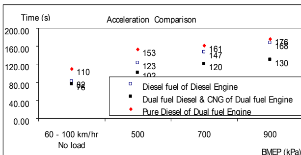
รูปที่ 21 ผลการทดสอบวัดอัตราเร่งของรถยนต์ CNGกับดีเซล
