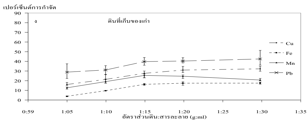
รูปที่ 4.2 ประสิทธิภาพการชะล้างโลหะหนักออกจากดินตัวอย่างเมื่อแปรผันอัตราส่วนระหว่างดินกับสารละลายโซเดียมอิตีทีเอ
