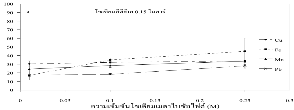
รูปที่ 4.3 ประสิทธิภาพการชะล้างโลหะหนักออกจากดินอุรุต (1)
