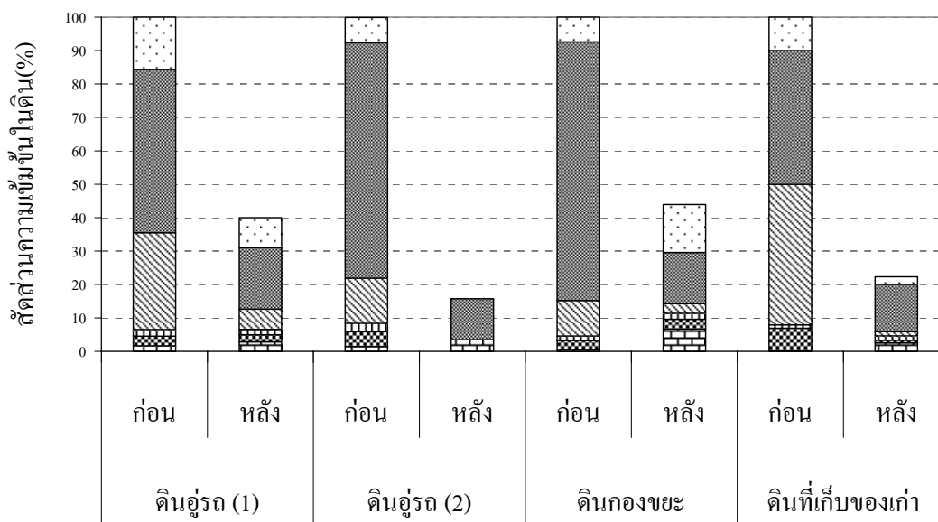
รูปที่ 4.24 สัดส่วนทองแดงในดินตัวอย่างก่อนและหลังการชะแบบคอลลัมน์
