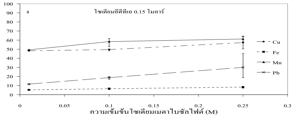
รูปที่ 4.4 ประสิทธิภาพการชะล้างโลหะหนักออกจากดินอุรูด (2)
