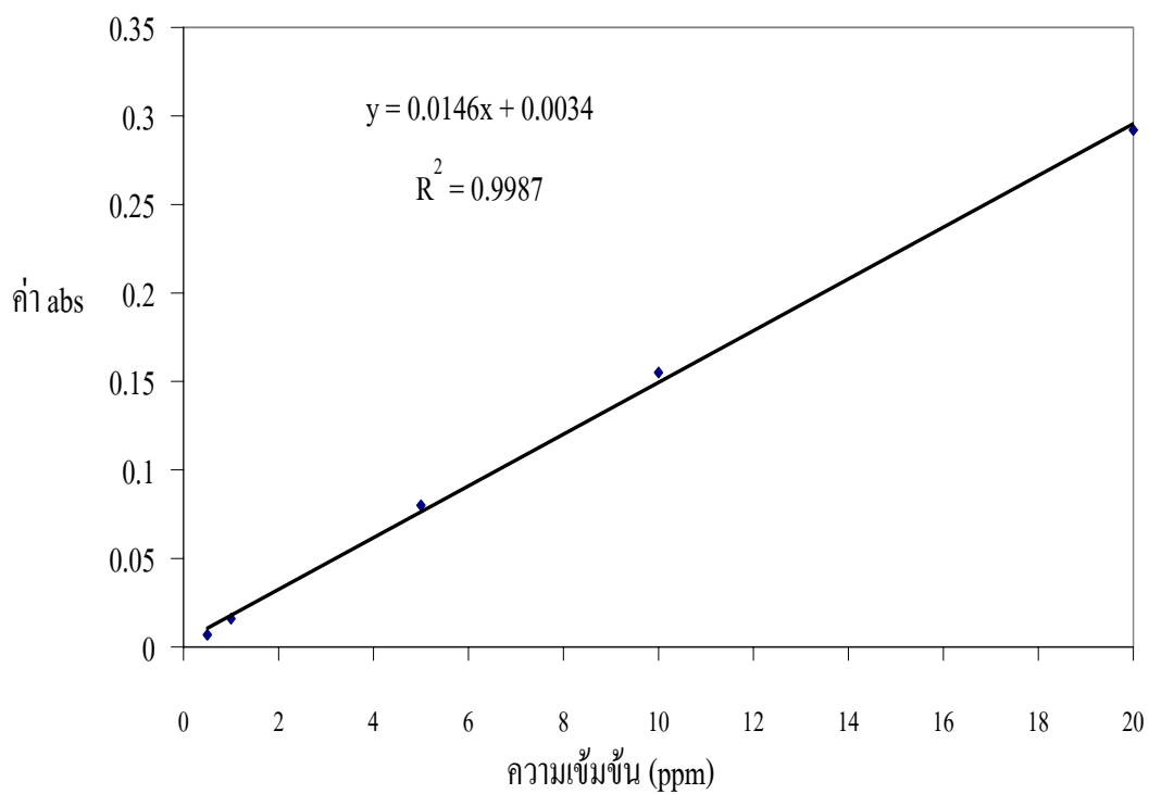
รูป ค.4 กราฟมาตรฐานของตะกั่ว
