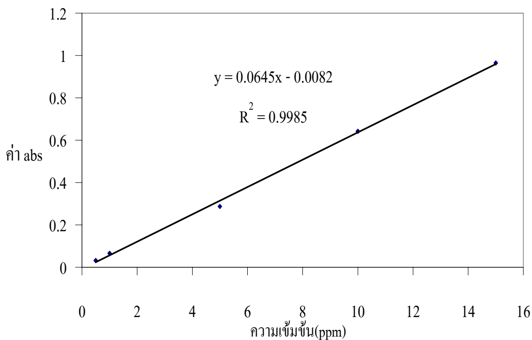
รูปที่ ค.1 กราฟมาตรฐานของทองแดง
