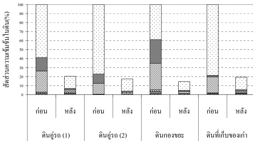
รูปที่ 4.25 สัดส่วนหลักในดินตัวอย่างก่อนและหลังการชะแบบคอลัมน์
