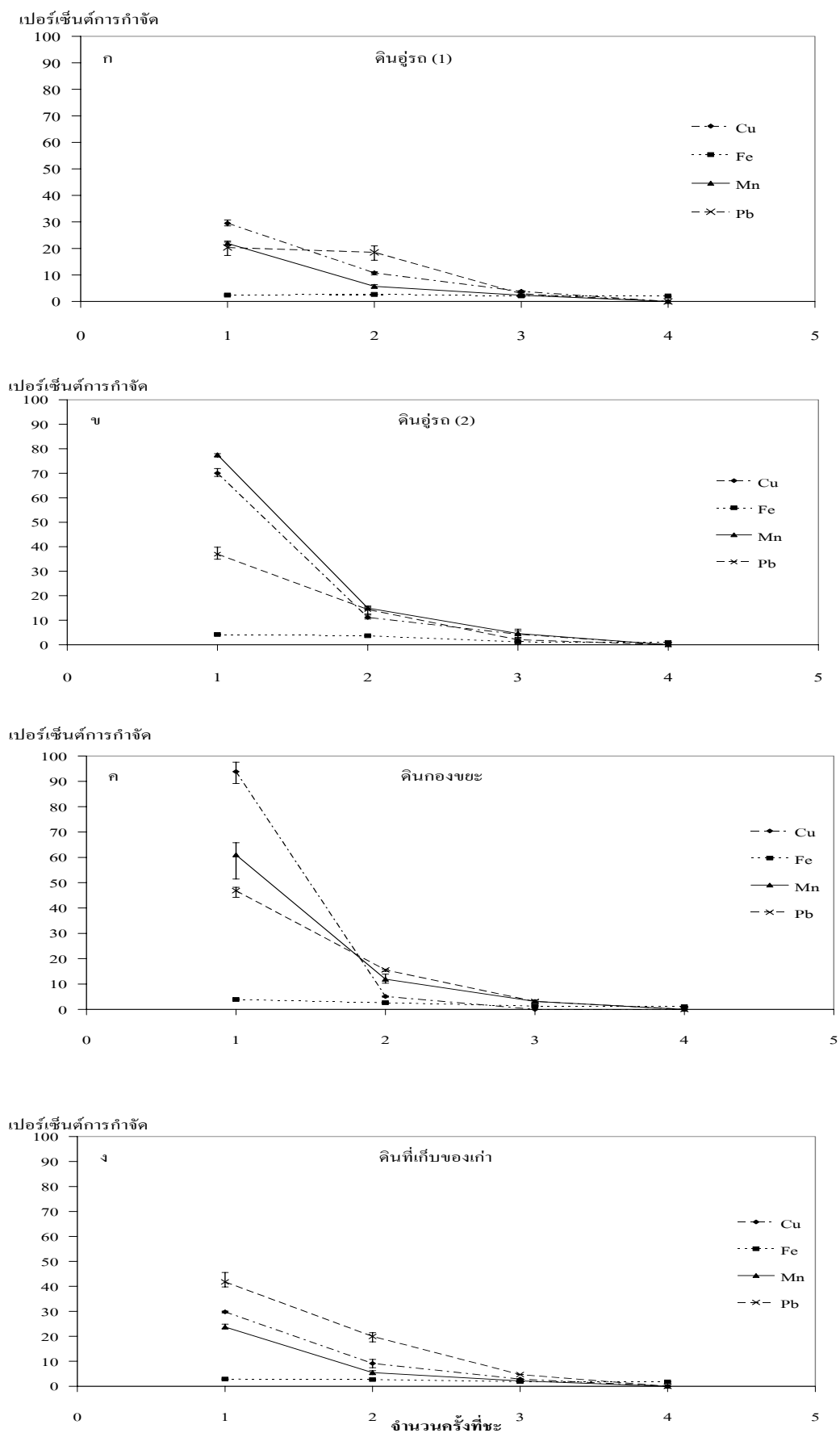
รูปที่ 4.28 การนำสารละลายโซเดียมไฮดรอกไซด์ที่เอกล้างมาใช้ใหม่
