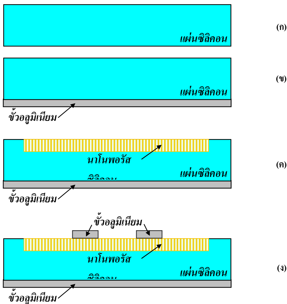
รูปที่ 4.2 ขั้นตอนการสร้างอุปกรณ์ตรวจจับไอระเหยของสารเคมีโดยใช้ชั้นนาโนพอร์ซิลิคอน
