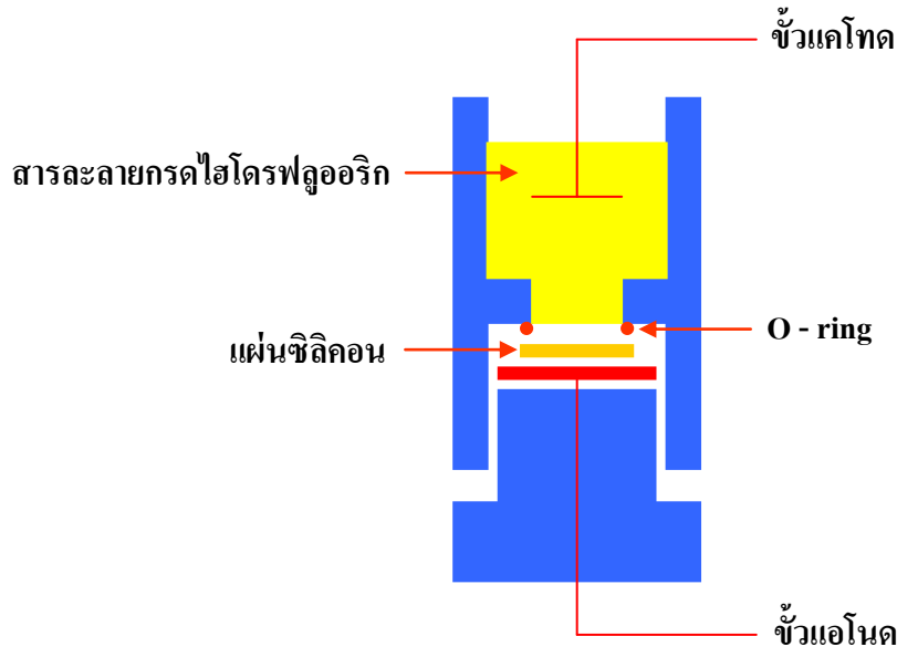
รูปที่ 4.1 อุปกรณ์เซลล์ไฟฟ้าเคมีแบบเซลล์แท็งก์เดี่ยวในแนวดิ่งใช้ในกระบวนการแอนโนไดซ์เซชัน
