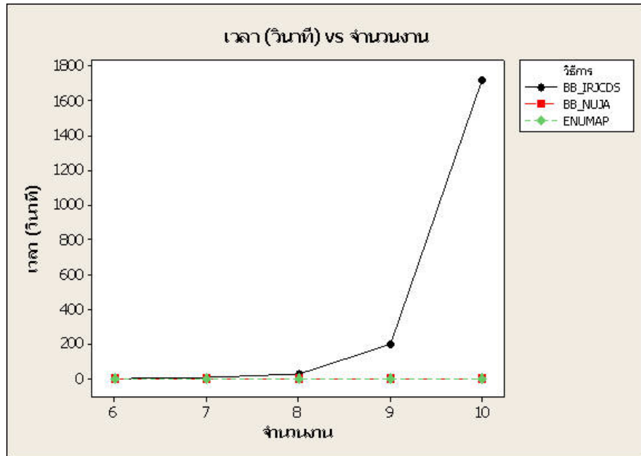
ภาพที่ 11 แสดงความสัมพันธ์ระหว่างเวลาในการคำนวณกับจำนวนงานของวิธีการต่างๆ (2 เครื่องจักร)
