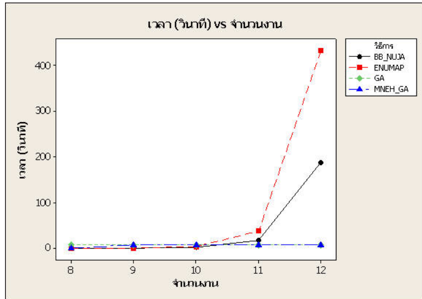
ภาพที่ 23 แสดงความสัมพันธ์ระหว่างเวลาในการคำนวณกับจำนวนงานของวิธีต่างๆ (10 เครื่องจักร)
