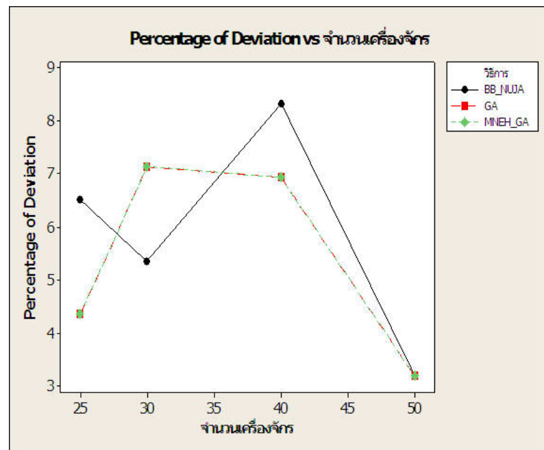
ภาพที่ 33 แสดงความสัมพันธ์ระหว่างเปอร์เซ็นต์ความคลาดเคลื่อนกับจำนวนเครื่องจักร (12 งาน)
