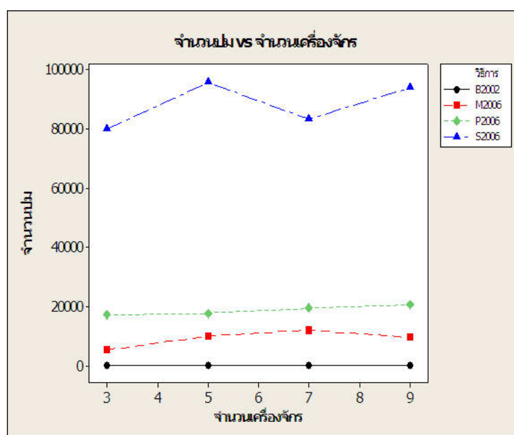
ภาพที่ 39 แสดงความสัมพันธ์ระหว่างจำนวนปมกับจำนวนเครื่องจักรของวิธีต่างๆ (12 งาน)
