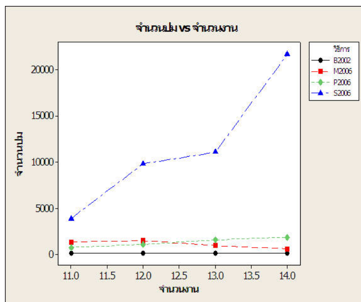
ภาพที่ 38 แสดงความสัมพันธ์ระหว่างจำนวนปมกับจำนวนงานของวิธีต่างๆ (4 เครื่องจักร)
