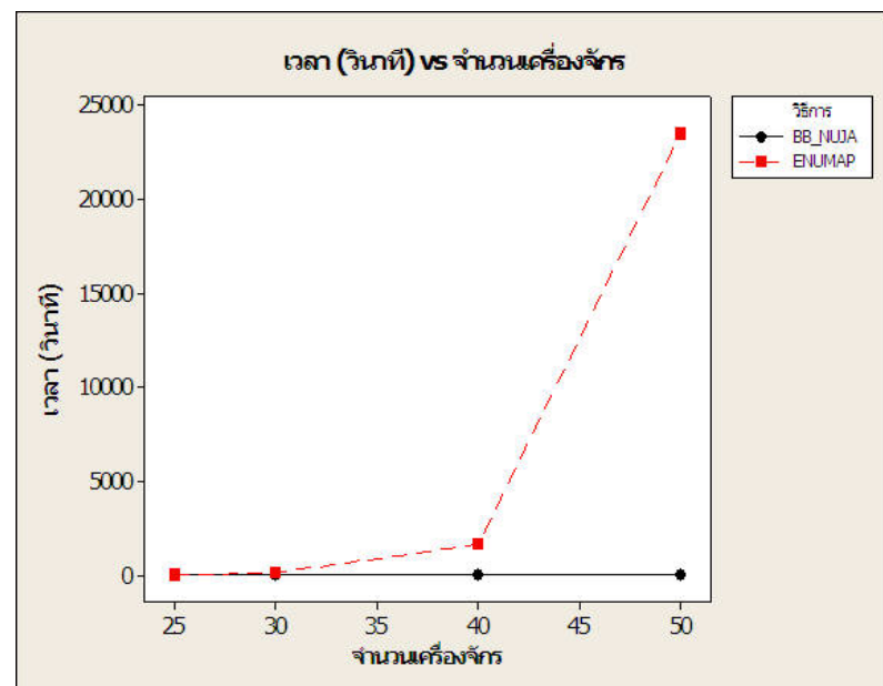
ภาพที่ 31 แสดงความสัมพันธ์ระหว่างเวลาในการคำนวณกับจำนวนเครื่องจักร (12 งาน)
