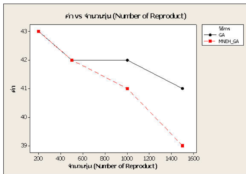
ภาพที่ 29 แสดงความสัมพันธ์ระหว่างค่าผลลัพธ์กับจำนวนรุ่นของประชากรในวิธี GA (กรณี 18 งาน 12 เครื่องจักร)
