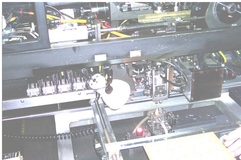
ภาพที่ 48 เครื่องจักรวางอุปกรณ์แบบ Axial Lead
