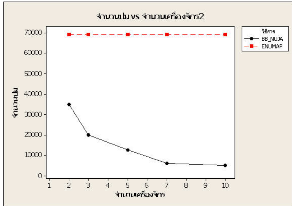
ภาพที่ 14 แสดงความสัมพันธ์ระหว่างจำนวนปมกับจำนวนเครื่องจักรของวิธีการ BB_NUJA (8 งาน)
