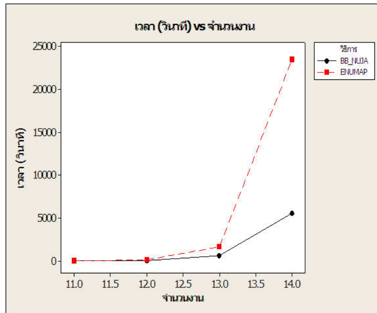
ภาพที่ 27 แสดงความสัมพันธ์ระหว่างเวลาในการคำนวณกับจำนวนงานของวิธี BB_NUJA (2 เครื่องจักร)
