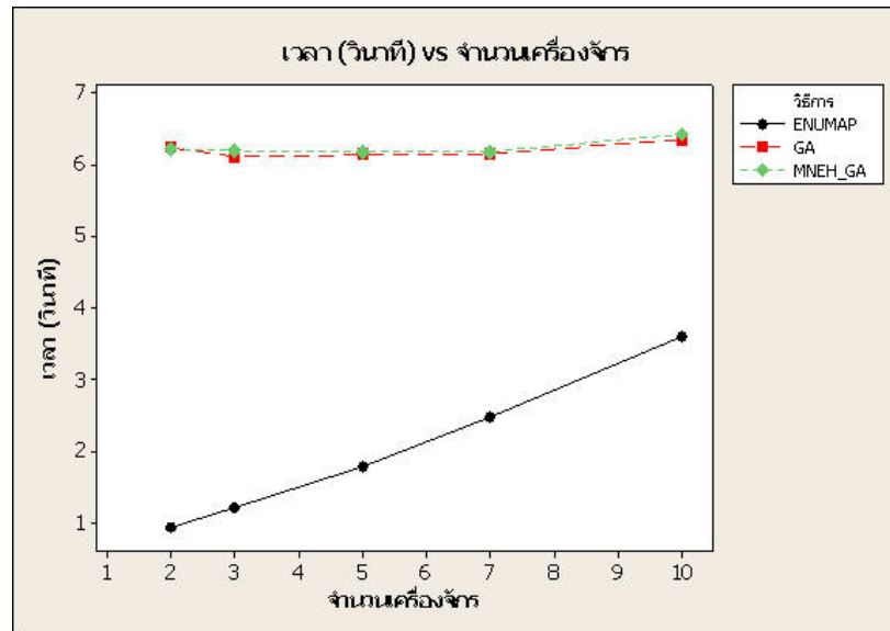
ภาพที่ 20 แสดงความสัมพันธ์ระหว่างเวลาคำนวณกับจำนวนเครื่องจักร ของวิธี GA, MNEH_GA และ ENUMAP (10 งาน)
