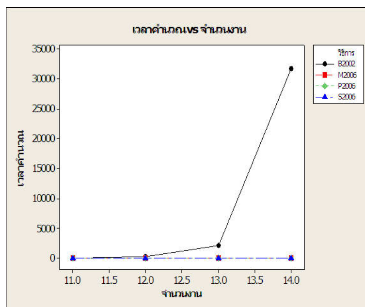
ภาพที่ 41 แสดงความสัมพันธ์ระหว่างเวลาในการคำนวณกับจำนวนงานของวิธีแตกกิ่งและจำกัดเขตแบบต่างๆ (4 เครื่องจักร)
