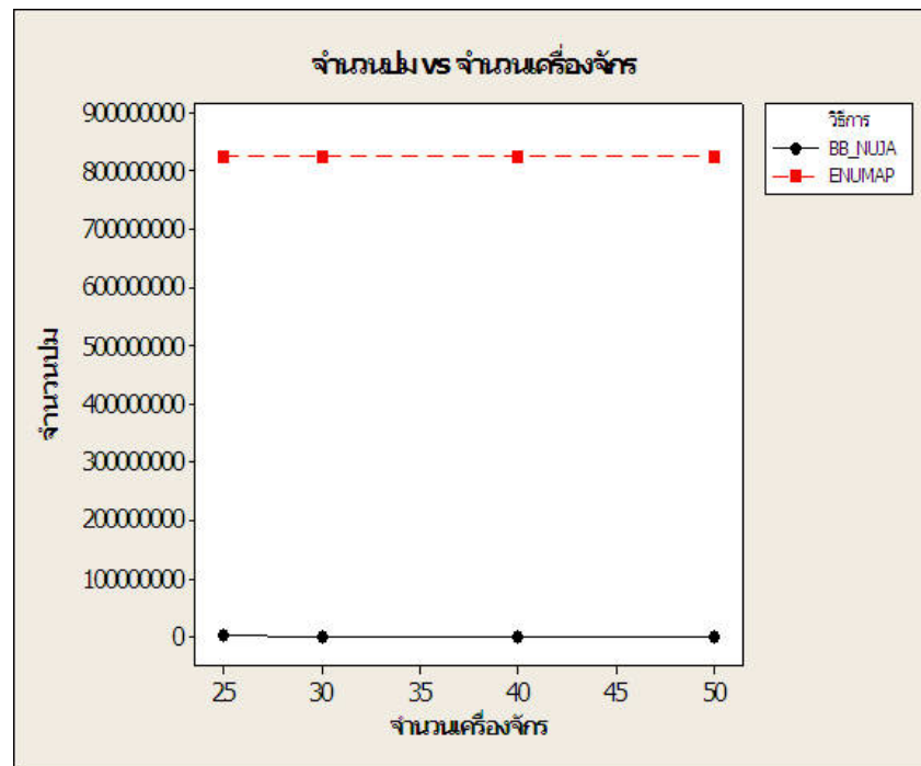
ภาพที่ 32 แสดงความสัมพันธ์ระหว่างจำนวนปมกับจำนวนเครื่องจักร (12 งาน)
