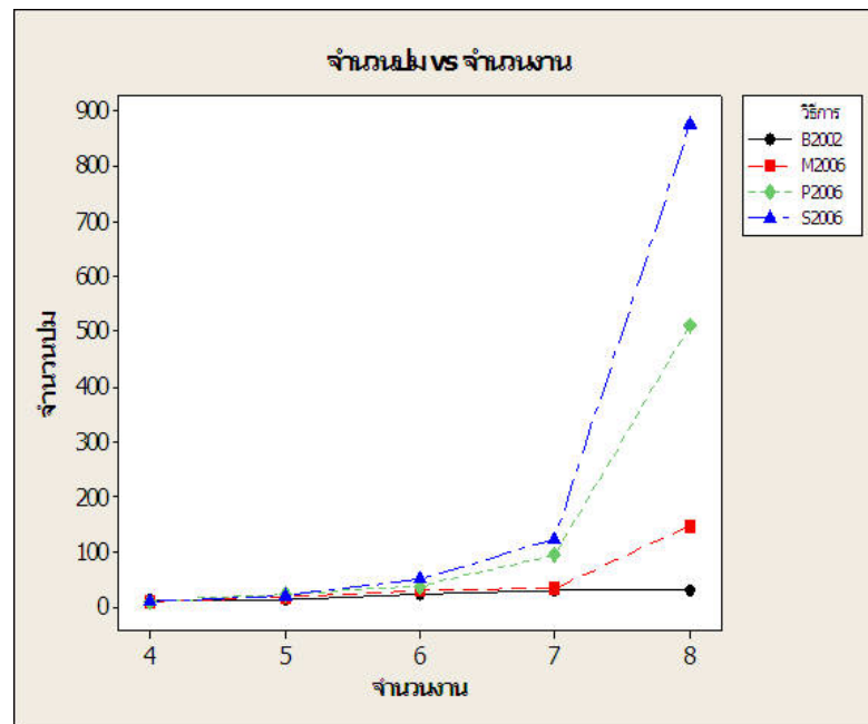
ภาพที่ 34 แสดงความสัมพันธ์ระหว่างจำนวนปมกับจำนวนงานของวิธีการต่างๆ (3 เครื่องจักร)
