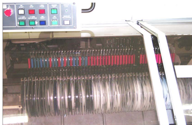
ภาพที่ 52 ฟีดเดอร์เครื่องวาง Chip
