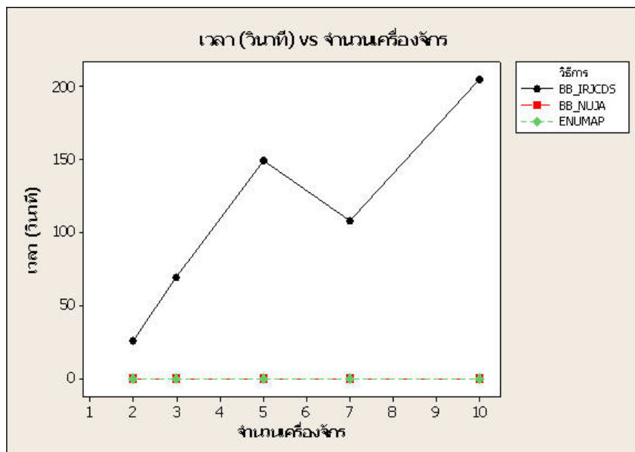
ภาพที่ 12 แสดงความสัมพันธ์ระหว่างเวลาในการคำนวณกับจำนวนเครื่องจักรของวิธีการแตกกิ่งที่เสนอ (8 งาน)
