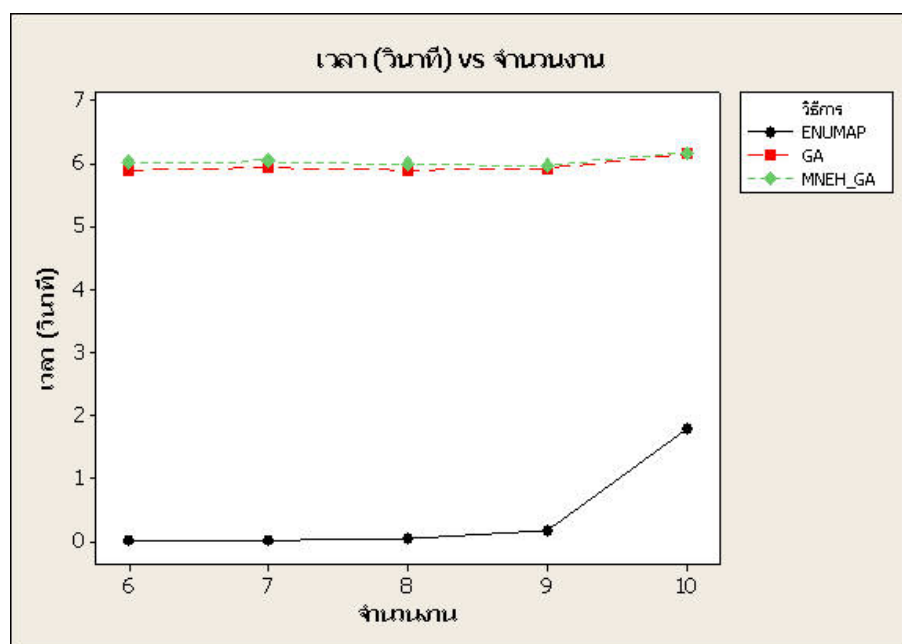
ภาพที่ 19 แสดงความสัมพันธ์ระหว่างเวลาคำนวณกับจำนวนงาน ของวิธี ENUMAP, GA และ MNEH_GA (5 เครื่องจักร)
