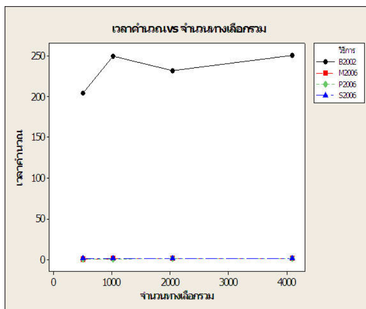
ภาพที่ 42 แสดงความสัมพันธ์ระหว่างเวลาในการคำนวณกับจำนวนทางเลือกรวมของวิธีต่างๆ (กรณี 12 งาน 5 เครื่องจักร)
