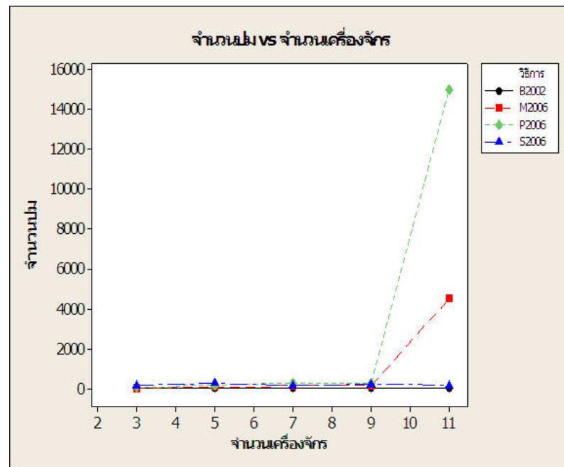
ภาพที่ 36 แสดงความสัมพันธ์ระหว่างจำนวนปมกับจำนวนเครื่องจักรของวิธีแตกกิ่งและจำกัดเขตแบบต่างๆ (7 งาน)
