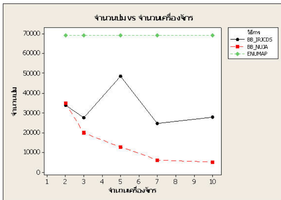
ภาพที่ 10 แสดงความสัมพันธ์ระหว่างเวลาจำนวนปมกับจำนวนเครื่องจักรของวิธีการต่างๆ (8 งาน)
