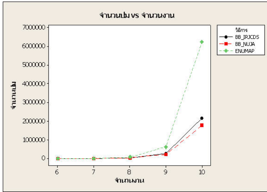
ภาพที่ 9 แสดงความสัมพันธ์ระหว่างจำนวนปมกับจำนวนงานของวิธีการต่างๆ (2 เครื่องจักร)
