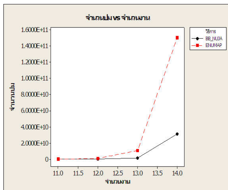
ภาพที่ 28 แสดงความสัมพันธ์ระหว่างจำนวนปมกับจำนวนงานของวิธี BB_NUJA (2 เครื่องจักร)
