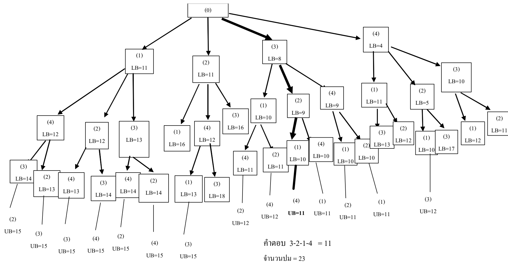
ภาพผนวกที่ ก4 แผนภูมิต้นไม้ของวิธี BB_NUJA กรณี 4 งาน 3 เครื่องจักร
