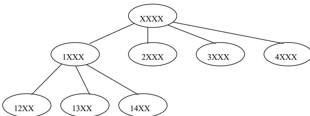
ภาพที่ 2 แขนงเซตย่อยของวิธีแตกกิ่งและขอบเขตผลเฉลย
