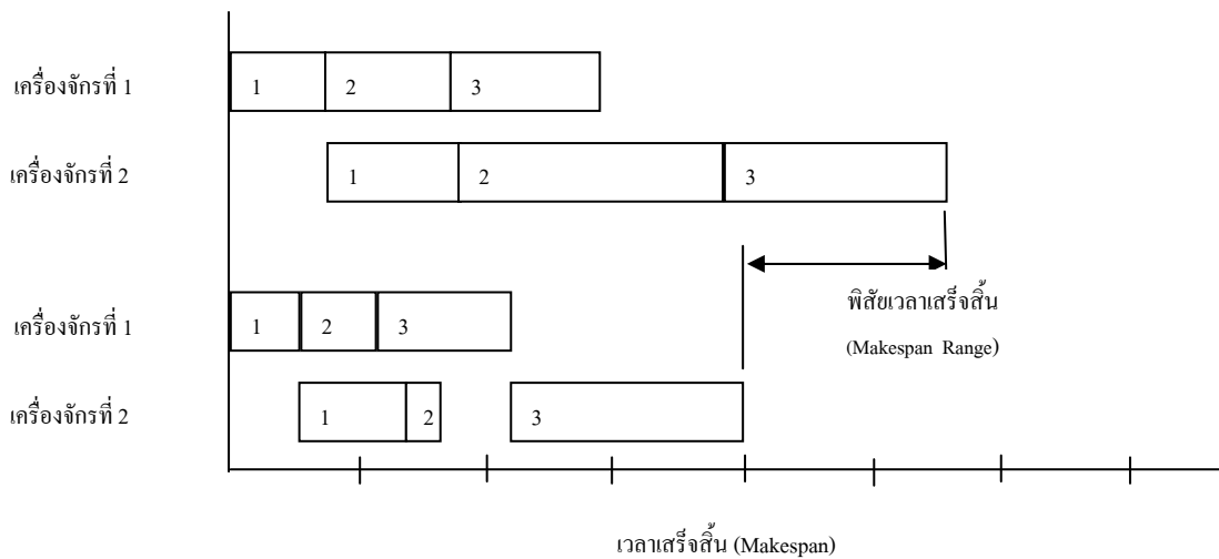
ภาพที่ 6 แสดงพิสัยเวลาเสร็จสิ้นของลำดับงาน 1-2-3
