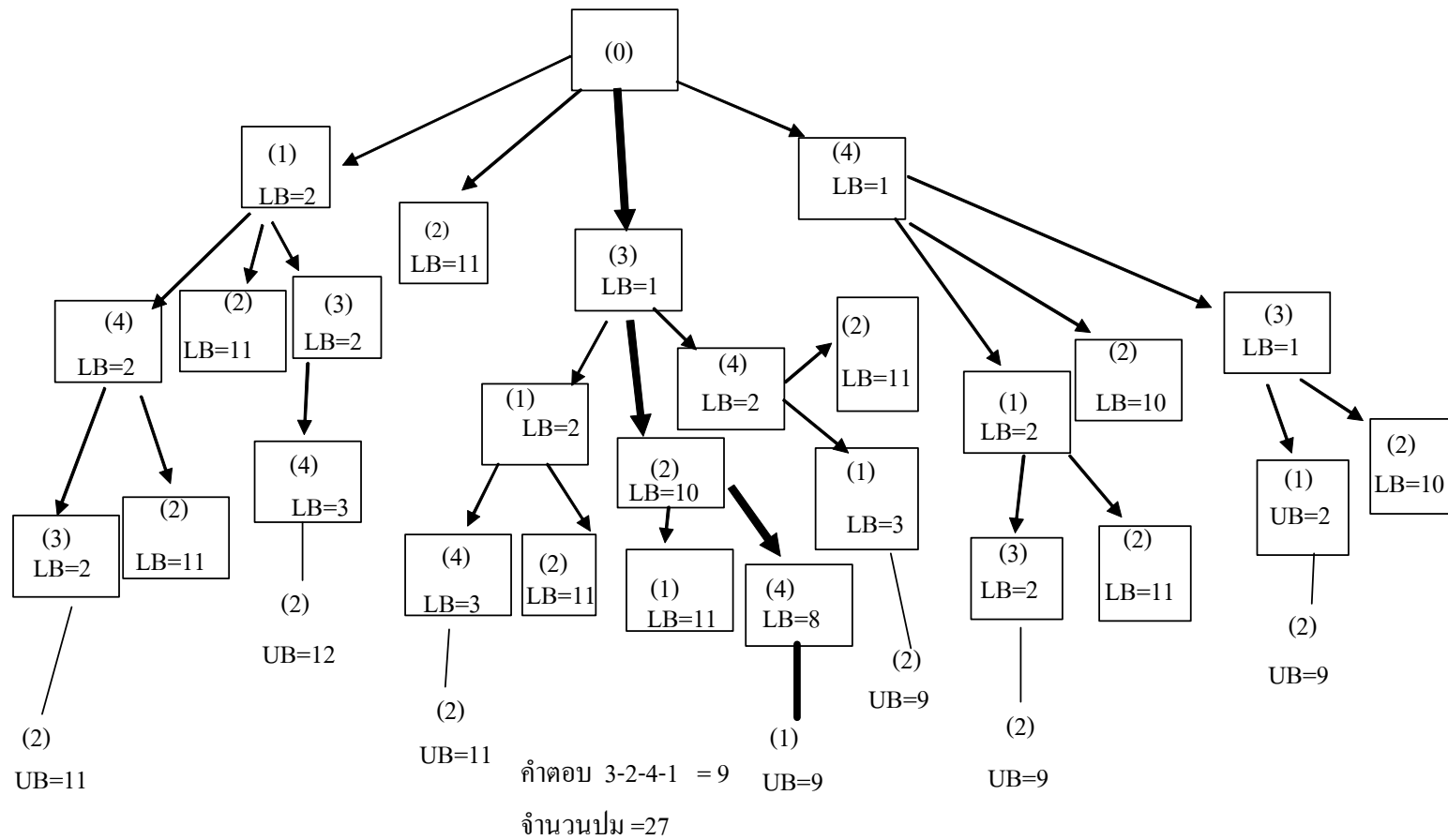
ภาพผนวกที่ ก3 แผนภูมิต้นไม้ของวิธี BB_NUJA กรณี 4 งาน 2 เครื่องจักร
