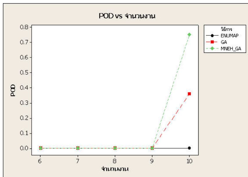
ภาพที่ 21 แสดงความสัมพันธ์ระหว่างเปอร์เซ็นต์ความคลาดเคลื่อนกับจำนวนงานจากคำตอบที่ดีที่สุดของวิธี GA และ MNEH_GA (5 เครื่องจักร)
