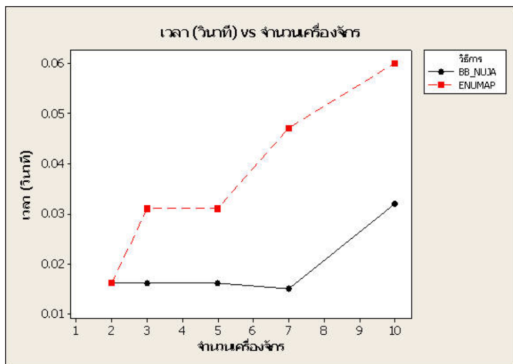
ภาพที่ 16 แสดงความสัมพันธ์ระหว่างเวลาในการคำนวณกับจำนวนเครื่องจักรของวิธีการ BB_NUJA (8 งาน)
