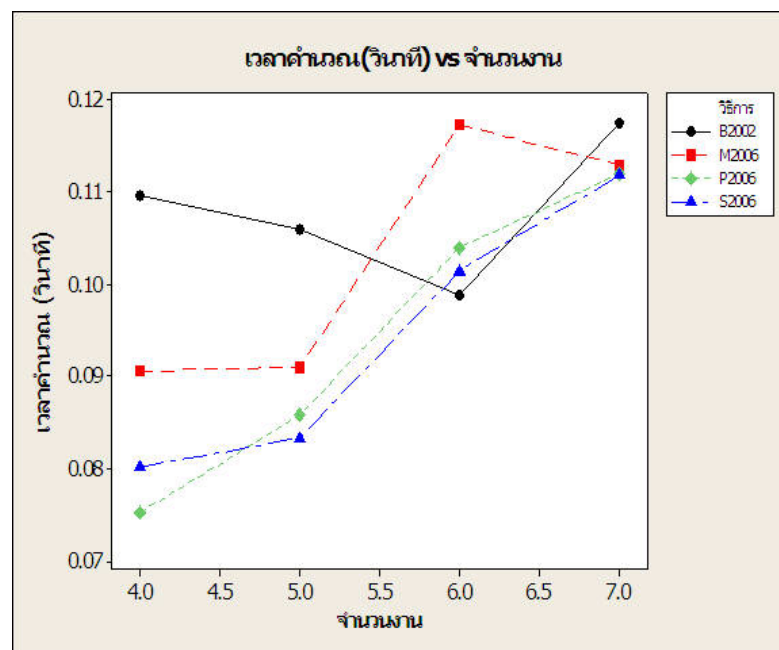
ภาพที่ 35 แสดงความสัมพันธ์ระหว่างเวลาในการคำนวณกับจำนวนงานของวิธีต่างๆ (3 เครื่องจักร)
