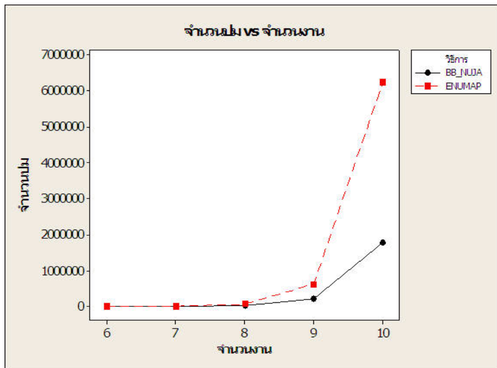
ภาพที่ 13 แสดงความสัมพันธ์ระหว่างจำนวนปมกับจำนวนงานของวิธี BB_NUJA (2 เครื่องจักร)
