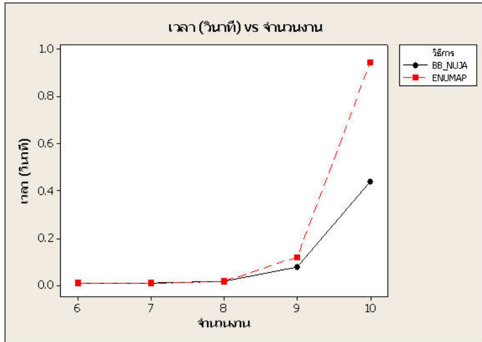
ภาพที่ 15 แสดงความสัมพันธ์ระหว่างจำนวนงานกับเวลาในการคำนวณ (2 เครื่องจักร)
