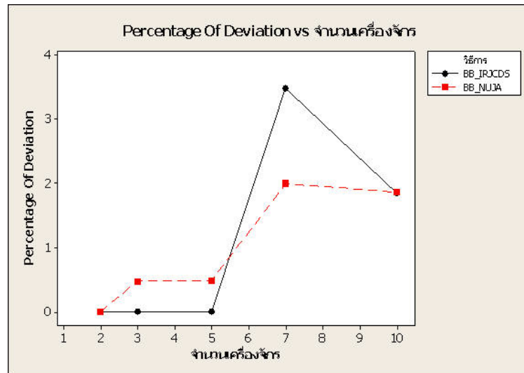
ภาพที่ 17 แสดงความสัมพันธ์ระหว่างเปอร์เซ็นต์ความคลาดเคลื่อนกับจำนวนเครื่องจักรจากคำตอบที่ดีที่สุด (8 งาน)
