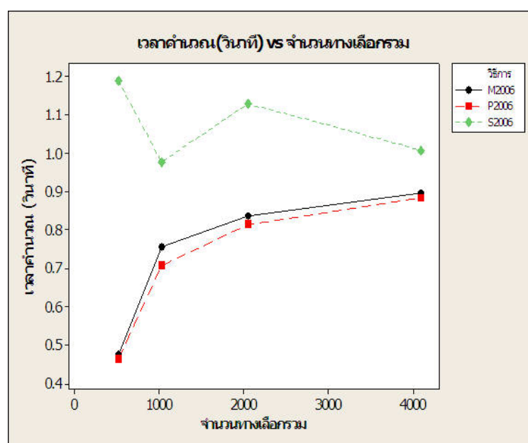
ภาพที่ 43 แสดงความสัมพันธ์ระหว่างเวลาคำนวณกับจำนวนทางเลือกรวมของวิธีต่างๆ (กรณี 12 งาน 5 เครื่องจักร)
