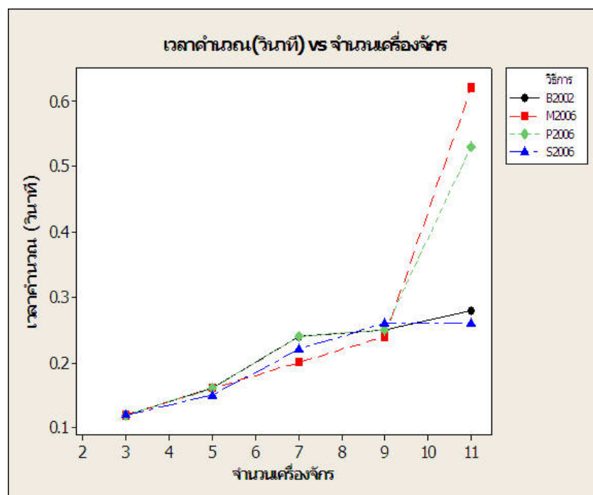
ภาพที่ 37 แสดงความสัมพันธ์ระหว่างเวลาในการคำนวณกับจำนวนเครื่องจักรของวิธีต่างๆ (7 งาน)
