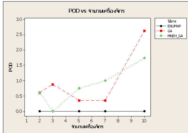
ภาพที่ 22 แสดงความสัมพันธ์ระหว่างเปอร์เซ็นต์ความคลาดเคลื่อนกับจำนวนเครื่องจักร จากคำตอบที่ดีที่สุดของวิธี GA, MNEH_GA และ ENUMAP (10 งาน)
