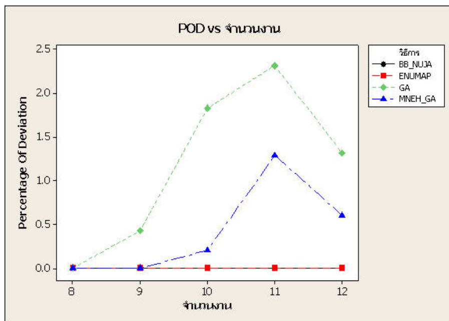
ภาพที่ 24 แสดงความสัมพันธ์ระหว่างเปอร์เซ็นต์ความคลาดเคลื่อนกับจำนวนงานจากคำตอบที่ดีที่สุดของวิธีการต่างๆ (10 เครื่องจักร)
