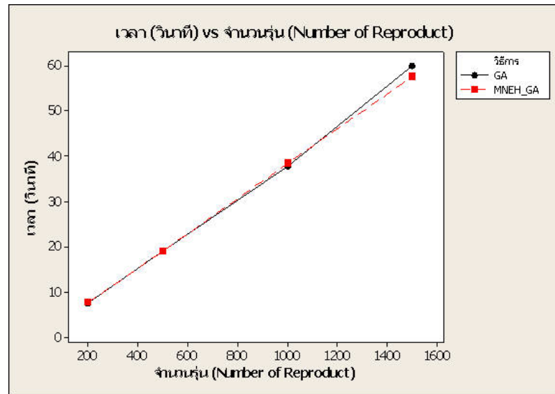
ภาพที่ 30 แสดงความสัมพันธ์ระหว่างเวลาคำนวณกับจำนวนรุ่นของประชากรในวิธี GA (กรณี 18 งาน 12 เครื่องจักร)
