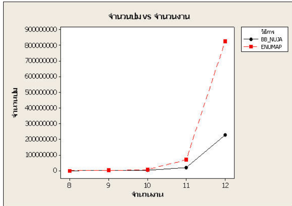
ภาพที่ 25 แสดงความสัมพันธ์ระหว่างจำนวนปมกับจำนวนงานของวิธี BB_NUJA(10 เครื่องจักร)
