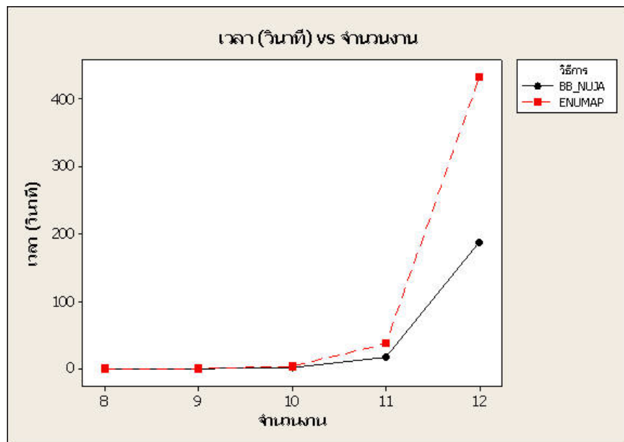
ภาพที่ 26 แสดงความสัมพันธ์ระหว่างเวลาในการคำนวณกับจำนวนงานของวิธี BB_NUJA(10 เครื่องจักร)
