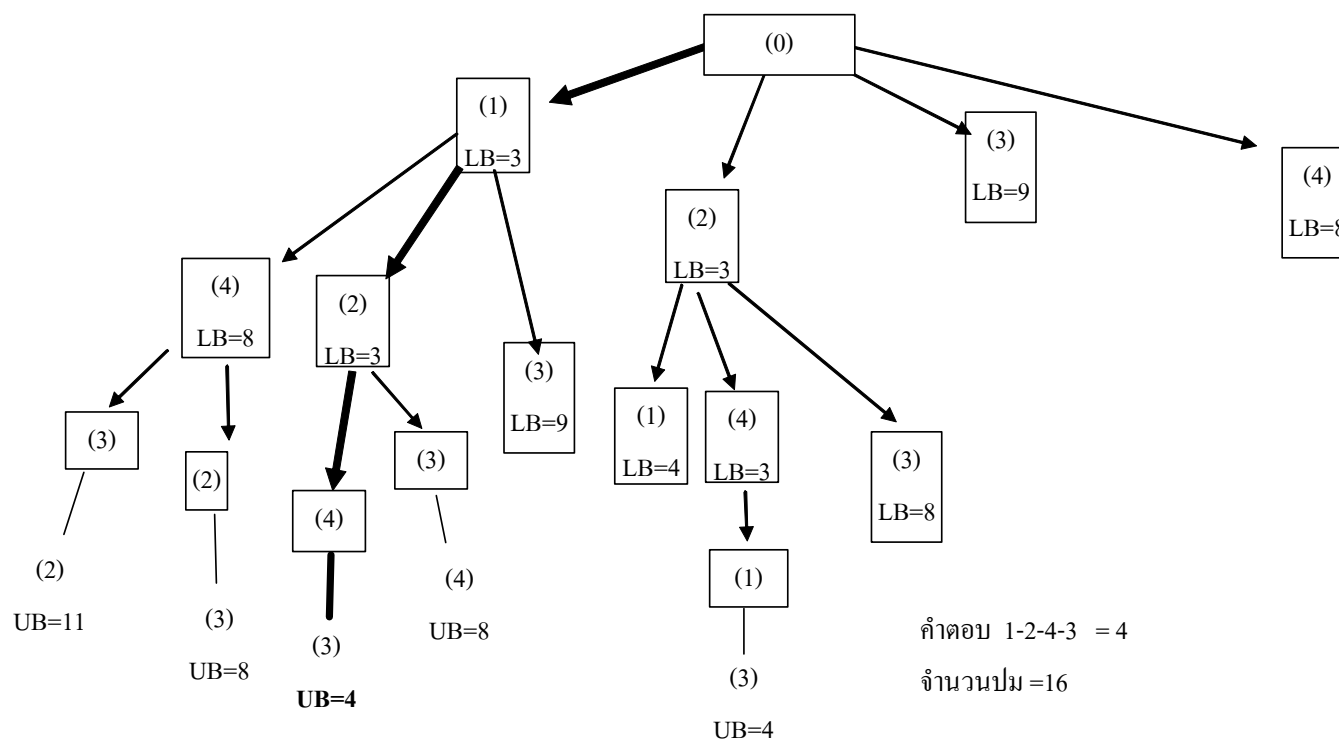
ภาพผนวกที่ ก1 แผนภูมิต้นไม้ของวิธี BB_IRJCDS กรณี 4 งาน 2 เครื่องจักร
