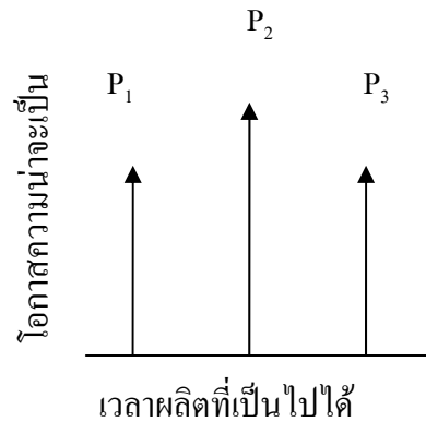
ภาพที่ 3 แสดงเวลาการผลิตไม่แน่นอนและโอกาสความน่าจะเป็น
