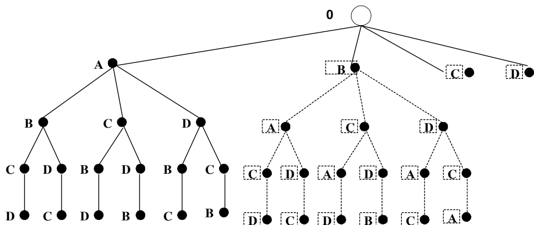
ภาพที่ 7 แสดงการท่องไปในทรีของวิธีการเรียงสับเปลี่ยน กรณีที่มีงาน 4 งาน
