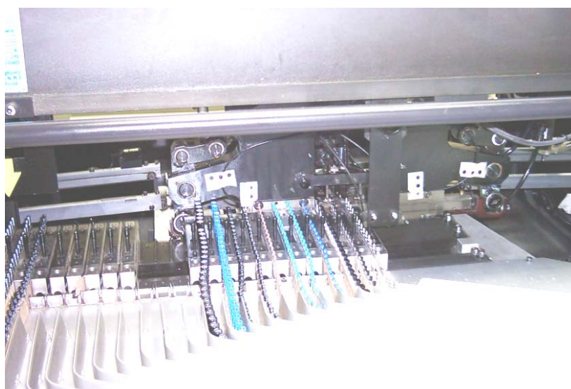
ภาพที่ 49 เครื่องจักรวางอุปกรณ์แบบ Radial Lead
