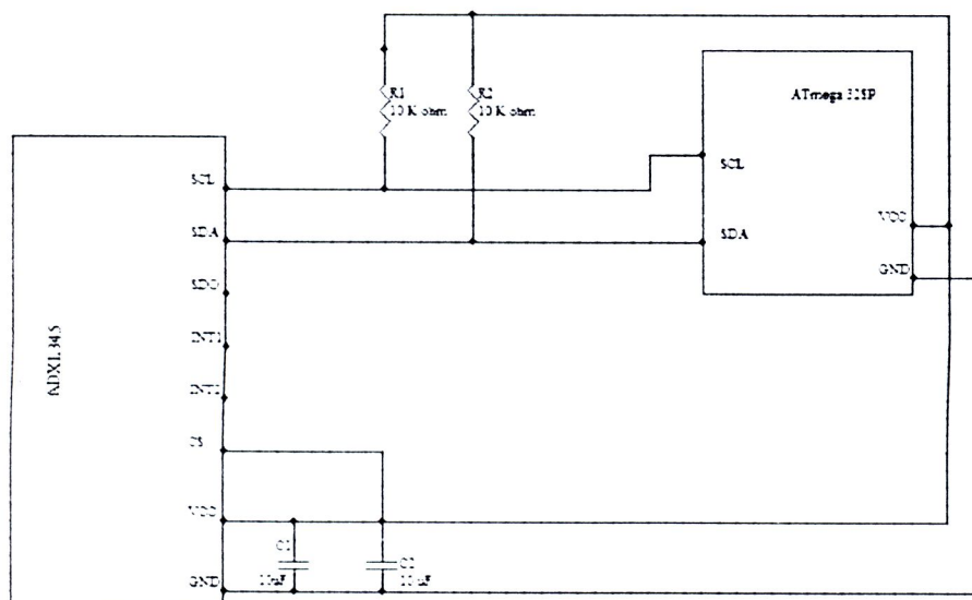
รูปที่ 3.3 การออกแบบการเชื่อมต่อข้อมูลแบบ I2C Bus กับบอร์ดทดลอง Arduino
