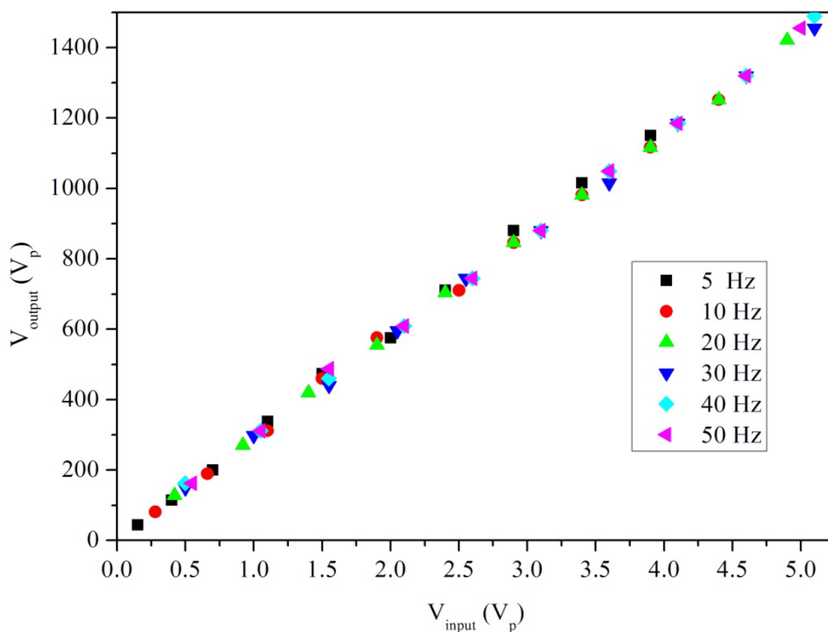
รูปที่ 5.3 กราฟความสัมพันธ์ระหว่างแรงดันไฟฟ้าขาเข้าและแรงดันไฟฟ้าขาออกของหม้อแปลง
