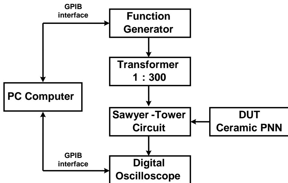
รูปที่ 5.1 แผนภาพการทำงานของระบบเครื่องมือวัดวงวนฮีสเทอรีซิส โดยใช้วงจรซอว์เยอร์-ทาวเวอร์
