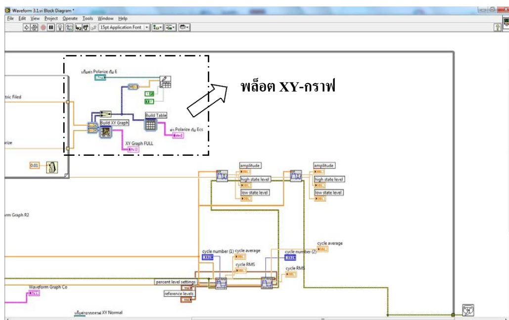
รูปที่ 4.9 ส่วนประกอบภายใน block diagram ที่แสดงส่วนการคำนวณ amplitude
