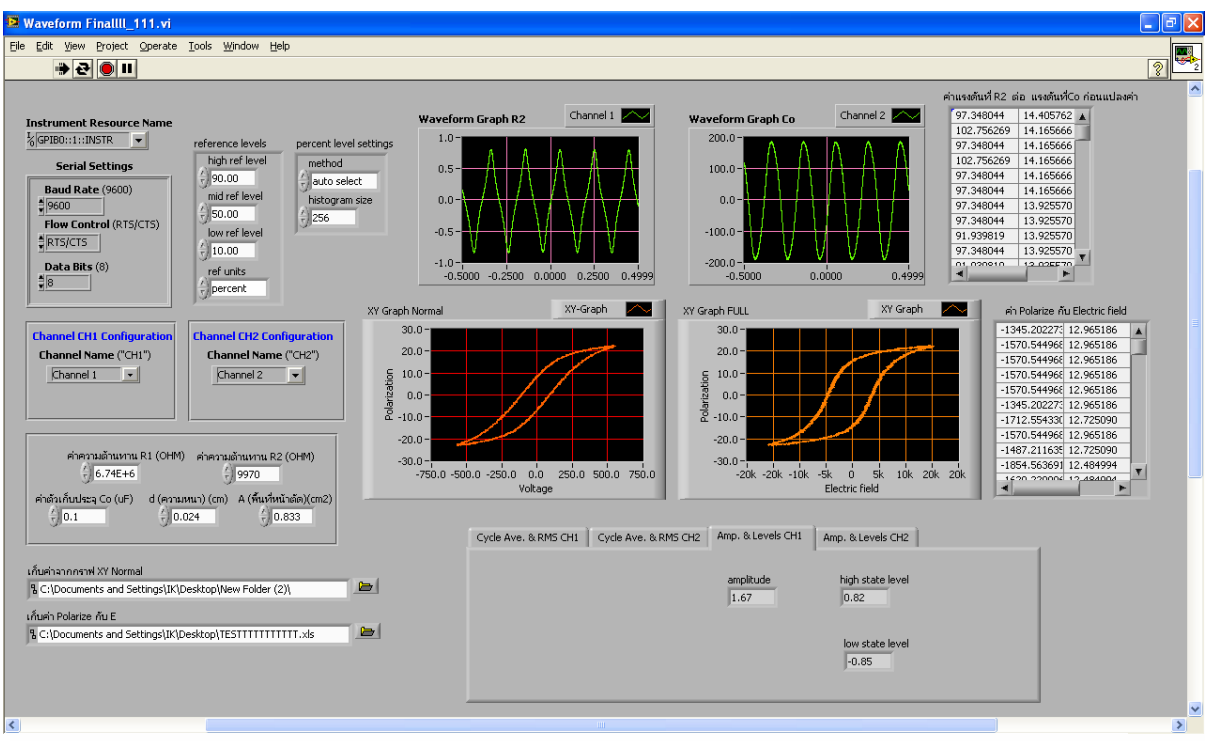
รูปที่ 4.12 Front panel แสดงส่วนการป้อนข้อมูล, การแสดงผลของแรงดันไฟฟ้า และวงวนฮิสทอริซิส
