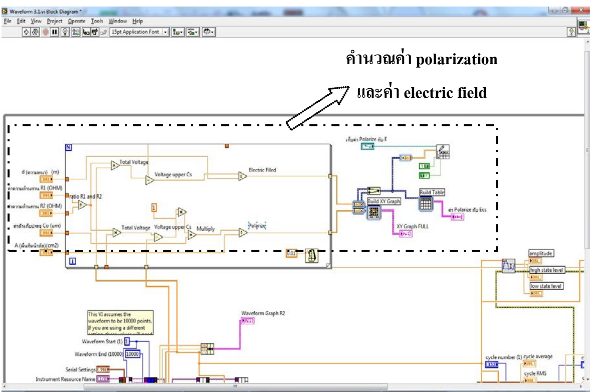
รูปที่ 4.11 ส่วนประกอบภายใน block diagram ที่แสดงส่วนการคำนวณโพลาไรเซชัน และสนามไฟฟ้า
