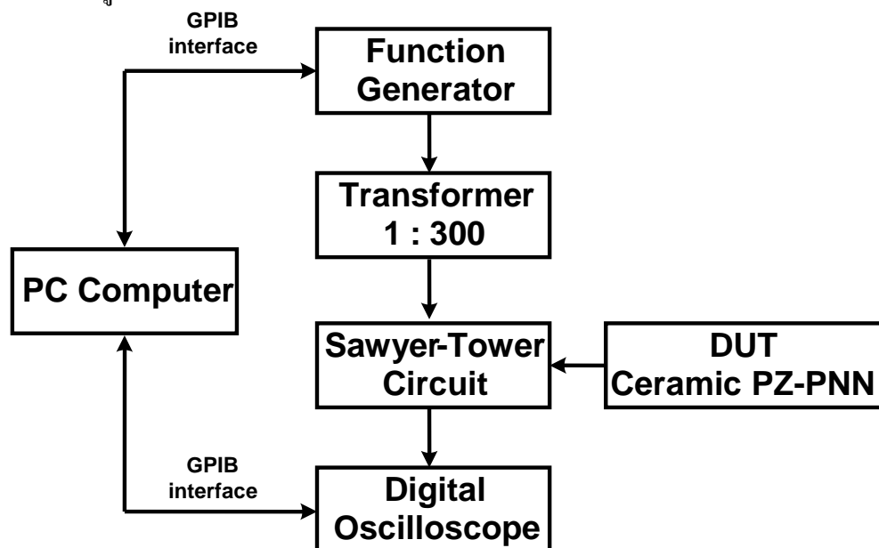
รูปที่ 4.1 แผนภาพการทำงานของระบบเครื่องมือวัดวงวนฮีสเทอรีซิส โดยใช้วงจรซอว์เยอร์-ทาวเวอร์
