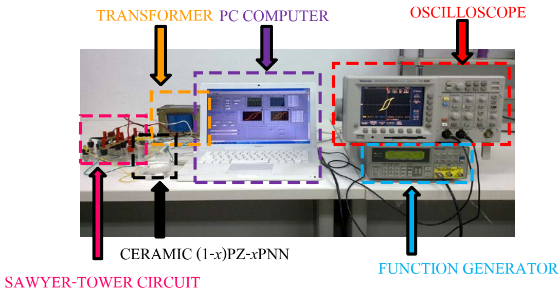
รูปที่ 4.2 ภาพถ่ายของชุดระบบเครื่องมือวัดวงวนฮิสเทอรีซิส
