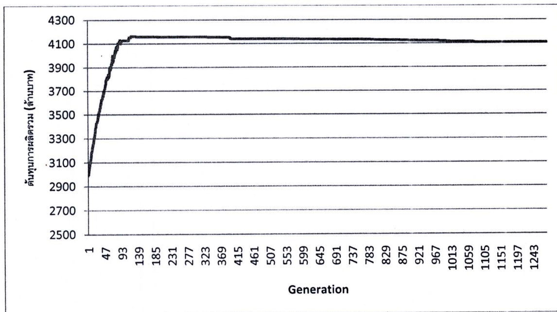
รูปที่ ค.3-3 กราฟแสดงต้นทุนการผลิตไฟฟ้าในแต่ละรอบ
