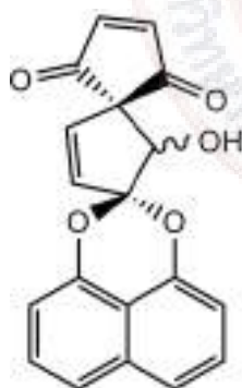
spiropreussione A [8]
