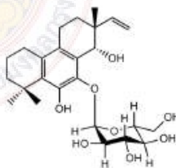
Xyloopimarane [9]
