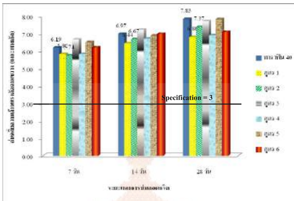
ภาพที่ 4.16 ค่าเฉลี่ยความดัดตามขวางของคอนกรีตบดอัดพาราฟิน ที่ระยะเวลาบ่มต่างๆ
