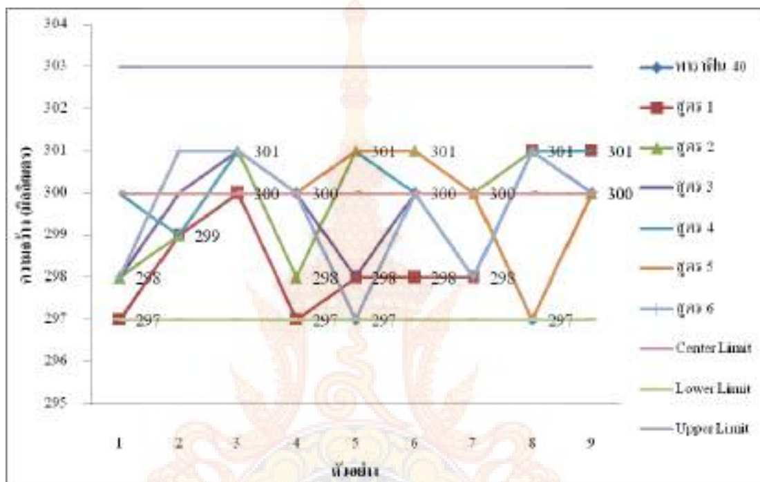
ภาพที่ 4.14 แผนภูมิพิสัยควบคุมมิติด้านความกว้างของคอนกรีตบล็อกพาราฟินผสมเกล็ดและไฟเบอร์กลาส
