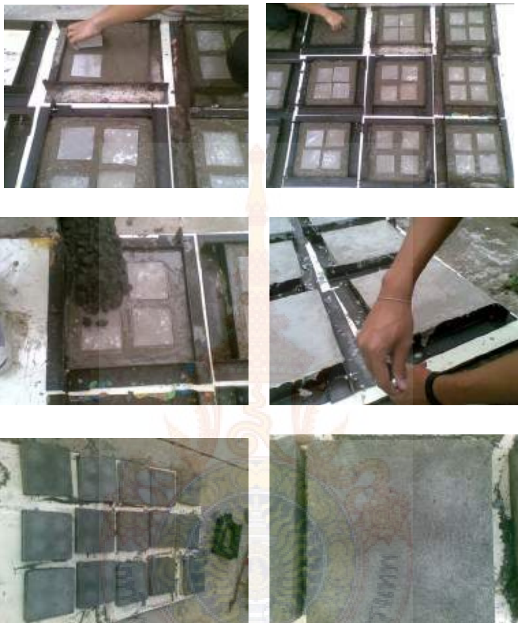
ภาพที่ 3.9 ลักษณะวางแผ่นพาราฟินและการถอดออกจากแบบ
