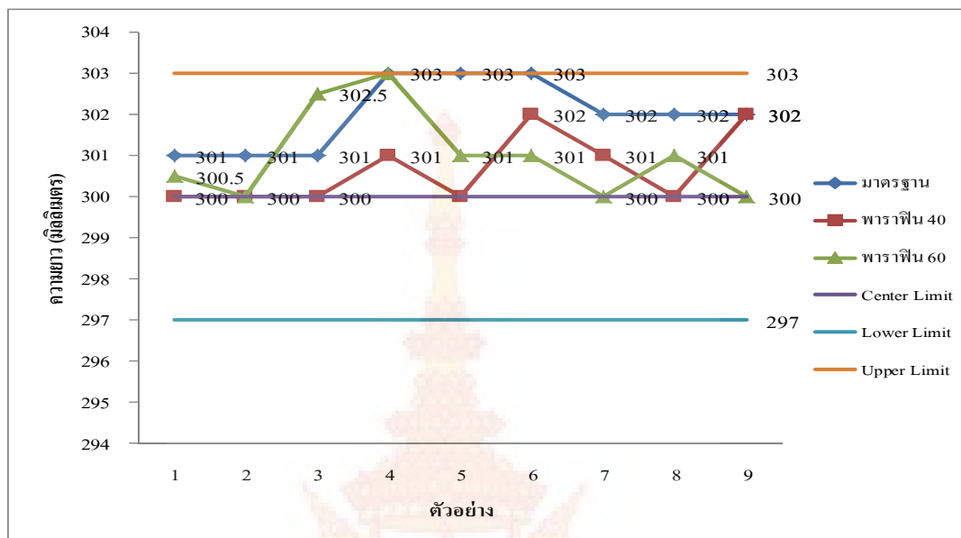
ภาพที่ 4.3 แผนภูมิพิสัยควบคุมมิติด้านความยาวของคอนกรีตบล็อก
