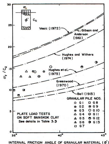
Fig. 32 Bearing capacity of a stone column (Bergado & Lam, 1987)
