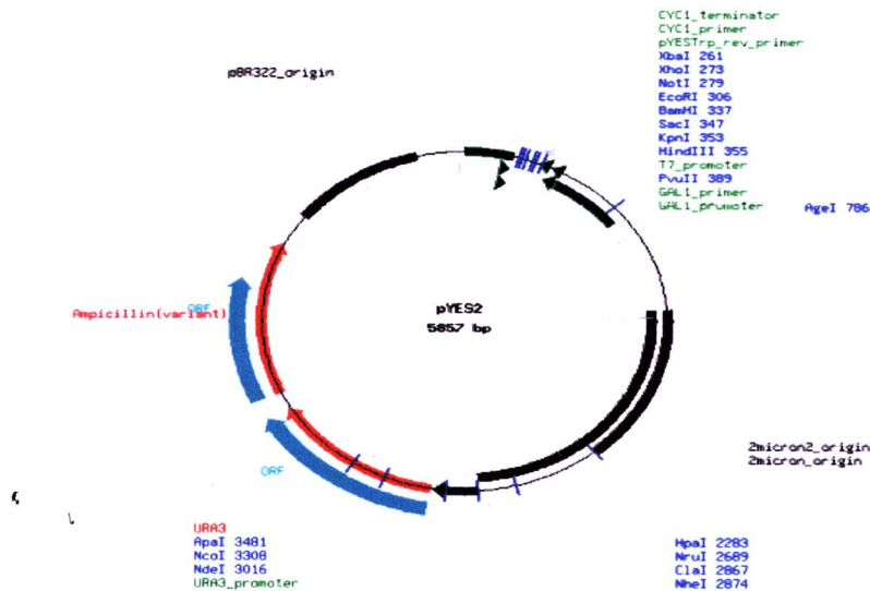
รูปที่ 3.1 แผนที่เรสทริกชันเอนไซม์ของพลาสมิด pYES2
