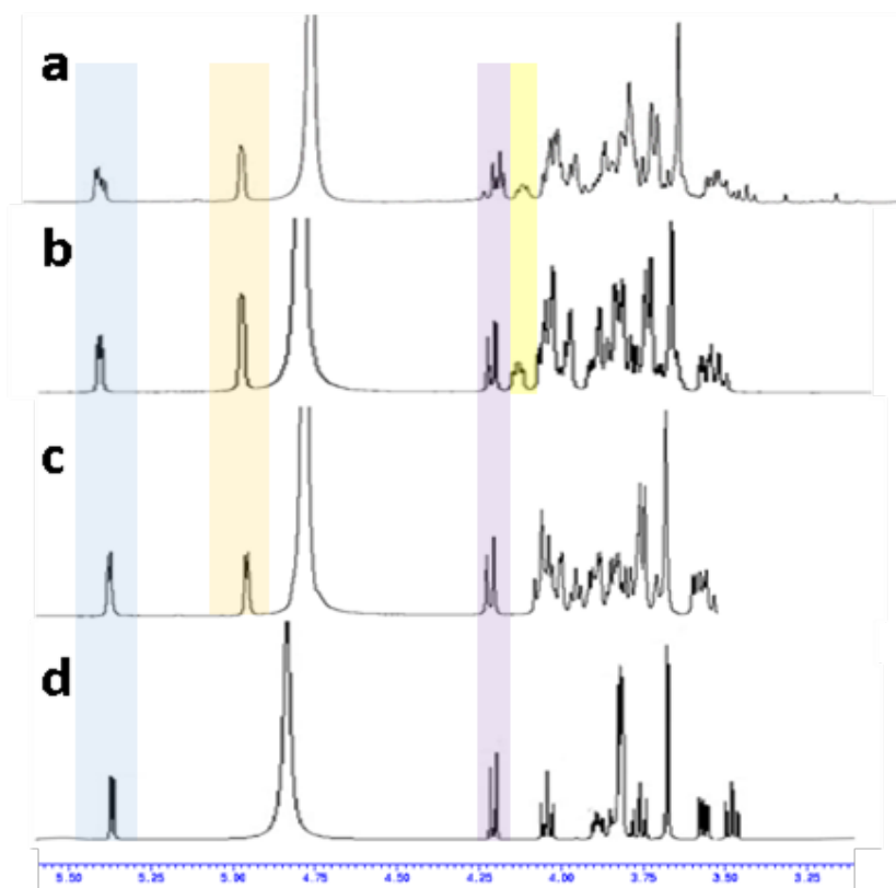
ภาพที่ 2 แสดงการเปรียบเทียบลักษณะพิกของ NMR สเปกตรัม (a) ^1\text{H} -NMR ของสารที่ได้จากกระบวนการตกตะกอน (ทำการละลายสารด้วยตัวทำละลายดีเอมออกไซด์ ( \text{D}_2\text{O} )); (b) ^1\text{H} -NMR ของน้ำตาลสแตคิโอส; (c) ^1\text{H} -NMR ของน้ำตาลราฟิโนส; (d) ^1\text{H} -NMR ของน้ำตาลซูโครส
