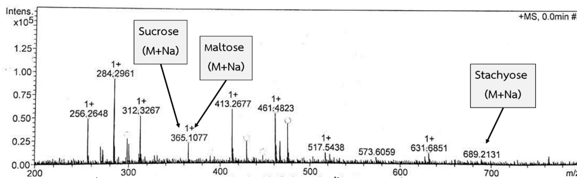
ภาพที่ 3 ผลการวิเคราะห์มวลโมเลกุลของสารตัวอย่างเบื้องต้นด้วยเครื่อง Mass spectrometry
