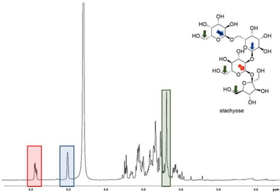
ภาพที่ 1 ลักษณะสเปกตรัม 1 H-NMR ของสารตัวอย่างที่ตกตะกอน (ทำการละลายสารด้วยตัวทำละลายดีวเทอเรียม ออกไซด์ มีสูตรโมเลกุล D 2 O)
