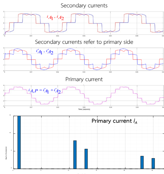
รูปที่ 6 กระแสและสเปกตรัมของ HMT เมื่อจ่ายโหลดชุดที่ 1 และ 3 พร้อมกัน (เลื่อนเฟส 30 องศา)
