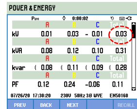
รูปที่ 14 ผลการทดสอบกำลังไฟฟ้าของหม้อแปลงขณะไร้อุปกรณ์ที่แรงดันพิกัด
