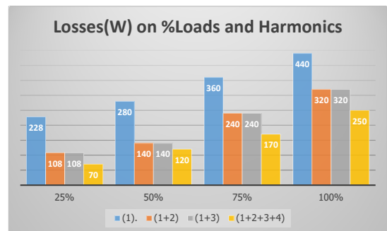
รูปที่ 12 ความสัมพันธ์ระหว่างค่าสูญเสียต่อกระแสฮาร์มอนิกสในแต่ละกรณีและค่าร้อยละของกระแสฟลักซ์
