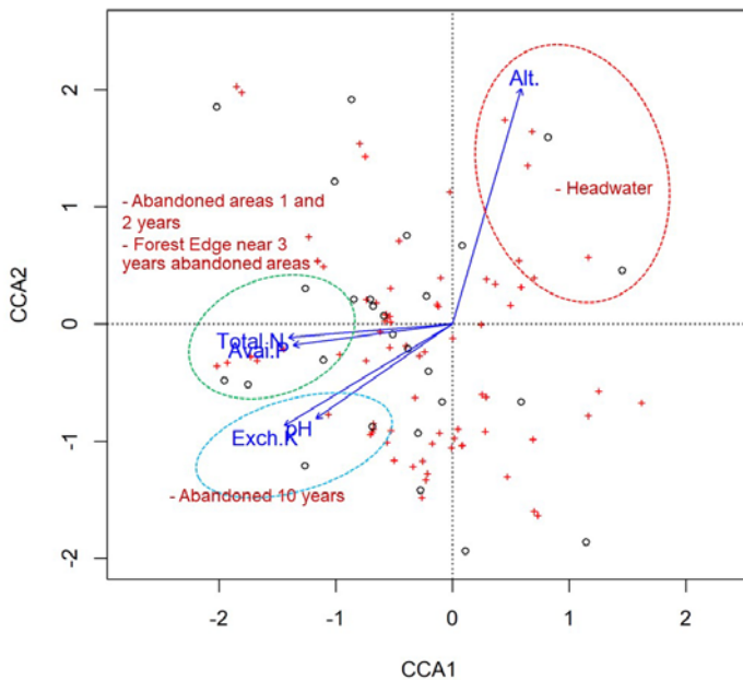
ภาพที่ 3 การจัดอันดับกลุ่มพันธุ์ไม้ด้วยการวิเคราะห์ canonical correspondence analysis (CCA)
