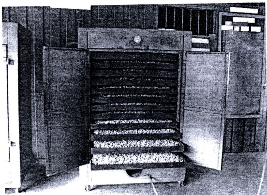
อบเมล็ดมะม่วงหิมพานต์ที่ผ่าแล้ว (ตู้อบที่ใช้แก๊ส)
