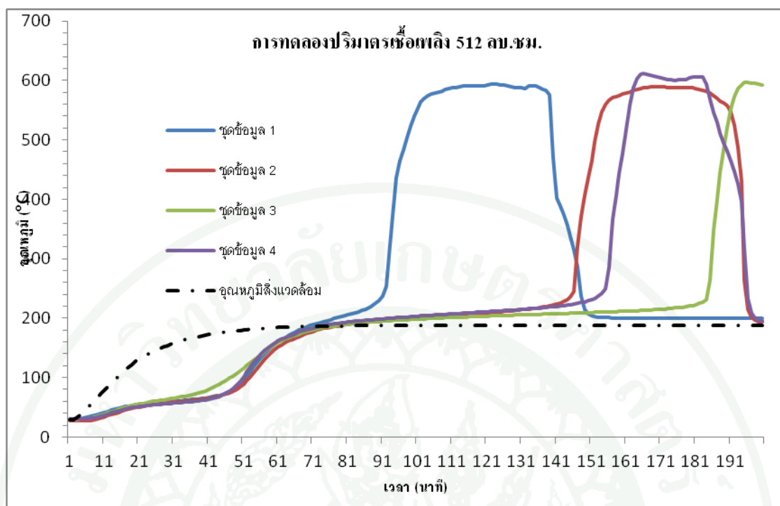
ภาพที่ 18 อุณหภูมิติดไฟของเชื้อเพลิงรูปทรงลูกบาศก์ที่มีสารปนเปื้อนขนาด 512 ลบ.ซม.
