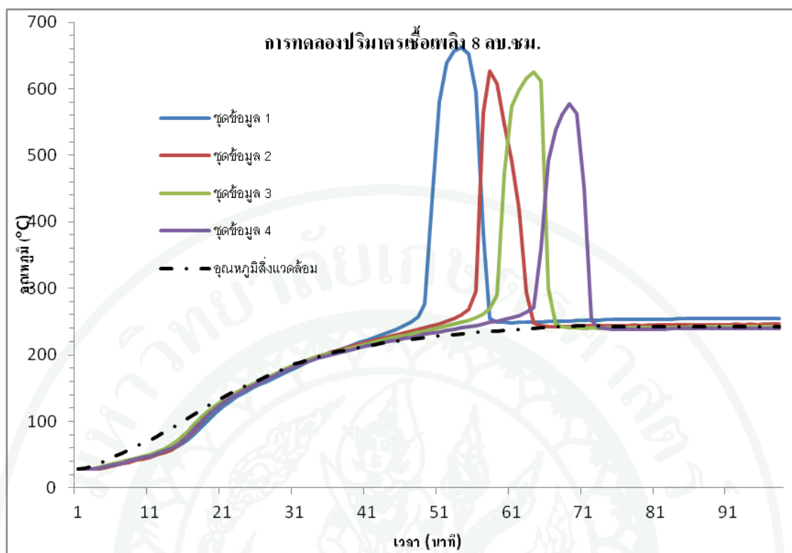
ภาพที่ 16 อุณหภูมิติดไฟของเชื้อเพลิงรูปทรงลูกบาศก์ที่มีสารปนเปื้อนขนาด 8 ลบ.ชม.
