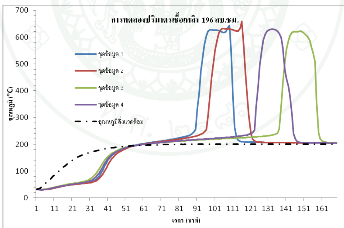
ภาพที่ 19 อุณหภูมิติดไฟของเชื้อเพลิงรูปทรงกระบอกที่มีสารปนเปื้อนขนาด 196 ลบ.ซม.
