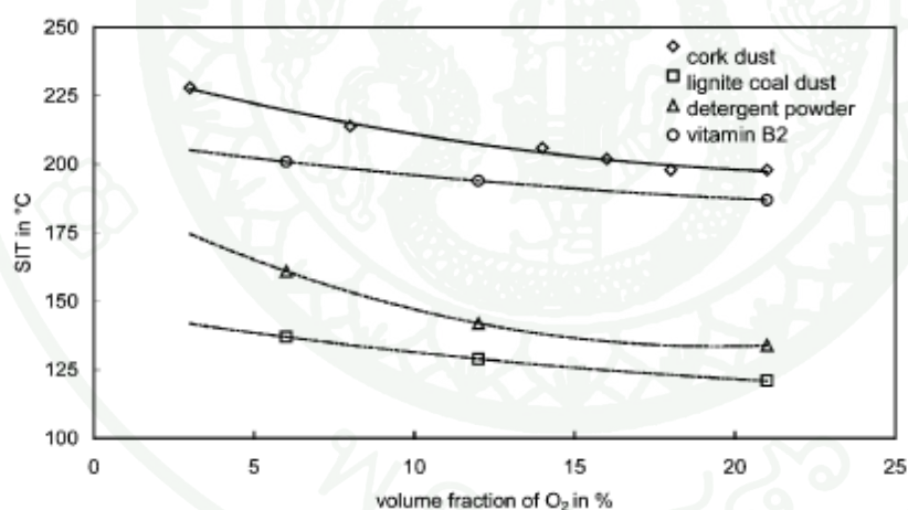
ภาพที่ 6 ความสัมพันธ์ระหว่างอุณหภูมิการจุดติดไฟ (SIT) กับสัดส่วนเปอร์เซ็นต์โดยปริมาตรของออกซิเจน
