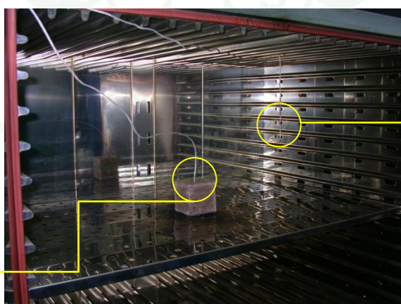
ภาพที่ 13 ตัวอย่างการจัดวางเชื้อเพลิงทดสอบและเทอร์มอคัปเปิล
