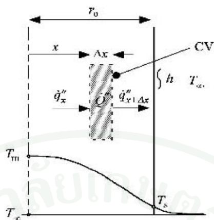
ภาพที่ 3 แบบจำลองปริมาตรควบคุมการสร้างความร้อนและการถ่ายโอนความร้อน
