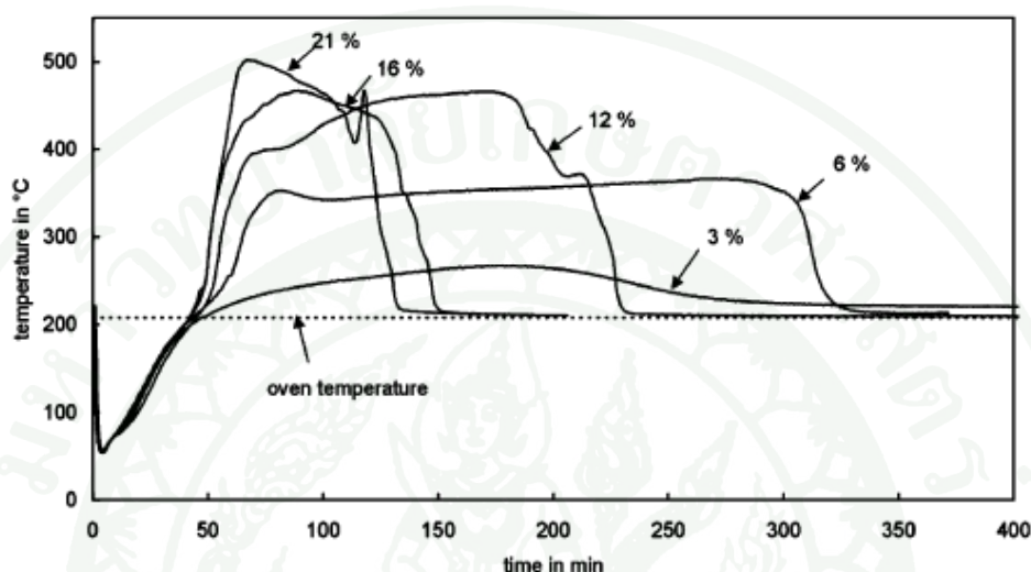
ภาพที่ 7 ความสัมพันธ์ระหว่างอุณหภูมิการลุกติดไฟเปรียบเทียบกับเวลาที่สัดส่วนเปอร์เซ็นต์ออกซิเจนต่าง ๆ
