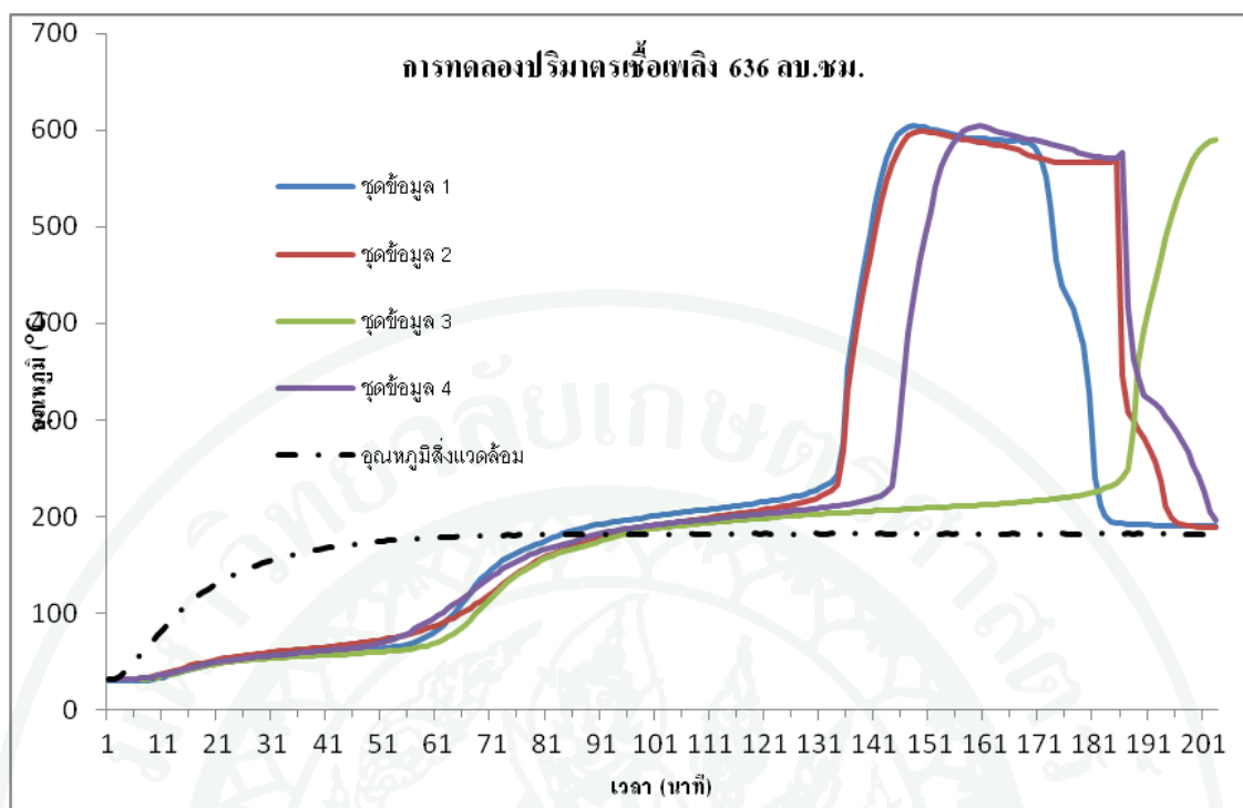
ภาพที่ 20 อุณหภูมิติดไฟของเชื้อเพลิงรูปทรงกระบอกที่มีสารปนเปื้อนขนาด 636 ลบ.ซม.
