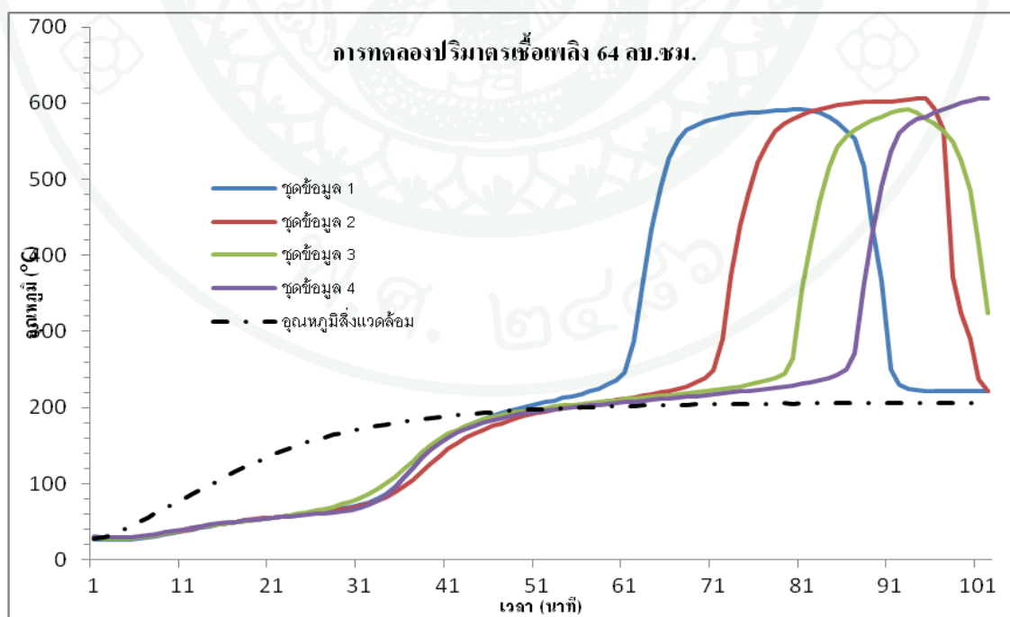
ภาพที่ 17 อุณหภูมิติดไฟของเชื้อเพลิงรูปทรงลูกบาศก์ที่มีสารปนเปื้อนขนาด 64 ลบ.ชม.
