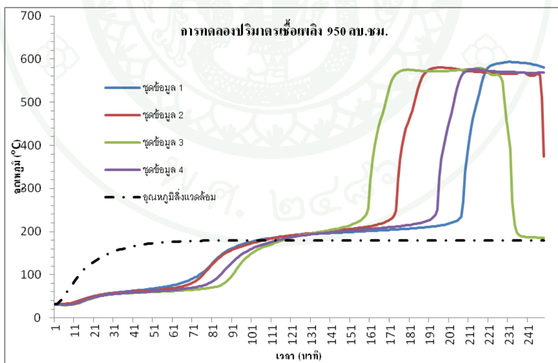
ภาพที่ 21 อุณหภูมิติดไฟของเชื้อเพลิงรูปทรงกระบอกที่มีสารปนเปื้อนขนาด 950 ลบ.ซม.
