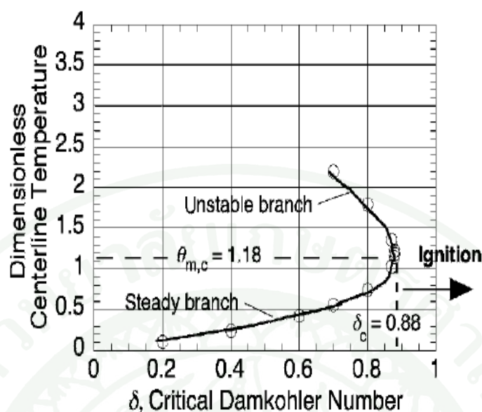
ภาพที่ 4 ความสัมพันธ์ระหว่างอุณหภูมิไร้หน่วยที่ศูนย์กลางกับค่าวิกฤตแดมโคลของวัสดุแผ่นบาง
