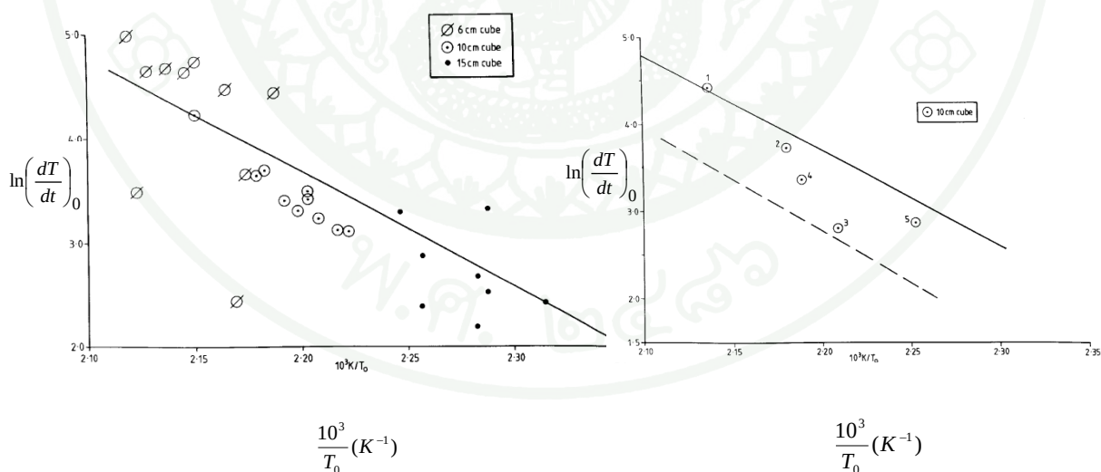
ภาพที่ 5 ความสัมพันธ์ระหว่าง \ln\left(\frac{dT}{dt}\right)_0 กับ \frac{10^3}{T_0} (K^{-1}) ของเชื้อเพลิงที่มีการผึ่งอากาศที่ต่างกัน
