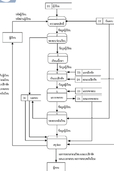
ภาพที่ 6 แผนภาพการไหลของข้อมูล (DFD level 0) ของระบบ
