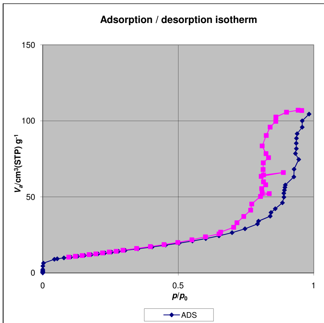
รูปที่ ข.3 Adsorption/desorption isotherm ของวัสดุที่สังเคราะห์ได้ผ่านการให้ความร้อนที่อุณหภูมิ 400 °C
