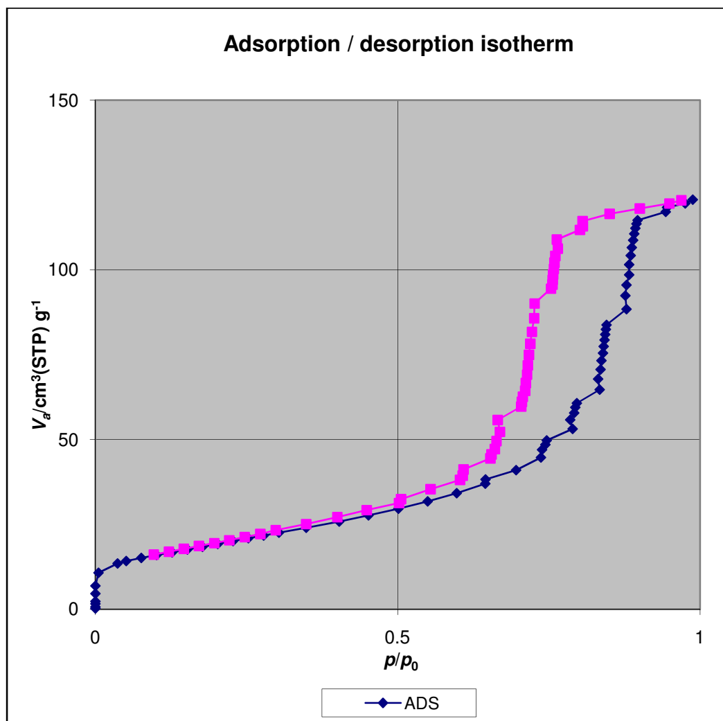
รูปที่ ข.4 Adsorption/desorption isotherm ของวัสดุที่สังเคราะห์ได้ผ่านการให้ความร้อนที่อุณหภูมิ 500 °C
