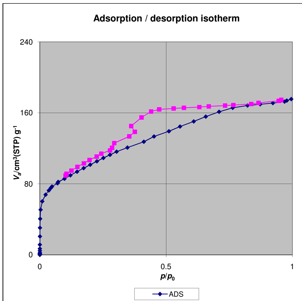
รูปที่ ข.1 Adsorption/desorption isotherm ของวัสดุที่สังเคราะห์ได้
