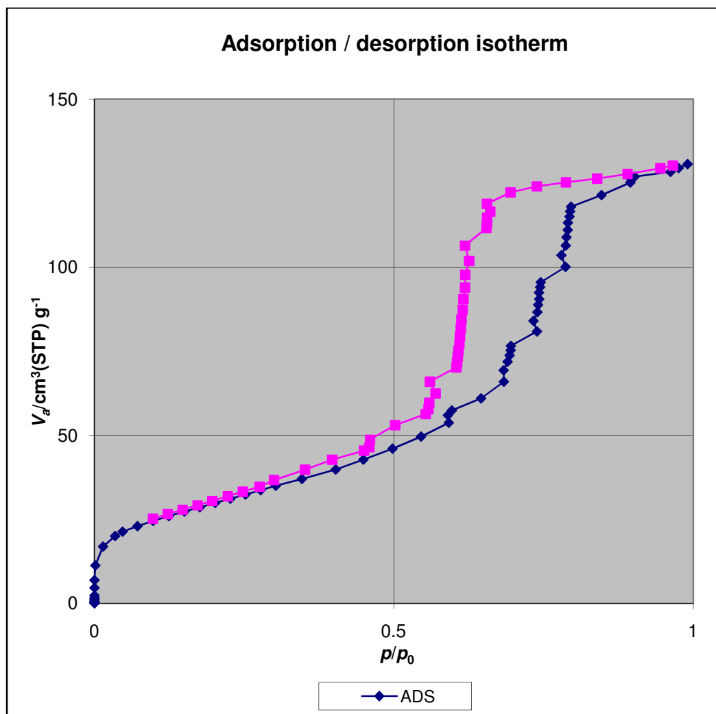
รูปที่ ข.2 Adsorption/desorption isotherm ของวัสดุที่สังเคราะห์ได้ผ่านการให้ความร้อนที่อุณหภูมิ 300 °C
