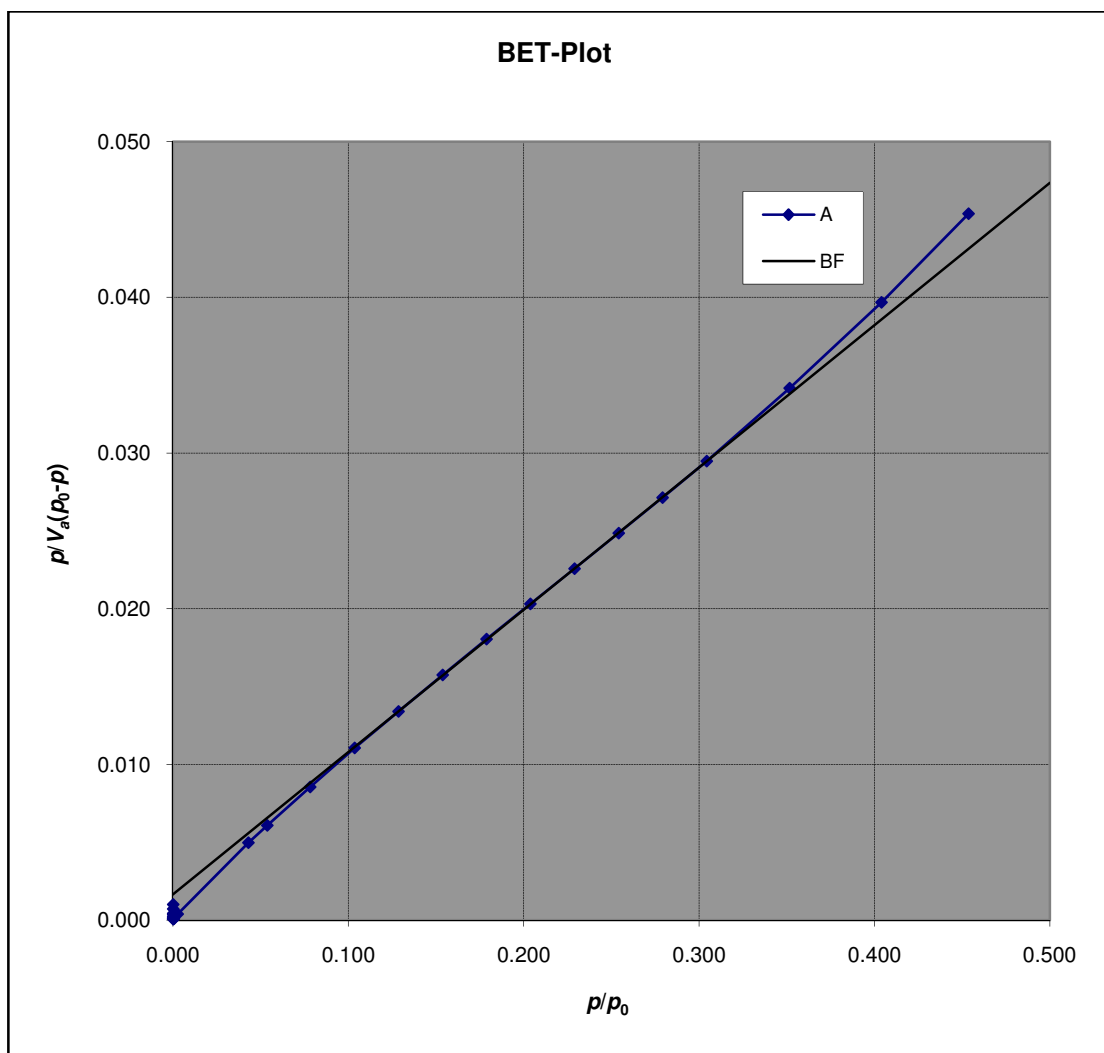
รูปที่ ก.4 พื้นที่ผิวจำเพาะของวัสดุที่สังเคราะห์ได้ผ่านการให้ความร้อนที่อุณหภูมิ 500 °C
