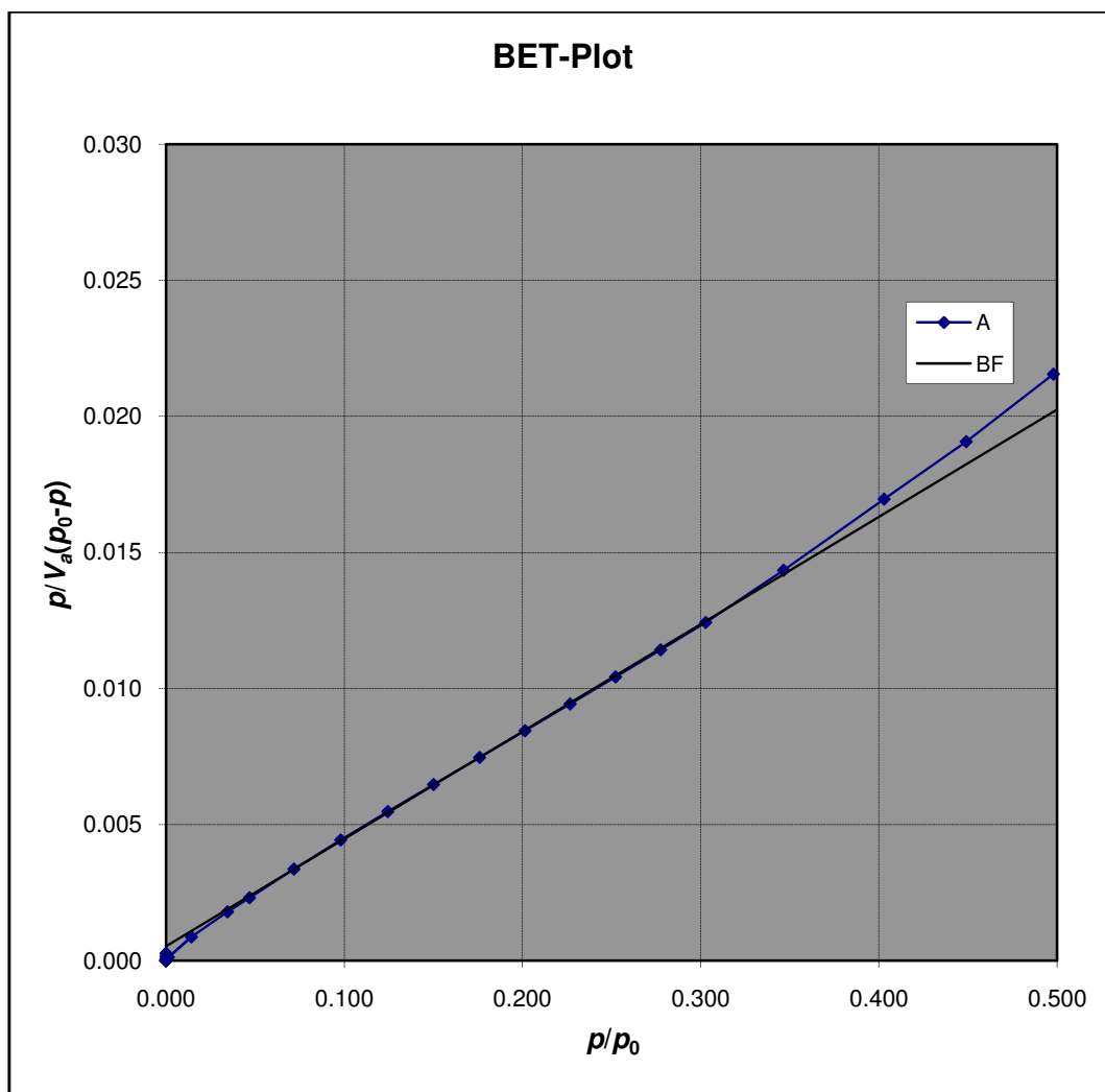
รูปที่ ก.2 พื้นที่ผิวจำเพาะของวัสดุที่สังเคราะห์ได้ผ่านการให้ความร้อนที่อุณหภูมิ 300 °C
