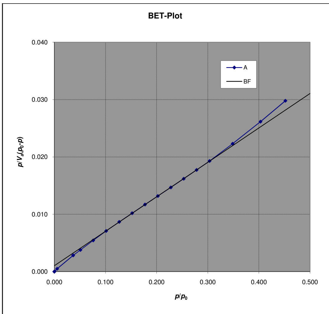
รูปที่ ก.3 พื้นที่ผิวจำเพาะของวัสดุที่สังเคราะห์ได้ผ่านการให้ความร้อนที่อุณหภูมิ 400 °C
