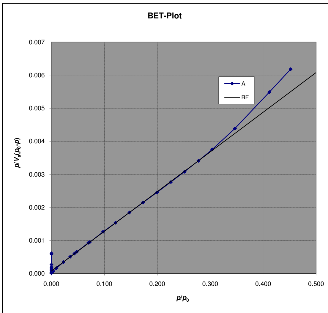
รูปที่ ก.1 พื้นที่ผิวจำเพาะของวัสดุที่สังเคราะห์ได้
