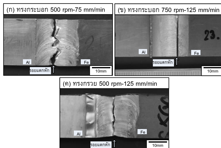
รูปที่ 4.10 รอยแตกหักของชิ้นทดสอบแรงดึง
