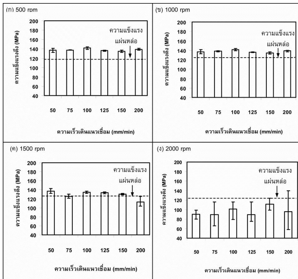
รูปที่ 4.6 ความสัมพันธ์ระหว่างความเร็วรอบ ความเร็วเดิน และความแข็งแรงดึงของแนวเชื่อม
