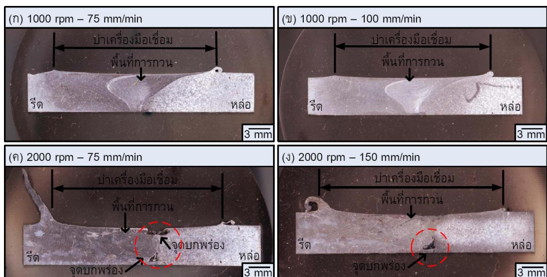
รูปที่ 4.5 โครงสร้างมหภาคของรอยเชื่อมที่สภาวะการเชื่อมต่างๆ
