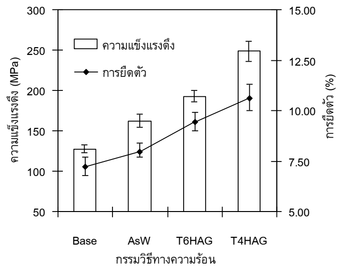
รูปที่ 4.3 ความสัมพันธ์ระหว่างความแข็งแรงดึง ร้อยละการยืดตัว และการอบคืนไฟแบบต่างๆ ของชิ้นงานที่ผ่านการบ่มแข็งธรรมชาติ
