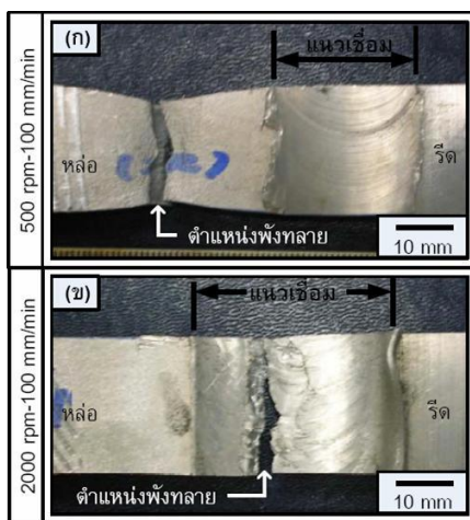
รูปที่ 4.7 ตำแหน่งการพังทลายของชิ้นทดสอบแรงดึง
