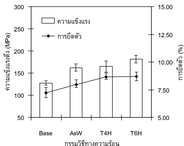
รูปที่ 4.1 ความสัมพันธ์ระหว่างความแข็งแรงดึง ร้อยละการยืดตัว และการอบคืนไฟแบบต่างๆ ของชิ้นงานที่ไม่ผ่านการบ่มแข็งธรรมชาติ
