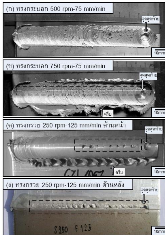
รูปที่ 4.8 ผิวหน้าและความสมบูรณ์ของแนวเชื่อม
