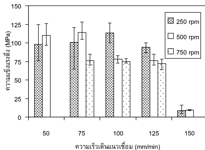
รูปที่ 4.9 ความสัมพันธ์ระหว่างความเร็วเดินแนวเชื่อม ความเร็วรอบ และความแข็งแรงดึงของรอยเชื่อมที่เชื่อมด้วยตัวกวนทรงกระบอ
