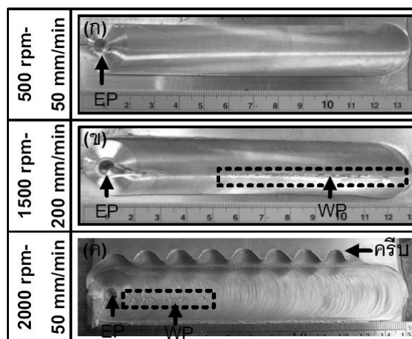
รูปที่ 4.4 ผิวหน้าแนวเชื่อมที่สภาวะการเชื่อมบางตัว
