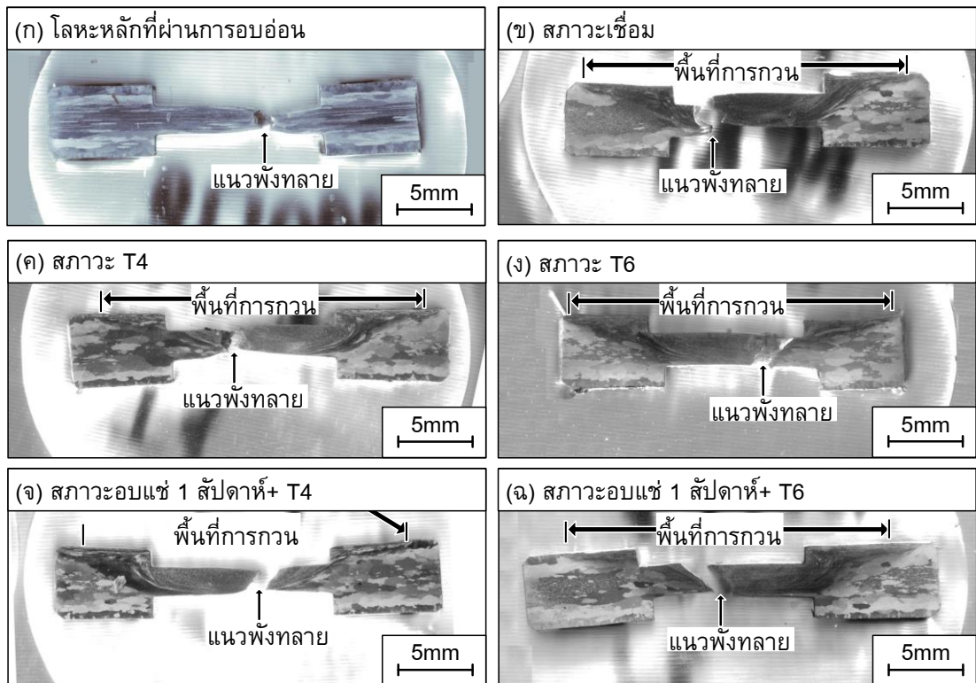
รูปที่ 4.2 ตำแหน่งการพังทลายของชิ้นทดสอบความแข็งแรงดึง
