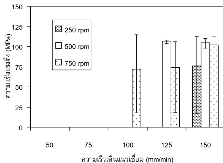
รูปที่ 4.11 ความสัมพันธ์ระหว่างความเร็วเดินแนวเชื่อม ความเร็วรอบ และความแข็งแรงดึงของรอยเชื่อมที่เชื่อมด้วยตัวกวนทรงกรวย
