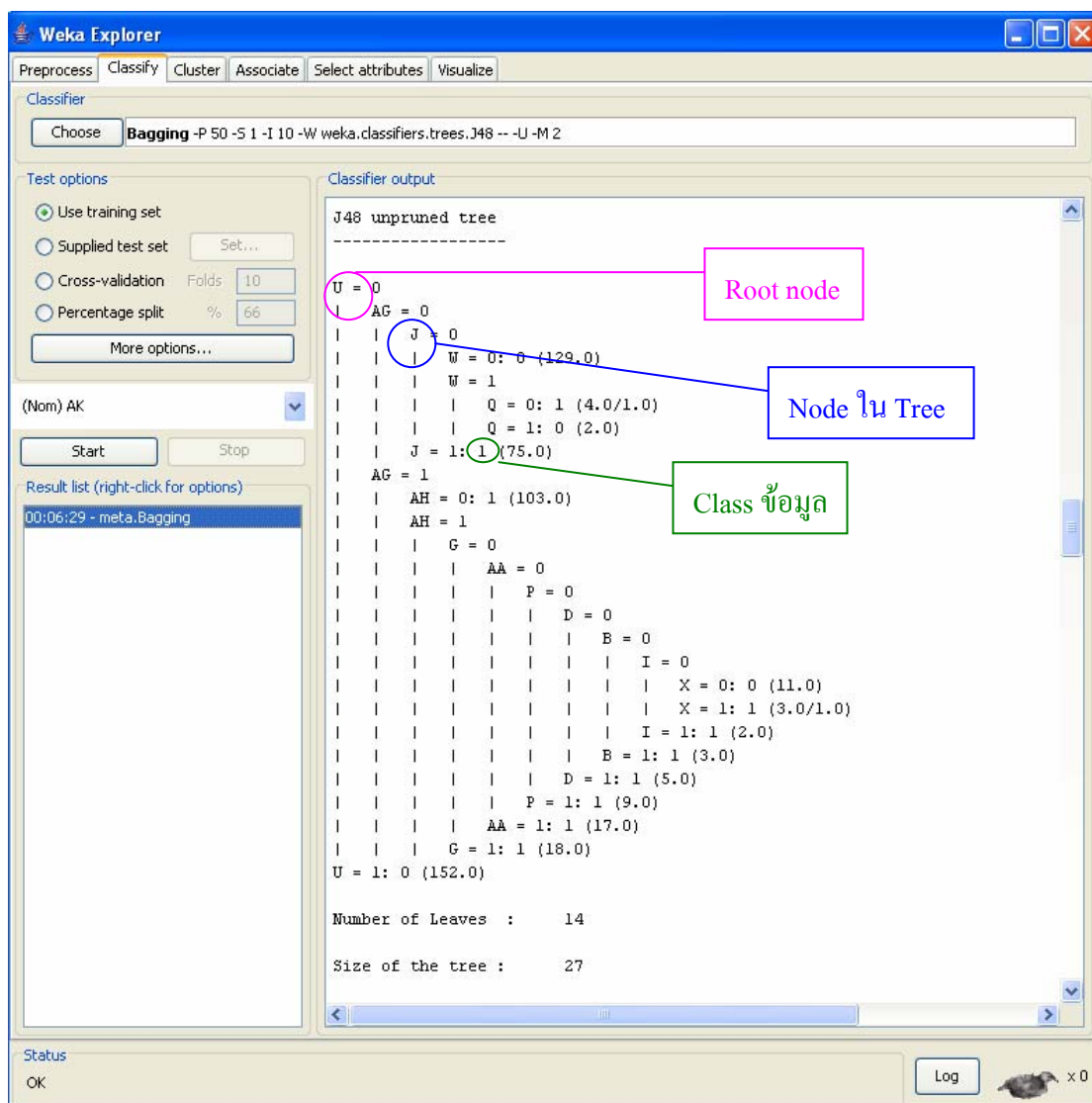
ภาพที่ 18 ตัวอย่างต้นไม้ตัดสินใจโดยใช้วิธีการแบ่งกิ่งของอัลกอริทึม J48 (C4.5) ในโปรแกรม Weka
