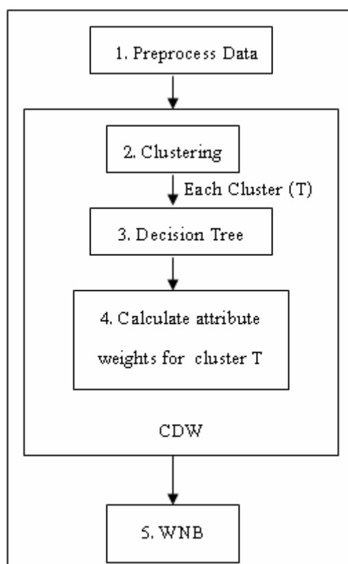
ภาพที่ 13 แสดงลำดับการทำงานของอัลกอริทึมคำนวณค่าน้ำหนักคุณลักษณะด้วยวิธีการจัดกลุ่มและต้นไม้ตัดสินใจ (CDW)
