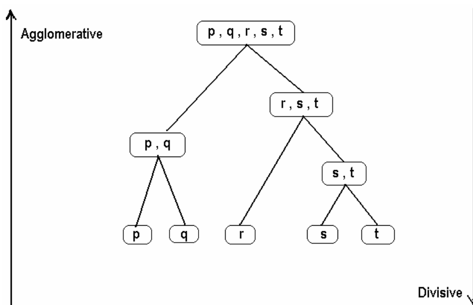
ภาพที่ 6 แสดงการจัดกลุ่มข้อมูลแบบลำดับชั้น
