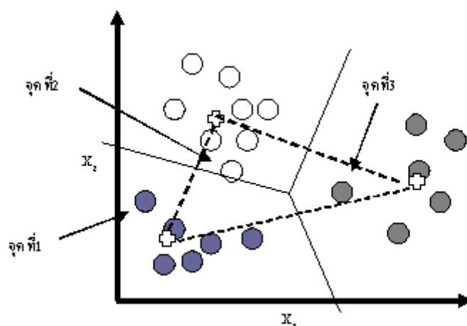
ภาพที่ 4 ภาพแสดงการจัดกลุ่มข้อมูลแบบแบ่งส่วน ที่มา : Jain et al. (1999)
