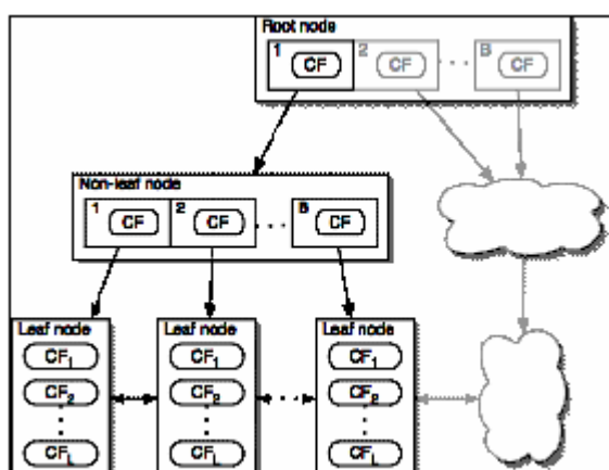
ภาพที่ 7 ลักษณะของ Clustering Feature Tree (CF-Tree)
