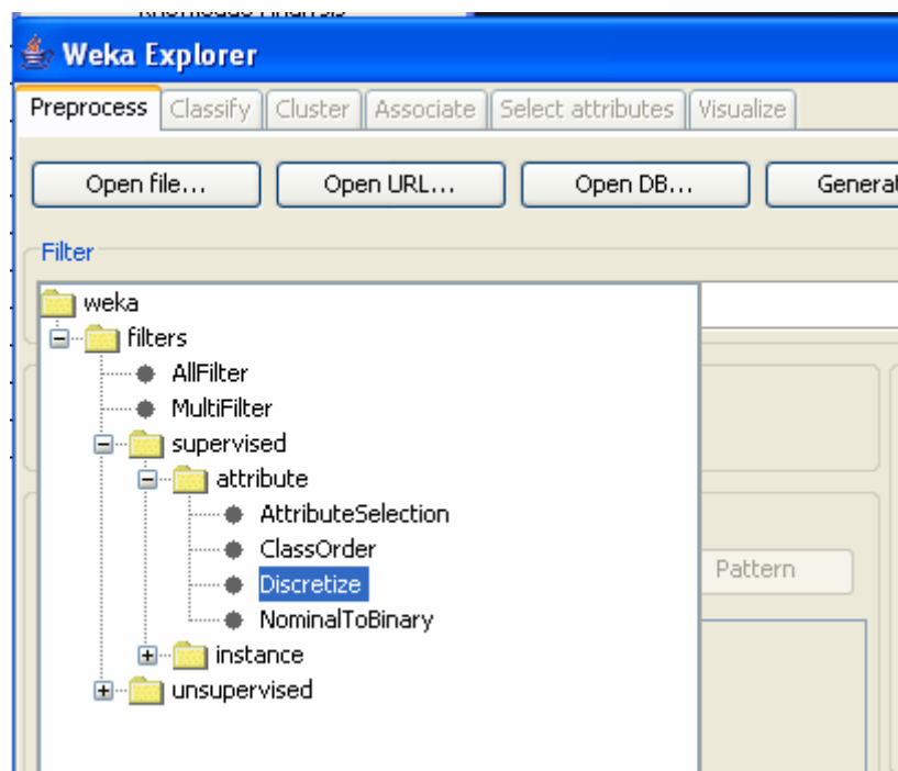
ภาพที่ 14 ตัวอย่างโปรแกรม Weka ในส่วนของการแปลงข้อมูลให้เป็นค่าที่ไม่ต่อเนื่อง (Discretize)
