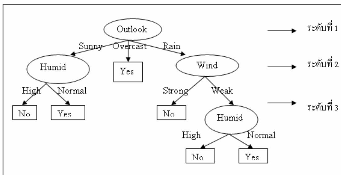
ภาพที่ 10 แสดงตัวอย่างต้นไม้ตัดสินใจสำหรับพิจารณาค่าน้ำหนักของคุณลักษณะข้อมูล ที่มา : Mitchell (1997)
