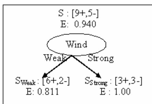
ภาพที่ 2 แสดงโหนดคุณลักษณะ Wind เพื่อหาอัตราส่วนเกน ที่มา : Mitchell, 1997
