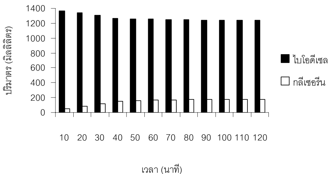
รูป 5.3 แสดงการแยกชั้นระหว่างไบโอดีเซลกับกลีเซอริน
