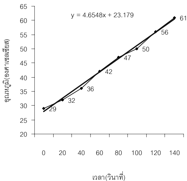
รูป 5.3 แสดงความสัมพันธ์ระหว่างการเพิ่มอุณหภูมิกับระยะเวลา
