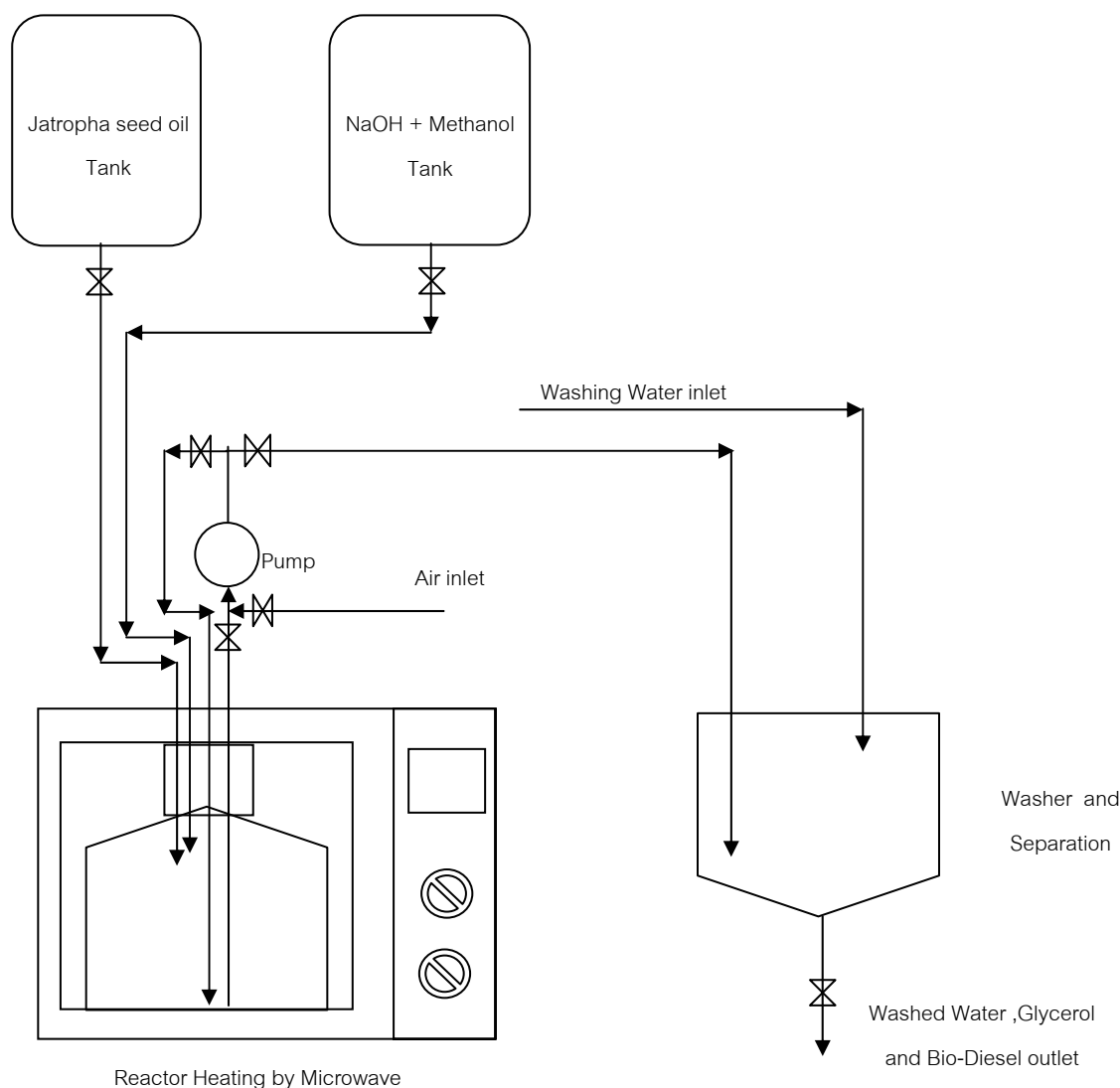
รูป 5.2 แสดงผังการทำงานของเครื่องผลิตไบโอดีเซลจากน้ำมันสบู่ดำโดยกระบวนการทรานส์เอสเทอริฟิเคชัน และให้ความร้อนด้วยคลื่นไมโครเวฟ
