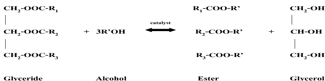
รูปที่ 2.1 ปฏิกิริยาทรานส์เอสเทอริฟิเคชันของไตรกลีเซอไรด์ กับแอลกอฮอล์
