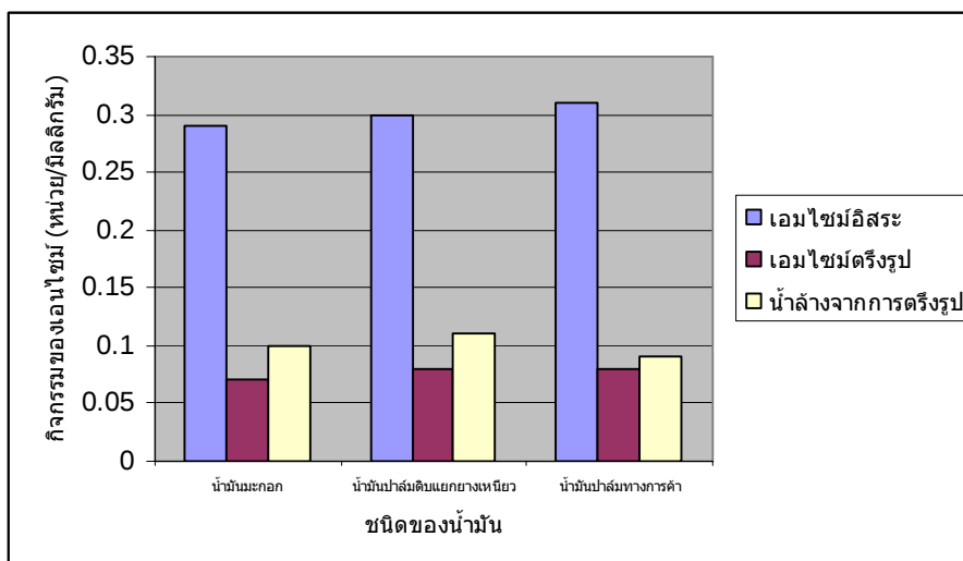
รูปที่ 3.1 กิจกรรมของเอนไซม์ไลเปสในสารตั้งต้นน้ำมันแต่ละชนิด
