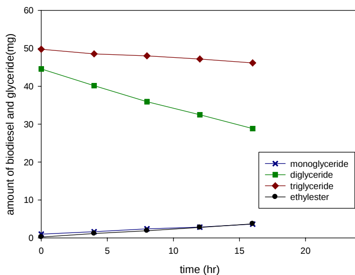
รูป 4.10 ปริมาณของไตรกลีเซอไรด์ ไดกลีเซอไรด์ โมโนกลีเซอไรด์ และเอธิลเอสเทอร์ระหว่างการทำปฏิกิริยา ทรานส์เอสเทอร์ฟิเคชันด้วยเอนไซม์ไลเปส
