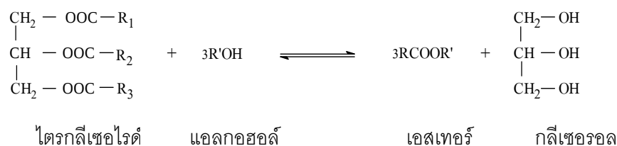
รูปที่ 4.1 ปฏิกริยาทรานส์เอสเทอริฟิเคชัน (Transesterification)
