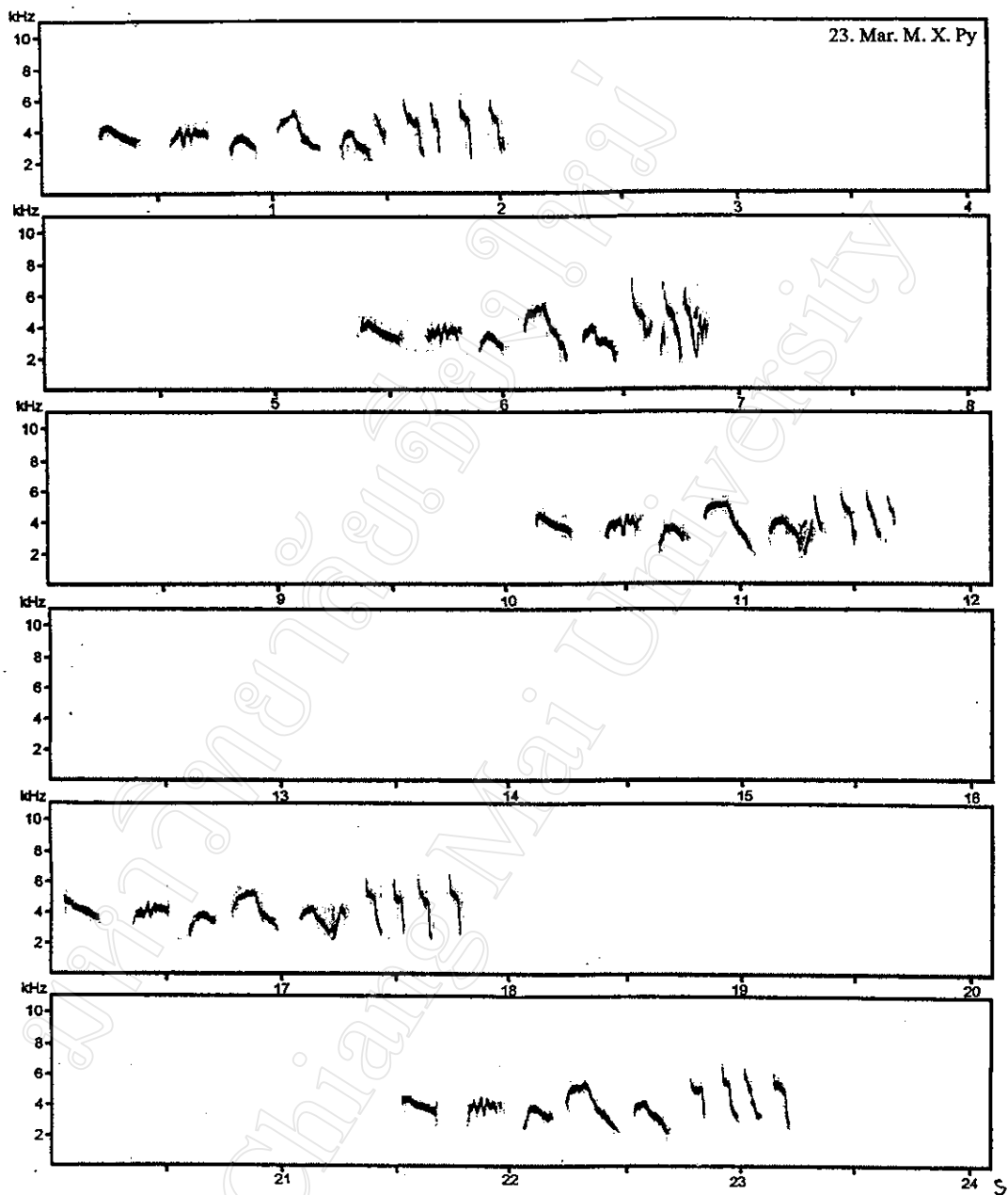
ภาพ 3 บทเพลงของนกนางแอ่นบ้านตัวที่ 23 ในจังหวัดพะเยา
