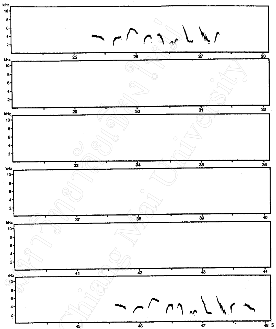
ภาพ 2 (ต่อ)
