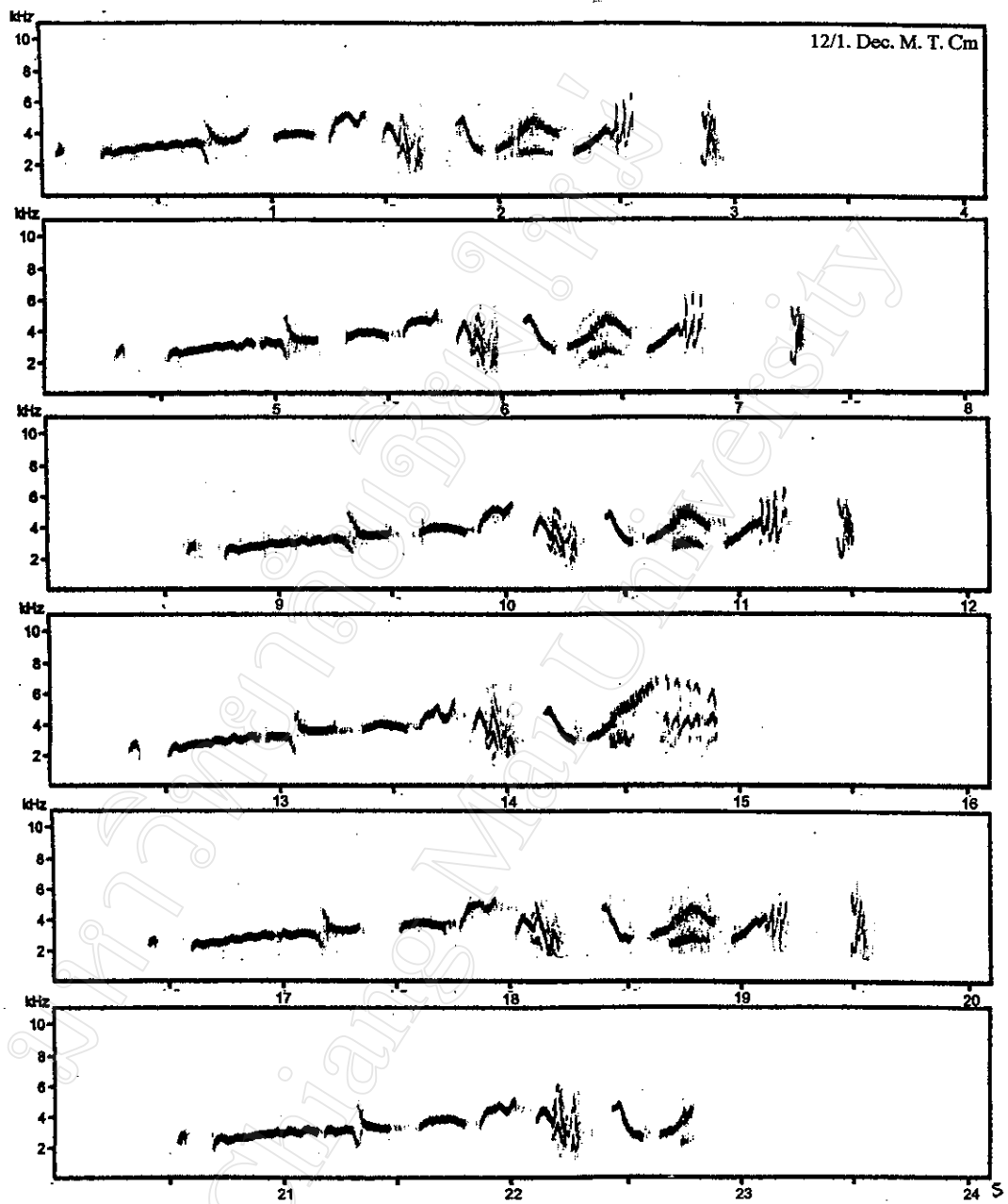
ภาพ 1 บทเพลงของนกนางแอ่นบ้านตัวที่ 12 ในจังหวัดเชียงใหม่ ก. บทเพลงที่ 1
