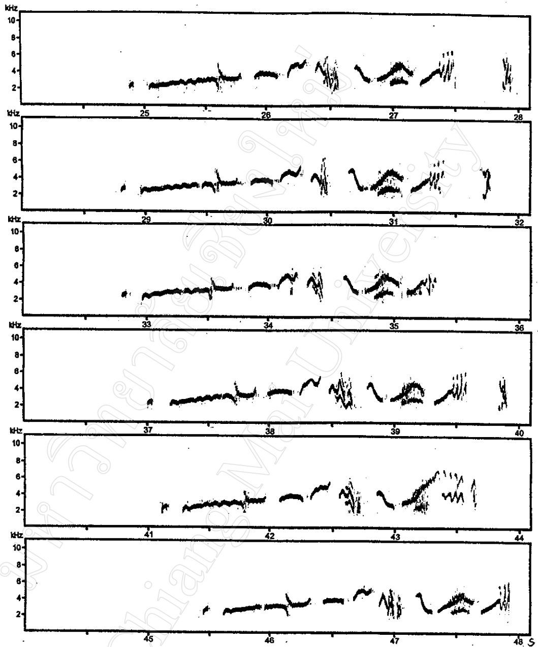
ก. (ต่อ) บทเพลงที่ 1
