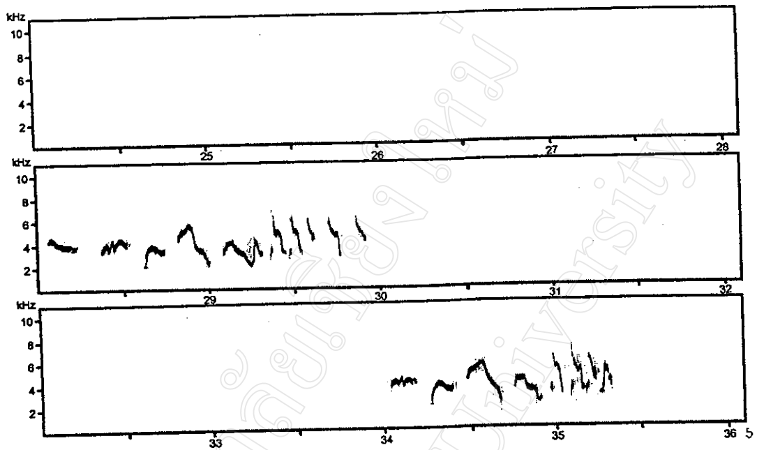
ภาพ 3 (ต่อ)
