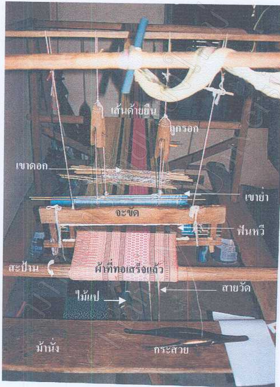
ภาพ 4.4 อุปกรณ์ต่างๆในการทอผ้ายกดอก
