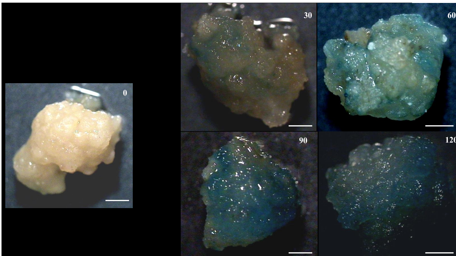
ภาพที่ 48 ผลการตรวจสอบการแสดงออกของยีน gus บนแคลลัสอ้อยพันธุ์ Phil 66-07 ที่บ่มร่วมกับ A. tumefaciens พันธุ์ LBA4404 (pCAMBIA 1305.1) ในระยะเวลา 0, 30, 60, 90 และ 120 นาที (สเกล = 1 มม.)
