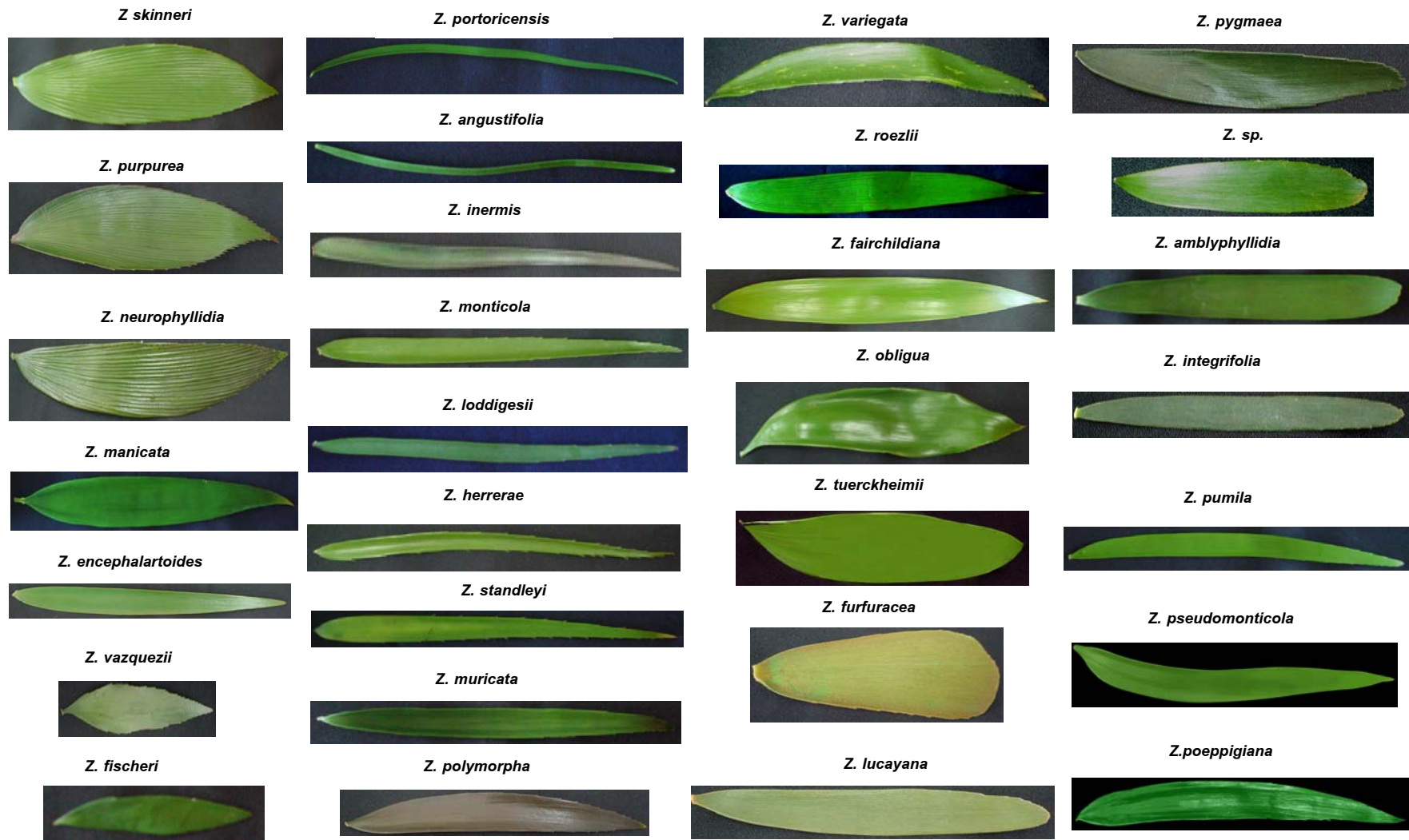
ภาพที่ 5 แสดงลักษณะทางสัณฐานวิทยาของใบย่อย โดยแสดงรูปร่าง สี และลักษณะของขอบใบย่อยของปรงในสกุล Zamia 30 ชนิด
