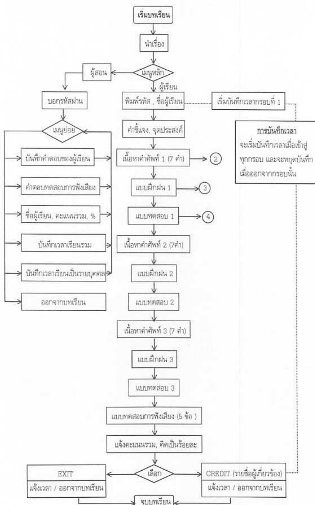
ภาพที่ 5 ผังงานรวมของบทเรียนคอมพิวเตอร์ช่วยสอนแบบมัลติมีเดีย เรื่องคำศัพท์
