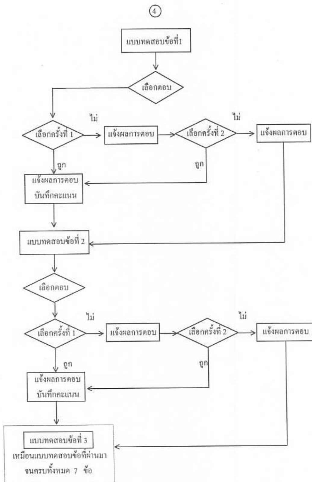
ภาพที่ 8 ผังงานแบบทดสอบของบทเรียนคอมพิวเตอร์ช่วยสอนแบบมัลติมีเดีย เรื่อง คำศัพท์
