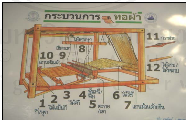
ภาพ 11 ขั้นตอนและวัสดุอุปกรณ์ในกระบวนการทอผ้า
