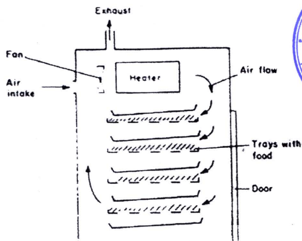
ภาพ 2.7 การทำงานของเครื่องอบแห้งลมร้อนแบบถาดทั่วไป
