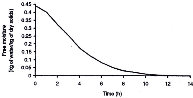
ภาพ 2.4 ปริมาณความชื้นที่เปลี่ยนแปลงตามเวลาการอบแห้ง
