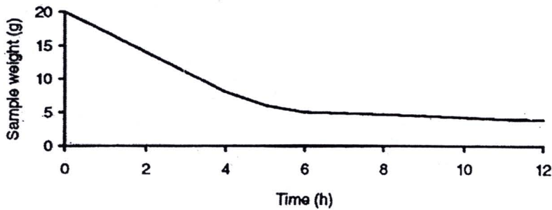
ภาพ 2.3 น้ำหนักที่เปลี่ยนแปลงระหว่างกระบวนการอบแห้ง
