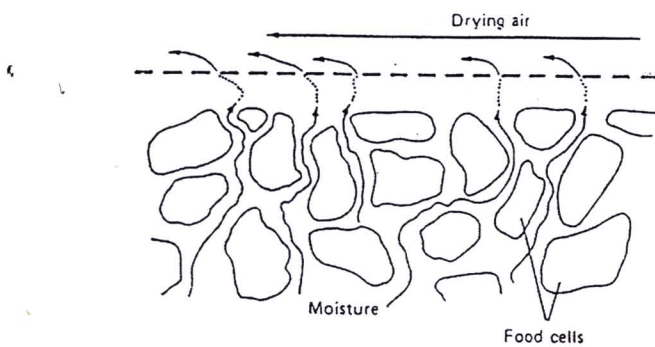
ภาพ 2.2 การเคลื่อนที่ของความชื้นออกจากชิ้นอาหารระหว่างการอบแห้ง ที่มา : Fellow (1990)
