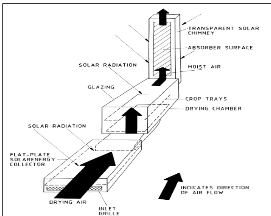
รูปที่ 2.5 เครื่องอบแห้งพลังงานแสงอาทิตย์แบบรับรังสีดวงอาทิตย์แบบผสม
