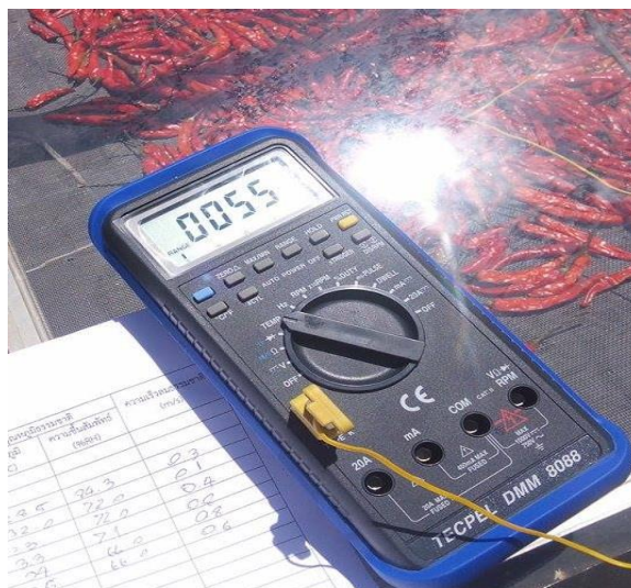
รูปที่ 3.11 การวัดอุณหภูมิภายในตู้อบแห้ง
