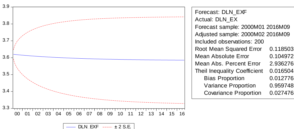
ภาพที่ 5 ผลการพยากรณ์อัตราแลกเปลี่ยนระหว่างบาทกับดอลลาร์สหรัฐด้วยแบบจำลอง
