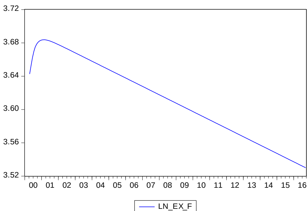
ภาพที่ 4 ผลการพยากรณ์อัตราแลกเปลี่ยนระหว่างบาทกับดอลลาร์สหรัฐในรูป ของลอการิทึมธรรมชาติ ตามแบบจำลอง VEC
